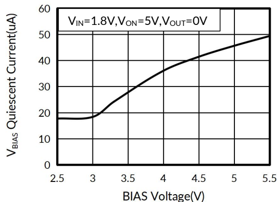
图 3. V_{\text{BIAS}} 静态电流与 BIAS 电压的关系
