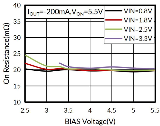
图 11. 导通电阻与偏置电压
