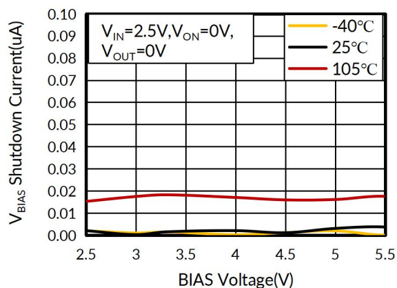
图 5. V_{\text{BIAS}} 关断电流与 BIAS 电压的关系
