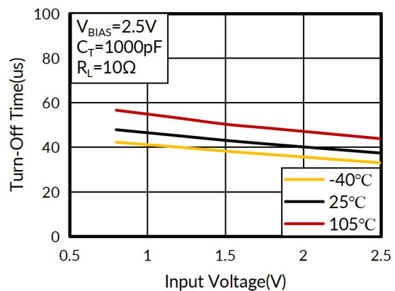
图 32. 关断时间与输入电压
