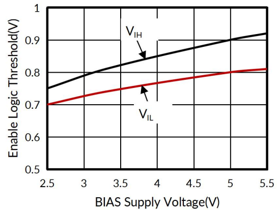
图 18. 启用逻辑阈值与 BIAS 电源电压
