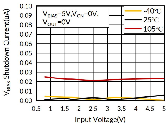
图 6. V_{\text{BIAS}} 关断电流与输入电压的关系
