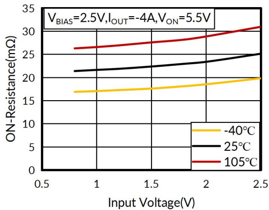
图 13. 导通电阻与输入电压的关系
