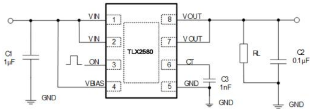
图 1.测试电路
