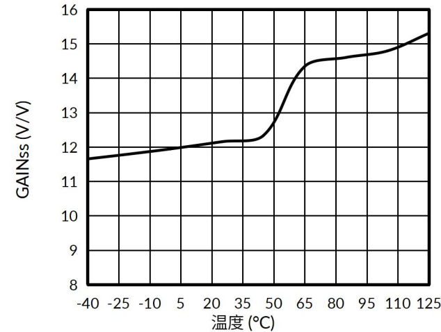
图 11. GAIN ss 与温度的关系
