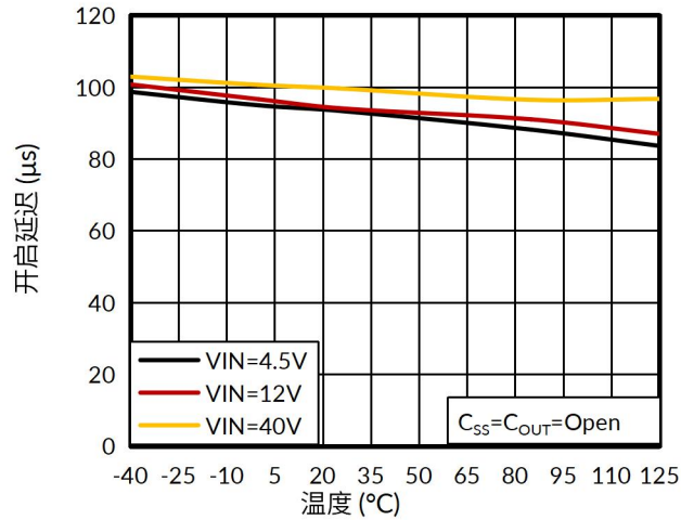
图 1. 开启延迟 t_{ON\_DLY} 与温度的关系
