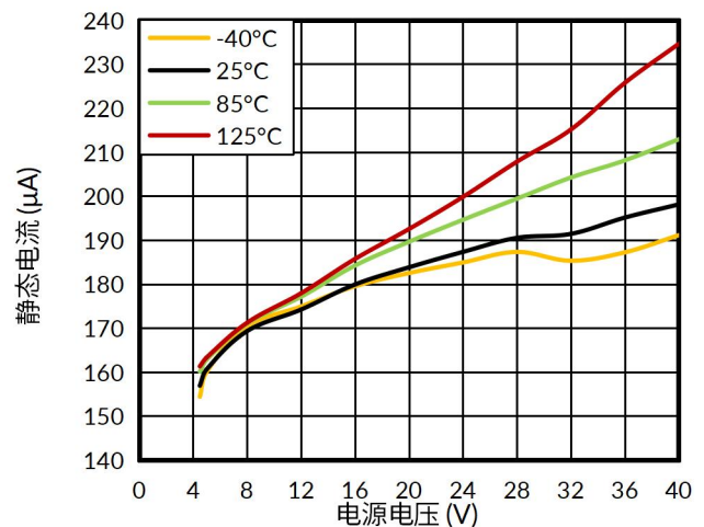
图 6. 静态电流与电源电压的关系
