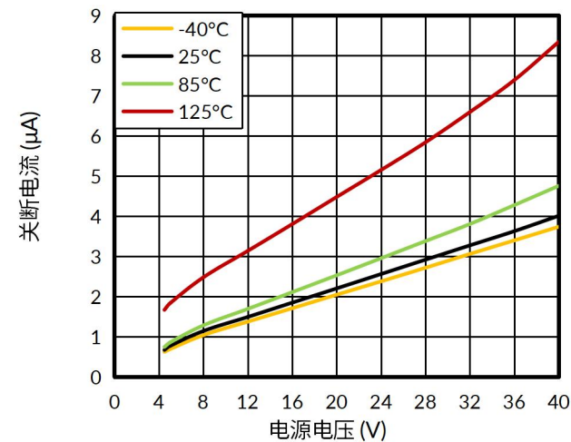
图 7. 关断电流与电源电压的关系
