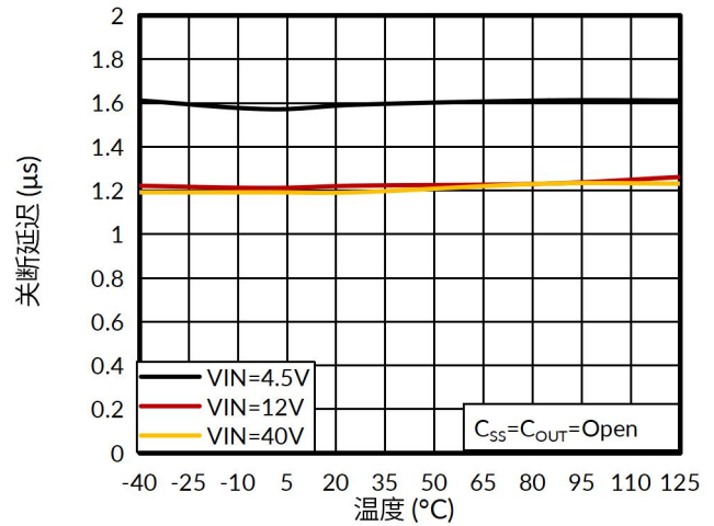
图 2. 关断延迟 t_{OFF\_DLY} 与温度的关系
