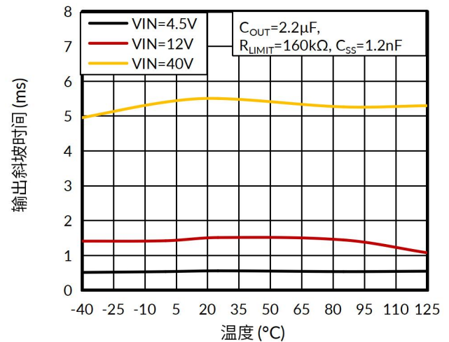
图 4. 输出斜坡时间 t_{RISE} 与温度的关系
