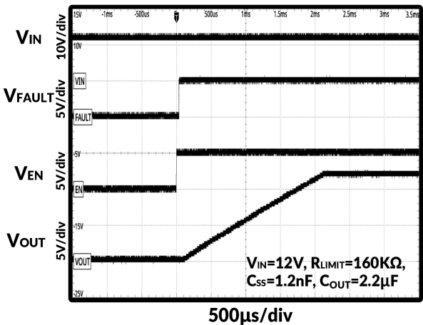
图 16. 使能启动
