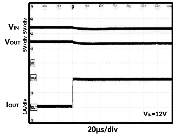
图 21. 输出过流
