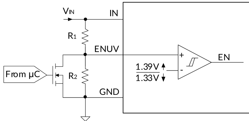
图 27. 关断控制
