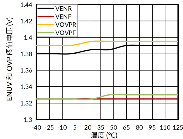
图 9. ENUV 和 OVP 阈值电压与温度的关系
