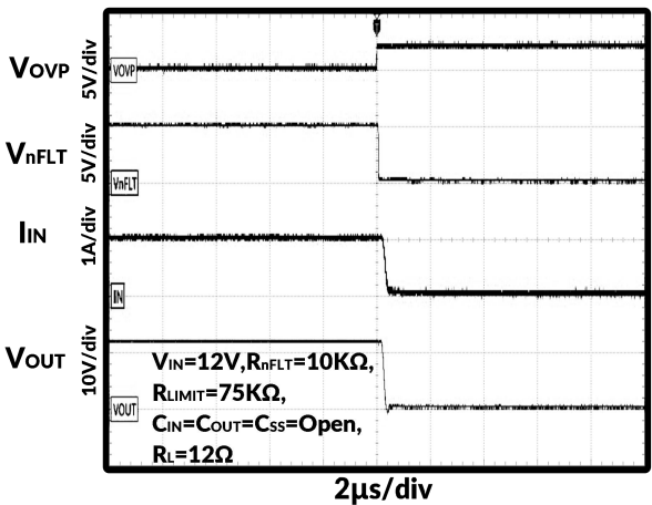
图 18. OVP 关断延迟: OVP↑ 至 Fault↓
