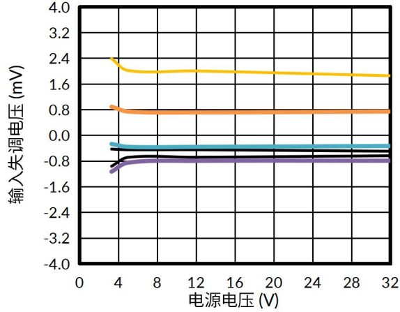
图 15. 输入失调电压与电源电压的关系, 25°C
