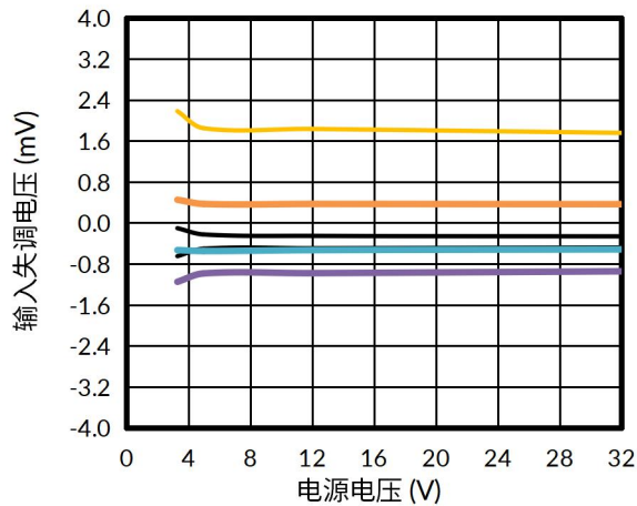
图 17. 输入失调电压与电源电压的关系, 125°C
