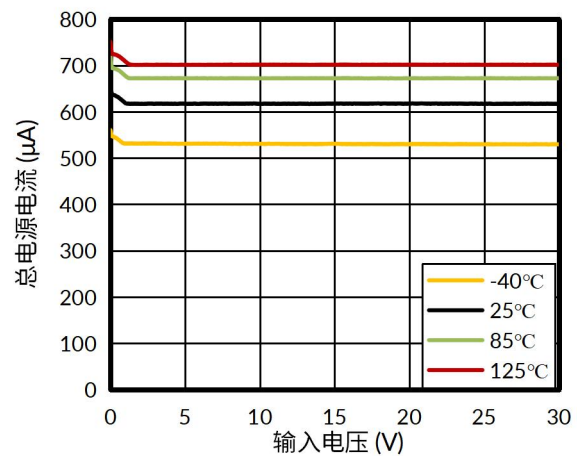
图 10. 总电源电流与输入电压的关系，32V
