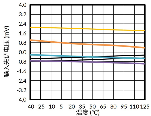
图 12. 输入失调电压与温度的关系，12V
