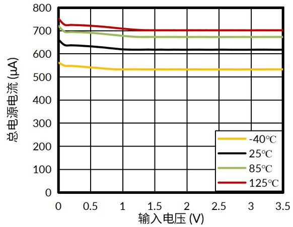
图 8. 总电源电流与输入电压的关系，5V
