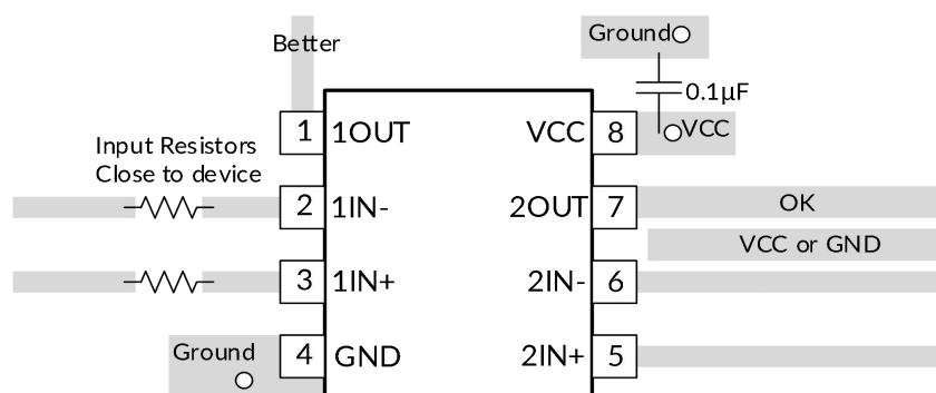
图 9. TLX2903 PCB 布局示例
