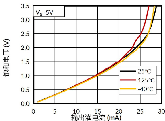
图 5. 饱和电压和输出灌电流的关系
