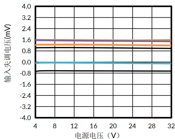
图 16. 85^{\circ}\text{C} 时输入失调电压与电源电压的关系
