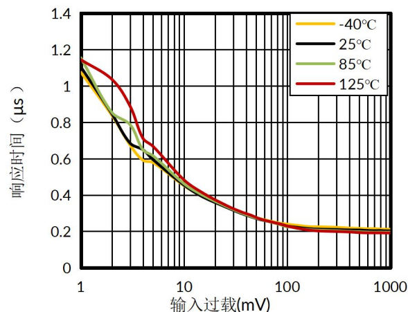
图 1. 响应时间与输入过驱动负转换，5V
