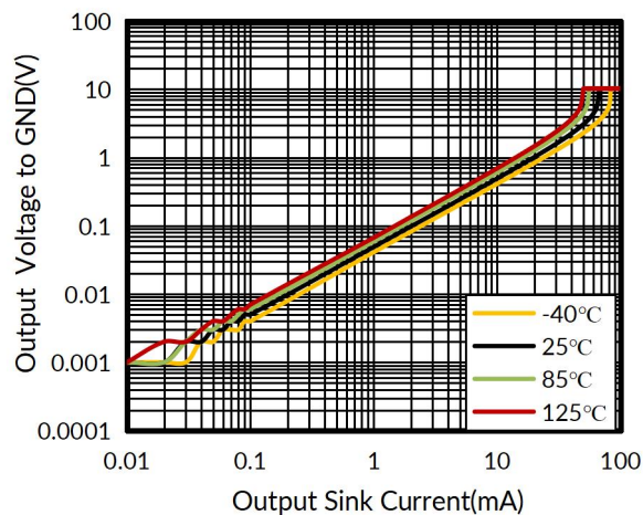
图 19. 12V 时输出低电压与输出灌电流的关系
