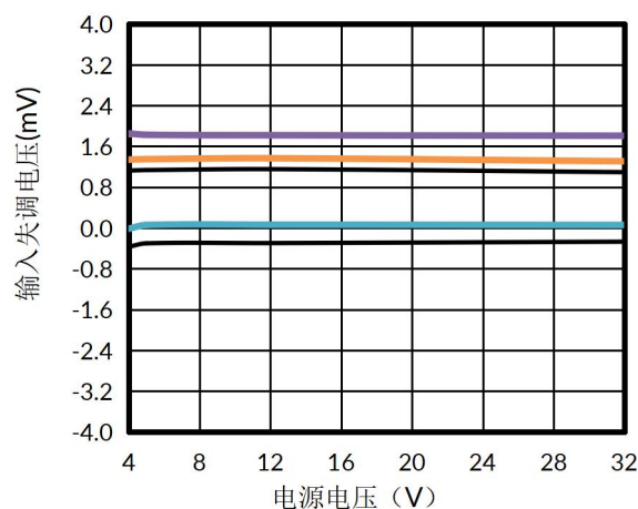
图 14. -40^{\circ}\text{C} 时输入失调电压与电源电压的关系
