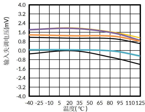
图 12. 12V 时输入失调电压与温度的关系
