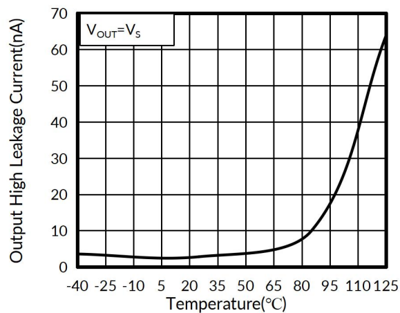
图 21. 5V 时输出高漏电流与温度的关系
