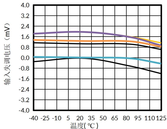
图 11. 5V 时输入失调电压与温度的关系
