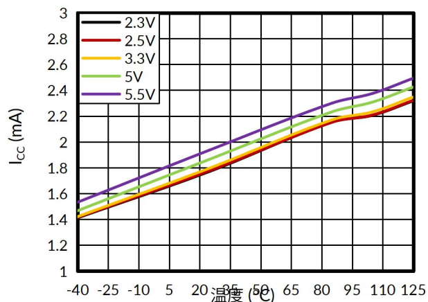
图 1. I_{CC} 与温度的关系
