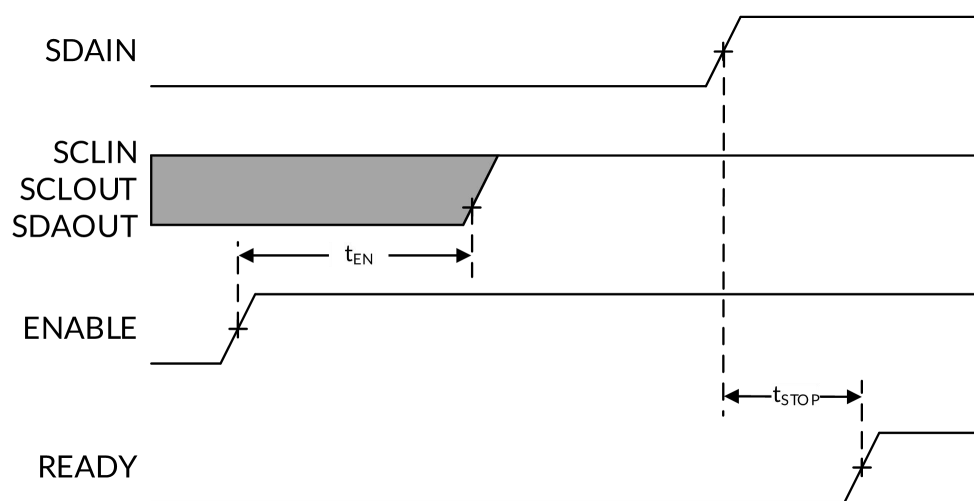
图 7. t_{STOP} 时序
