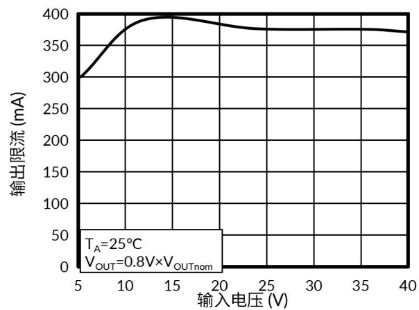
图 16. 输出限流与输入电压的关系
