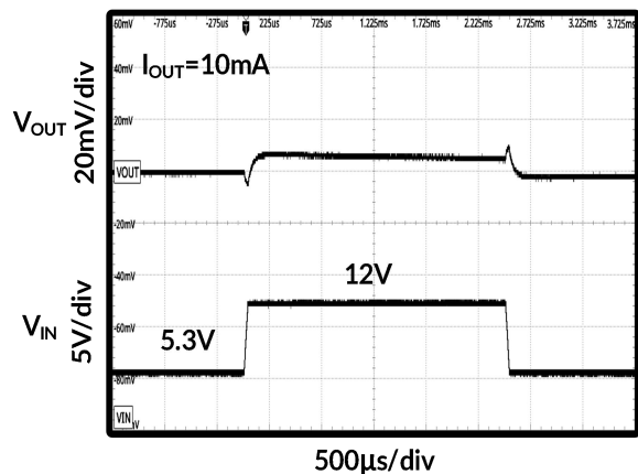
图 29. 线性瞬态响应
