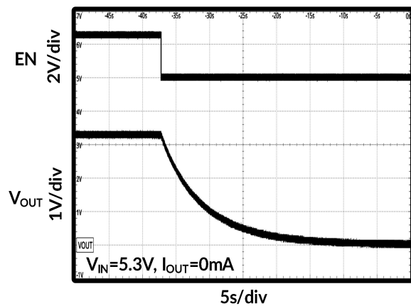
图 22. 关断时序
