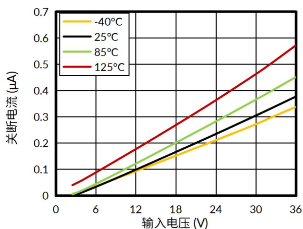
图 3. 关断电流与输入电压的关系
