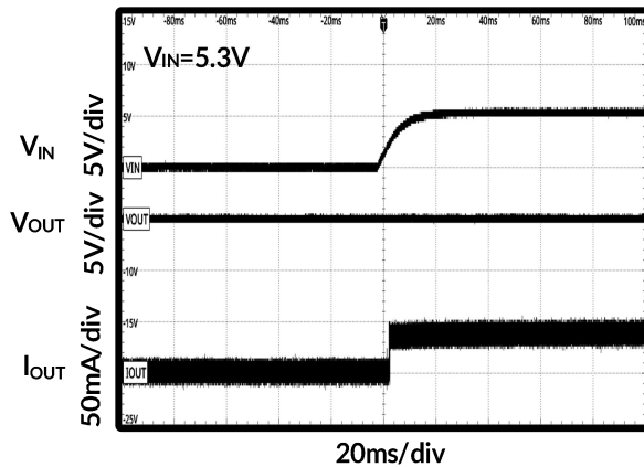
图 26. 先短路后 VIN 开启时序图
