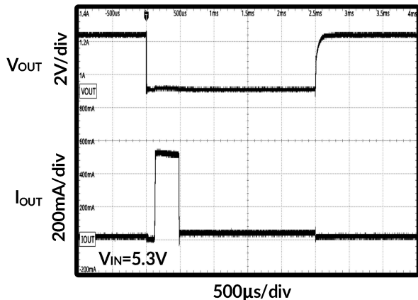
图 25. 先开启后短路时序图
