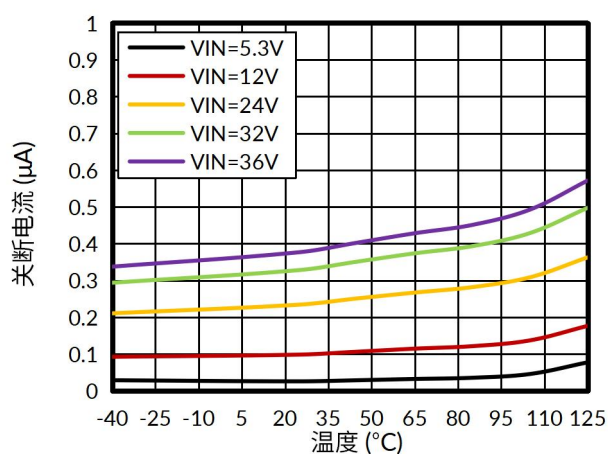
图 4. 关断电流与温度的关系
