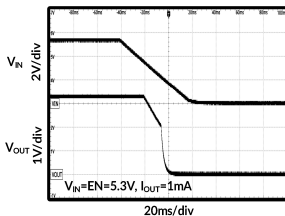
图 18. 下电时序
