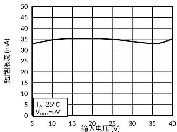
图 15. 短路限流与输入电压的关系
