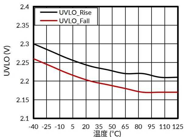
图 12. UVLO 与温度的关系
