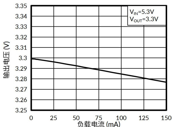
图 7. 负载调整率
