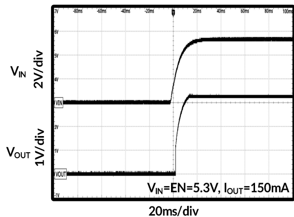
图 19. 上电时序
