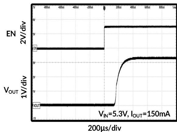
图 23. 开启时序
