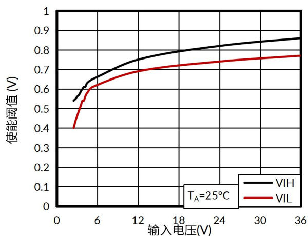
图 13. 使能阈值与输入电压的关系
