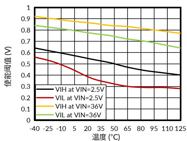
图 14. 使能阈值与温度的关系
