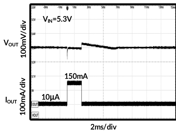
图 31. 负载瞬态响应
