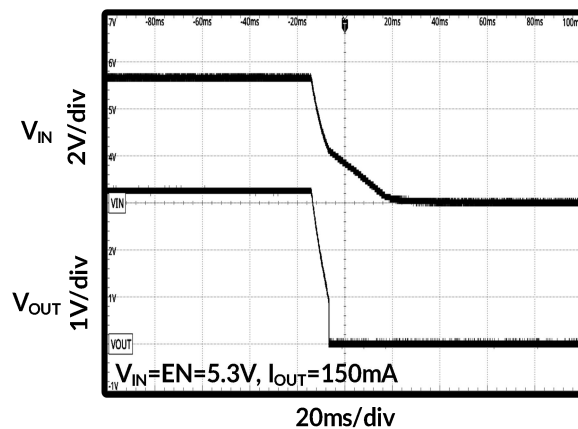
图 20. 下电时序
