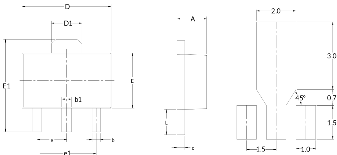
推荐焊盘尺寸 (单位: 毫米)
