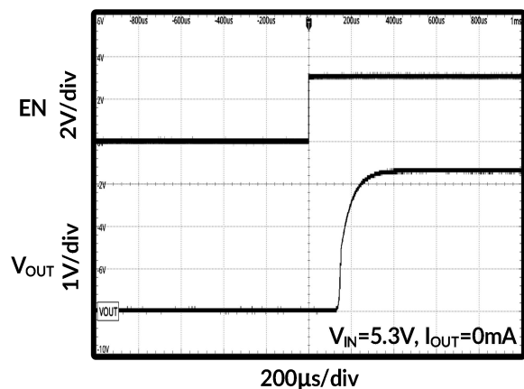
图 21. 开启时序
