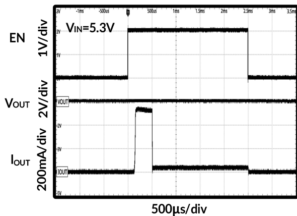
图 27. 先短路后 EN 开启时序图
