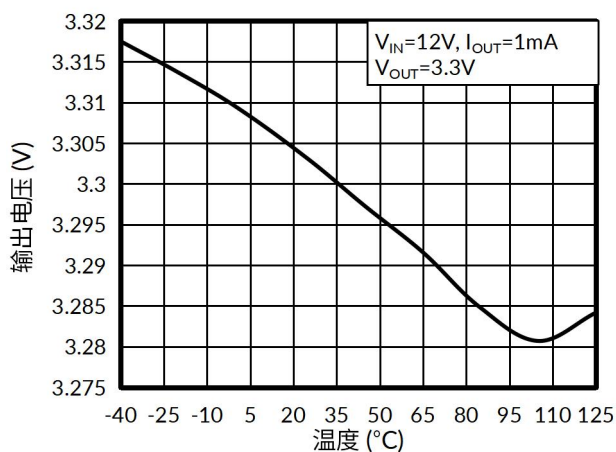
图 9. 输出电压与温度的关系
