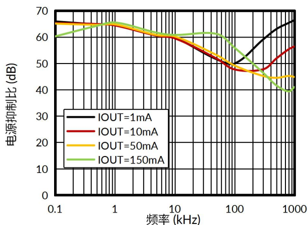
图 11. 电源抑制比与频率的关系
