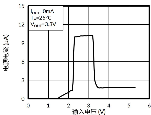
图 5. 电源电流与输入电压的关系
