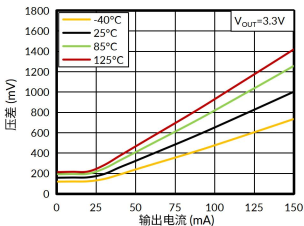
图 10. 压差与输出电流的关系
