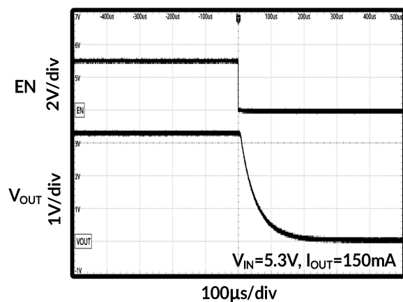
图 24. 关断时序
