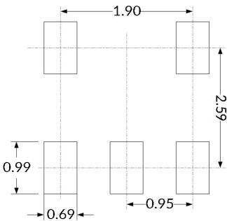
推荐焊盘尺寸 (单位: 毫米)
