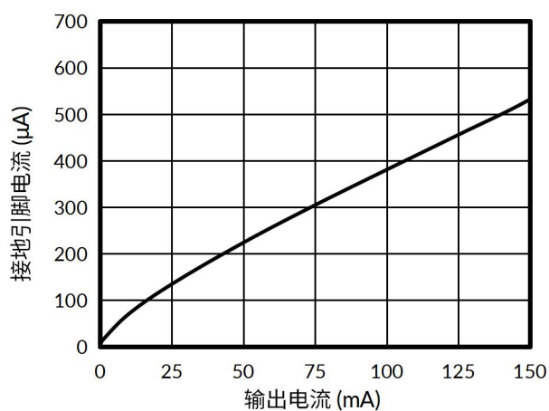
图 6. 接地引脚电流与输出电流的关系
