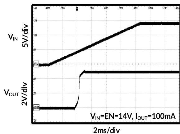
图 21. 上电时序
