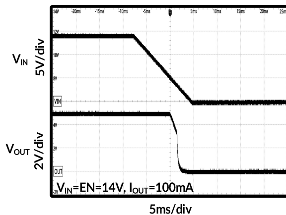
图 22. 下电时序
