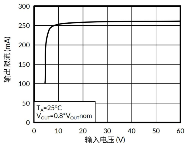
图 17. 输出限流与输入电压的关系
