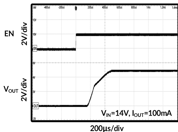
图 25. 开启时序
