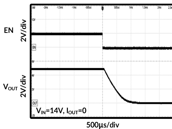
图 24. 关断时序
