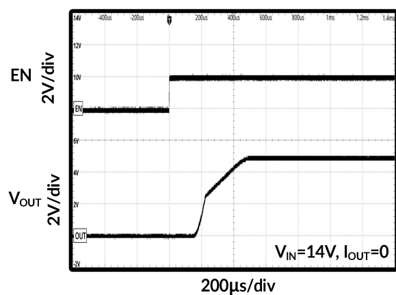
图 23. 开启时序
