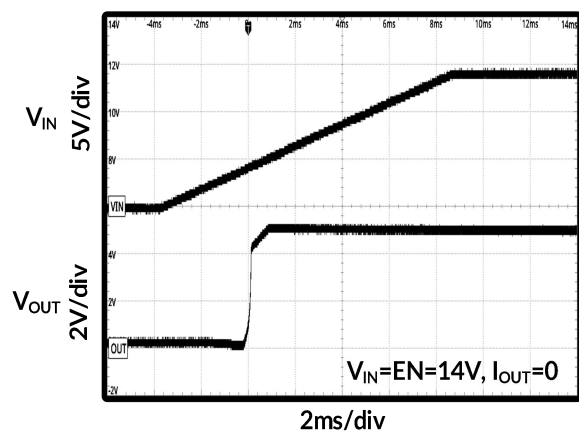
图 19. 上电时序
