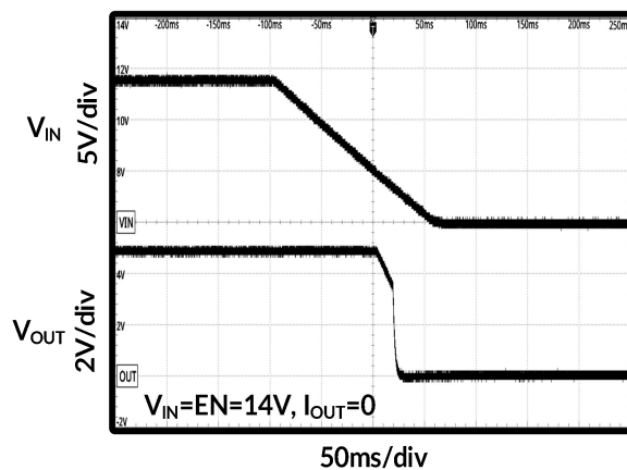
图 20. 下电时序
