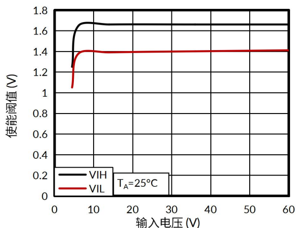
图 13. 使能阈值与输入电压的关系
