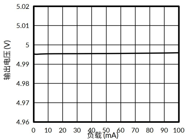
图 7. 负载调整率
