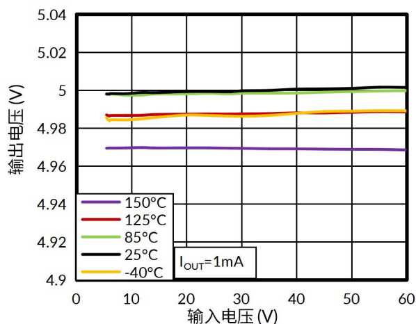
图 8. 线性调整率
