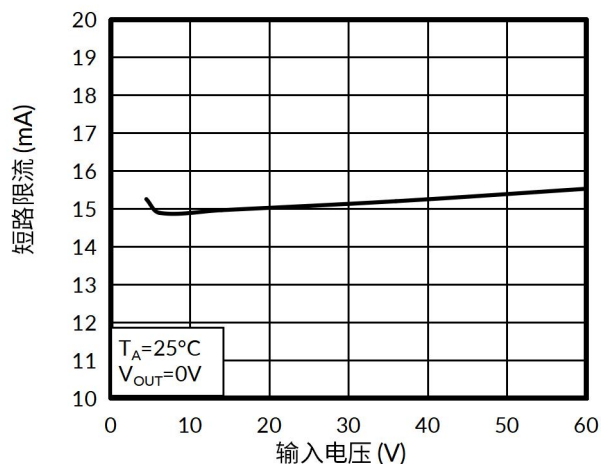
图 15. 短路限流与输入电压的关系
