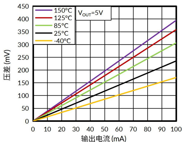
图 10. 压差与输出电流的关系
