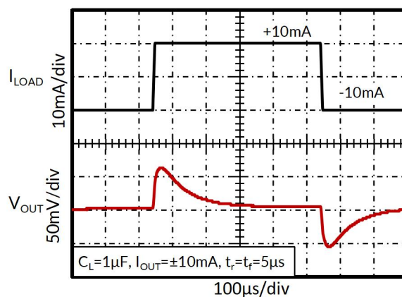
图 16. 负载瞬态
