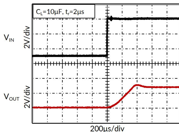
图 14. 启动
