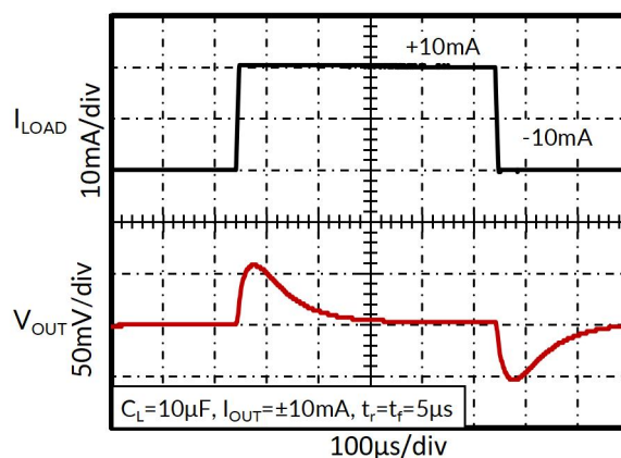
图 18. 负载瞬态
