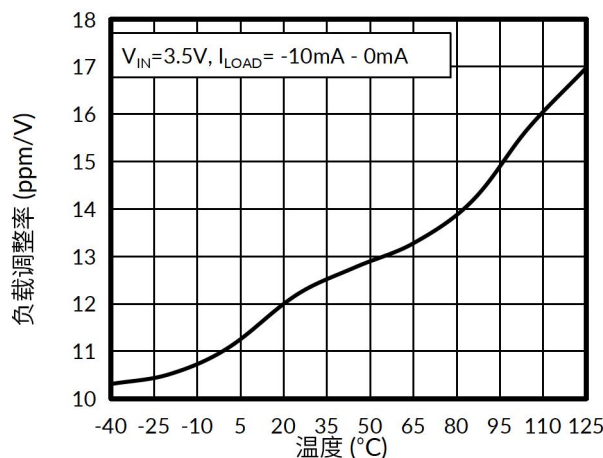
图 11. 负载调整率与温度的关系
