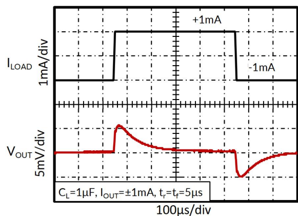
图 15. 负载瞬态
