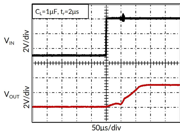
图 13. 启动
