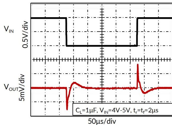
图 19. 线性瞬态响应
