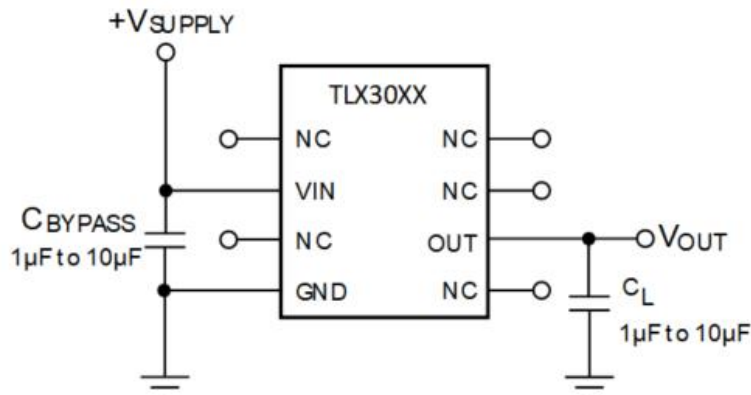
图 21. 基本连接
