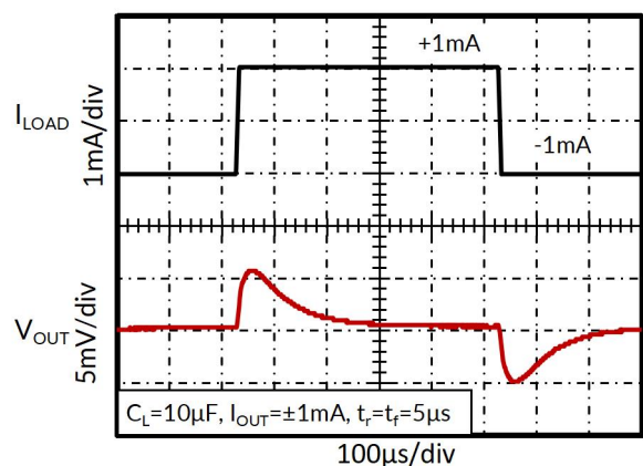
图 17. 负载瞬态
