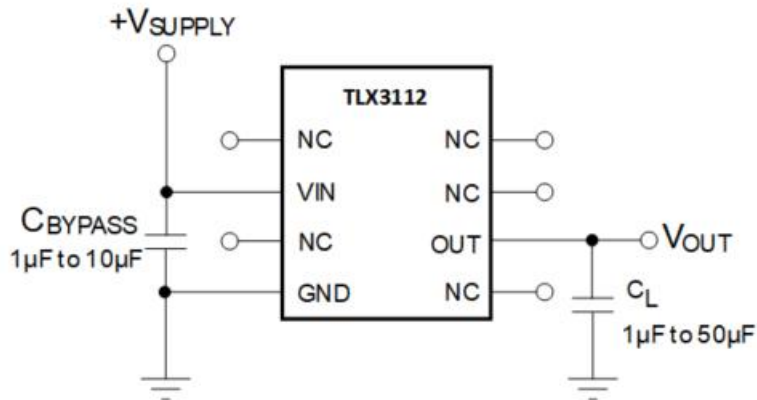
图 16. 基本连接
