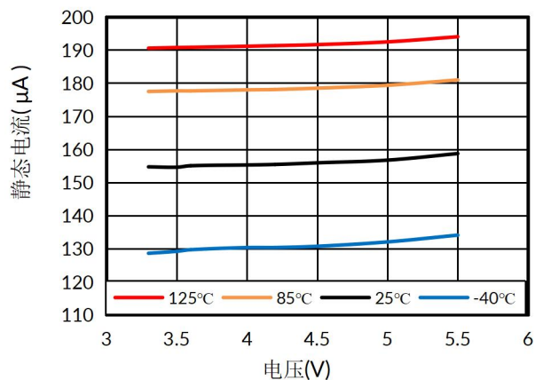
图 5. 静态电流与电源电压
