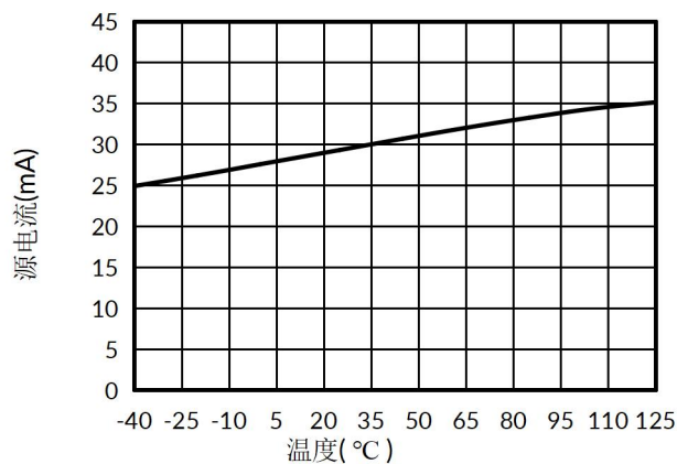
图 7. 源电流与温度
