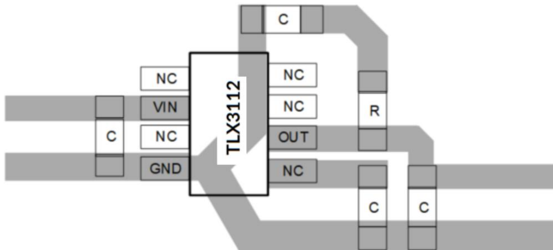
图 18. 布局示例
