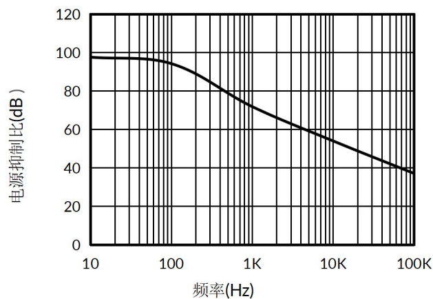
图 8. PSRR 与频率
