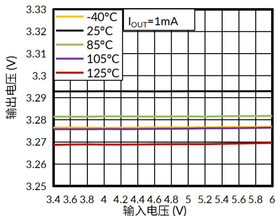
图 7. 线性调整率
