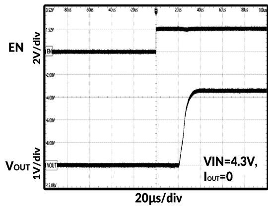
图 18. 开启时序
