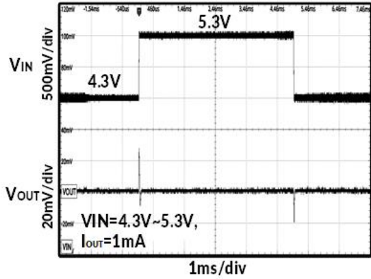
图 22. 线性瞬态响应 ( I_{OUT}=1mA )
