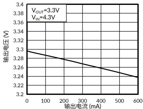
图 6. 负载调整率
