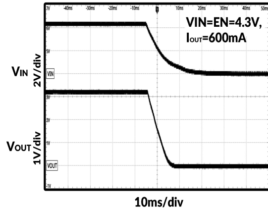
图 17. 下电时序
