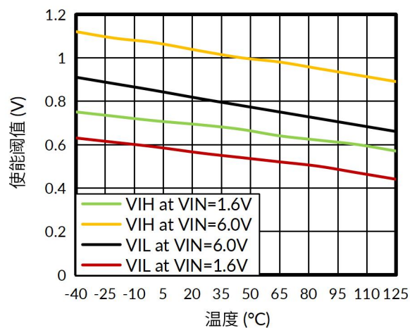
图 11. 使能阈值与结温的关系
