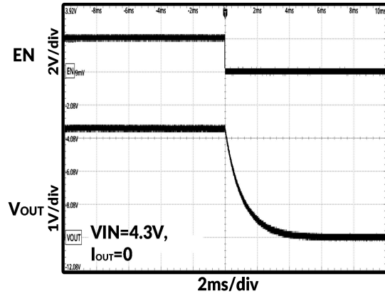
图 19. 关断时序
