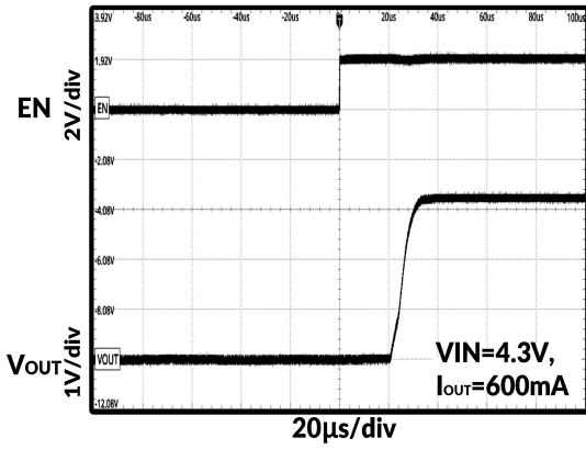
图 20. 开启时序
