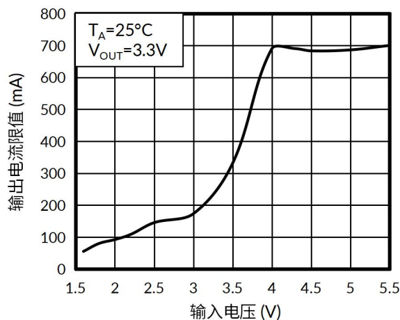
图 12. 输出电流限值与输入电压的关系
