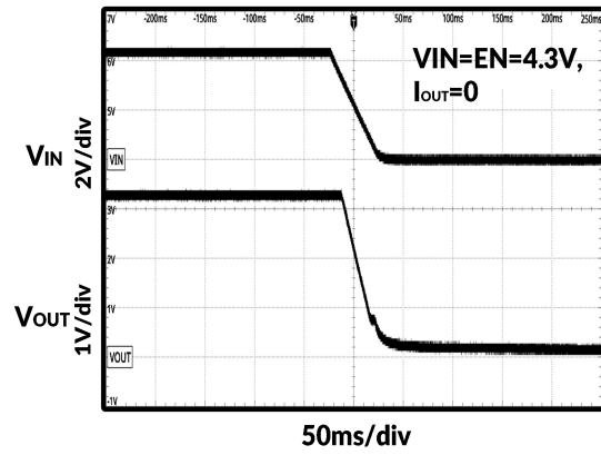
图 15. 下电时序
