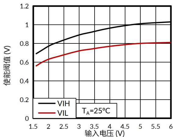
图 10. 使能阈值与输入电压的关系
