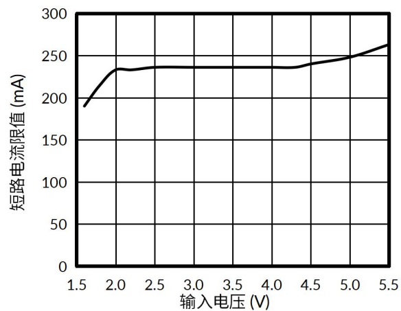
图 13. 短路电流限值与输入电压的关系
