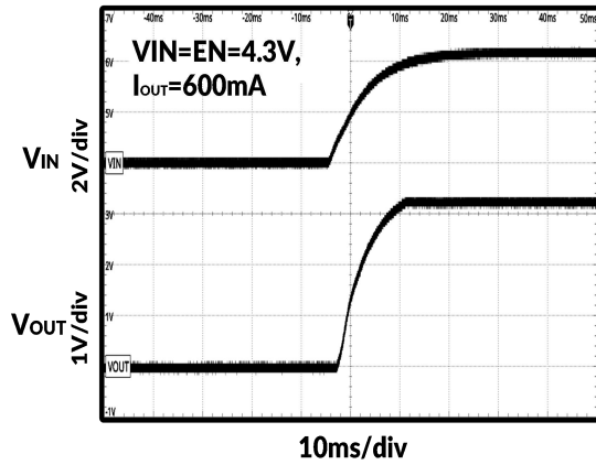
图 16. 上电时序
