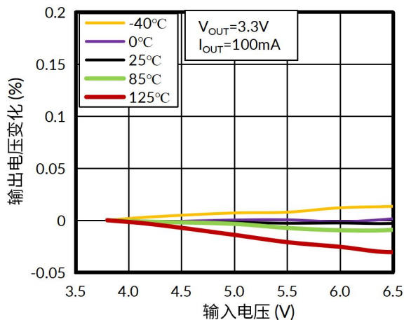
图 10. 线性调整率
