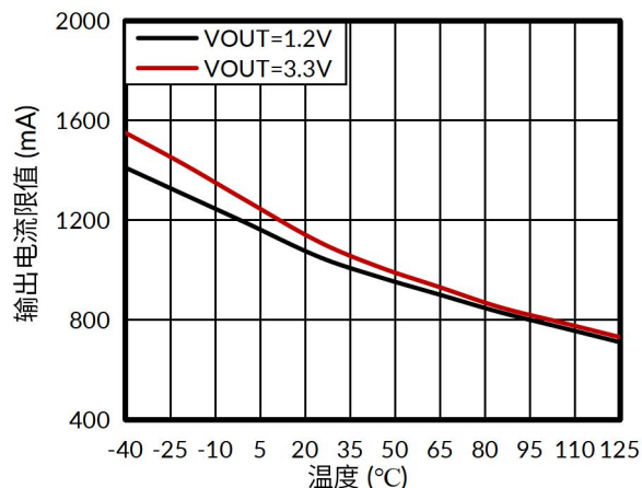
图 21. 输出电流限值与温度的关系
