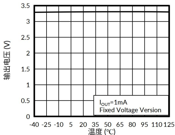
图 11. 输出电压与结温的关系
