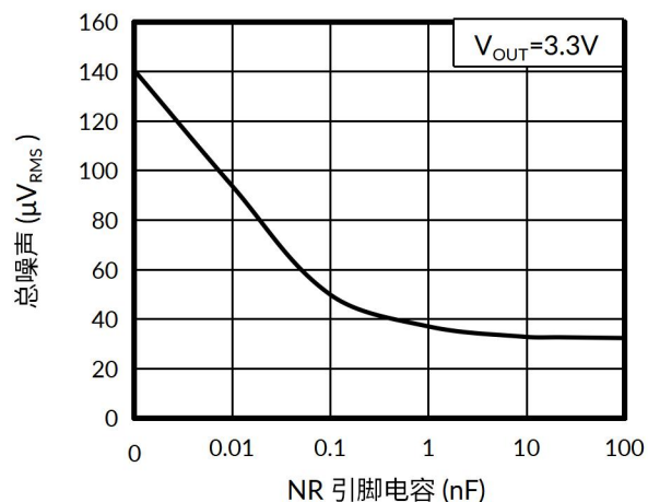
图 20. RMS 噪声与 CNR 的关系
