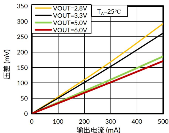
图 17. 压差与输出电流的关系
