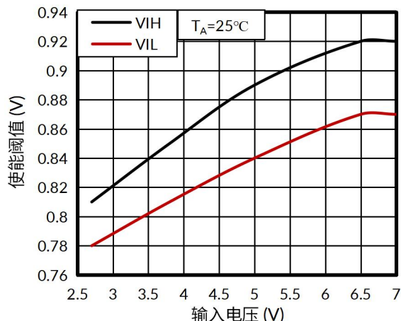
图 15. 使能阈值与输入电压的关系
