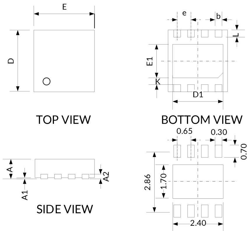
推荐焊盘尺寸 (单位: 毫米)
