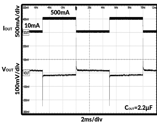
图 23. 负载瞬态响应
