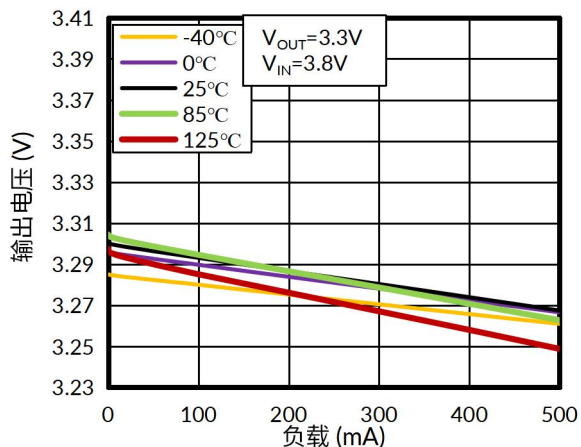
图 8. 负载调整率
