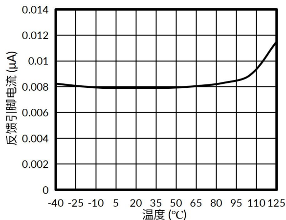
图 13. 反馈引脚电流与结温的关系
