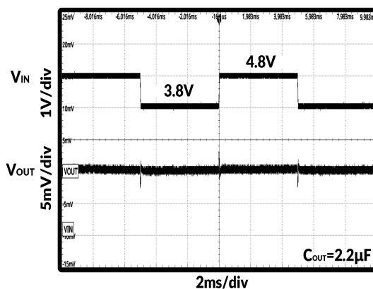
图 22. 线性瞬态响应
