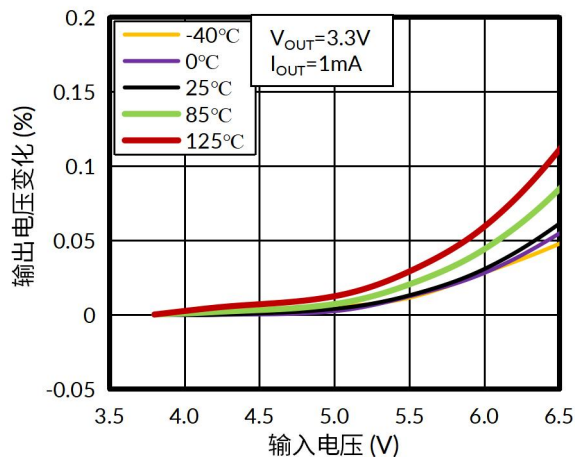
图 9. 线性调整率
