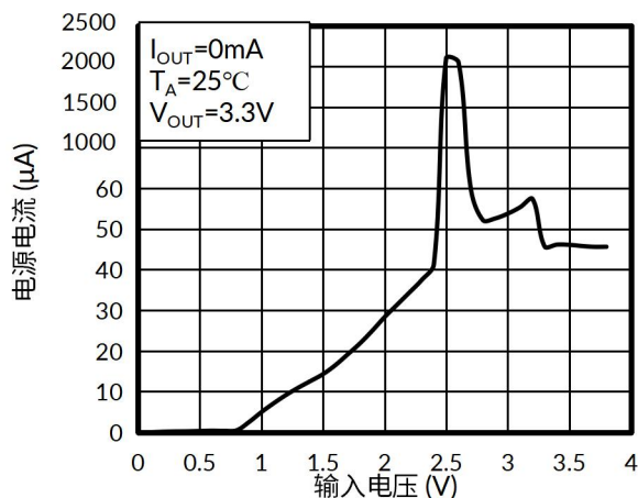
图 6. 电源电流与输入电压的关系
