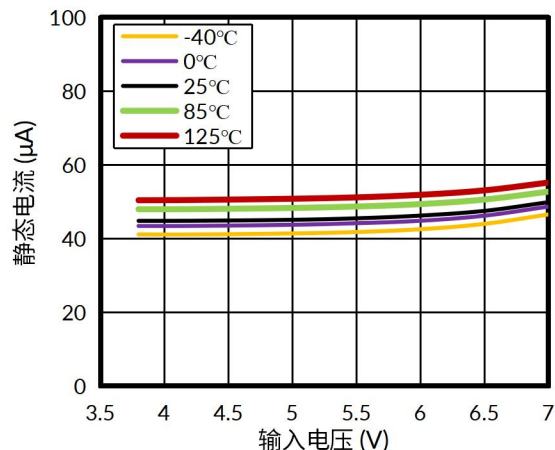
图 3. 静态电流与输入电压的关系
