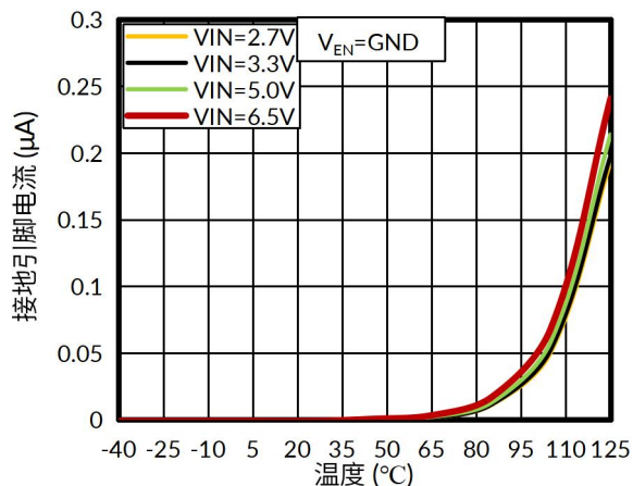
图 7. 关断电流与温度的关系
