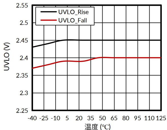
图 14. UVLO 与结温的关系
