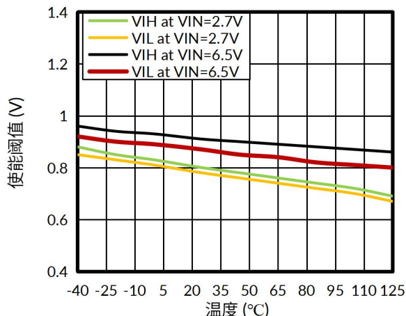
图 16. 使能阈值与结温的关系
