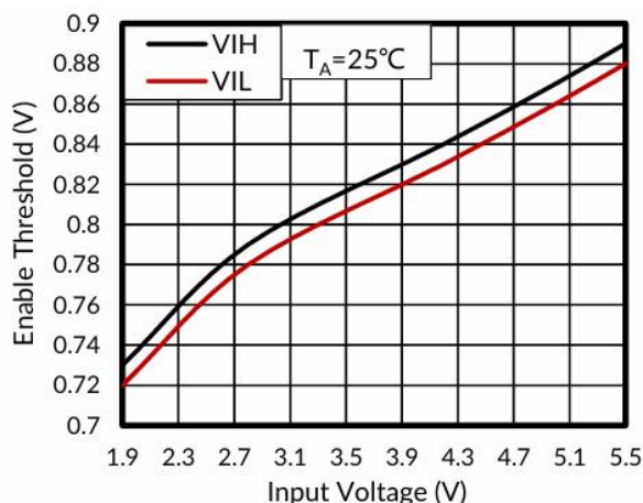
图 12. 使能阈值与输入电压
