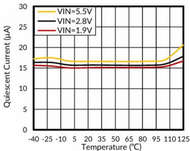
图 2. 静态电流与结温的关系
