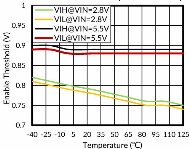
图 13. 使能阈值与结温
