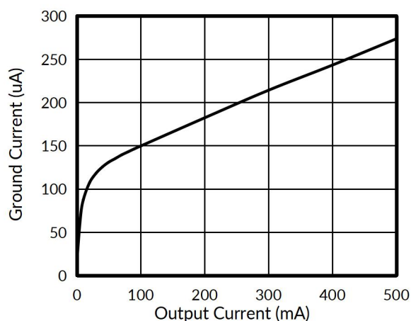
图 5. 地电流与输出电流
