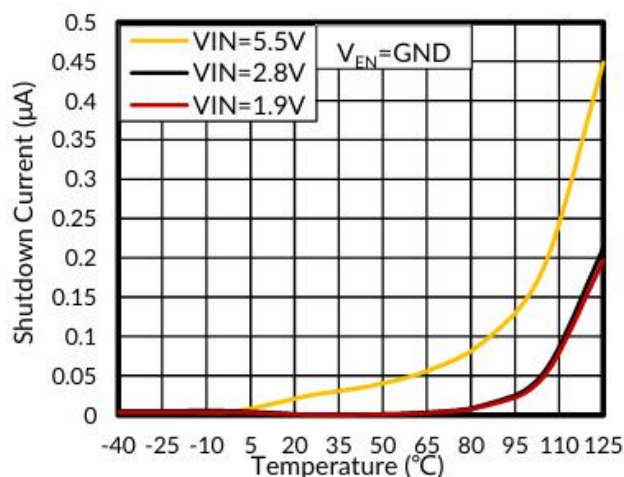
图 3. 关断电流与结温的关系
