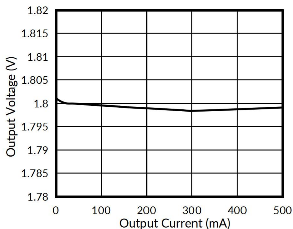
图 6. 负载调节
