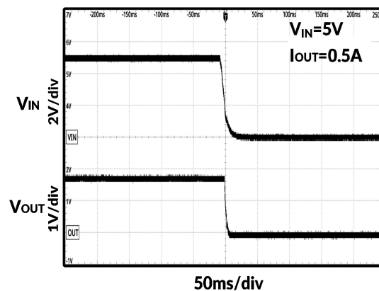
图 17. 下电时序
