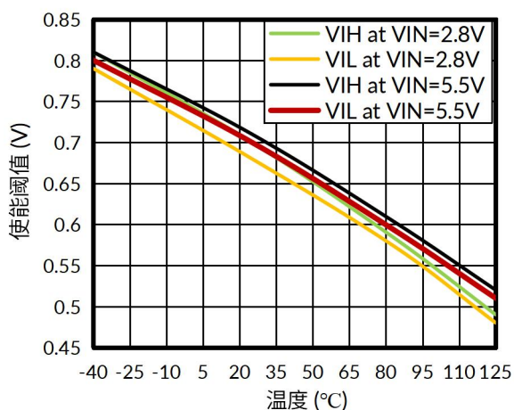
图 12. 使能阈值与结温的关系
