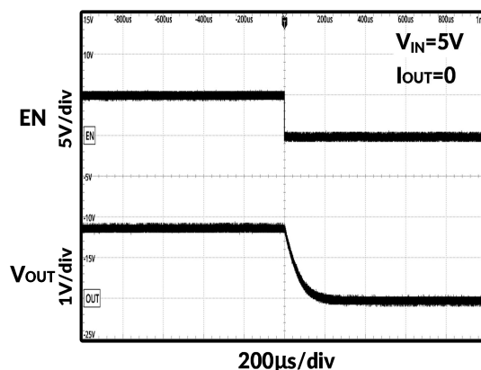
图 19. 关断时序
