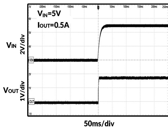
图 16. 上电时序
