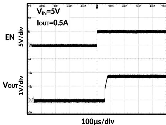
图 20. 开启时序
