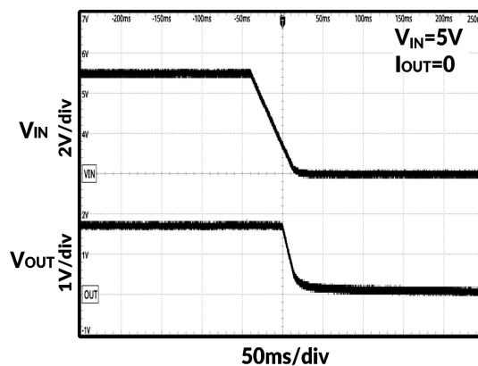
图 15. 下电时序
