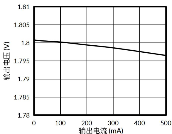
图 6. 负载调整率
