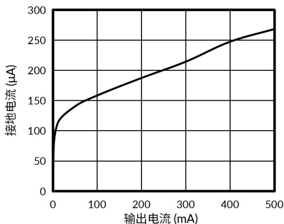
图 5. 接地电流与输出电流的关系
