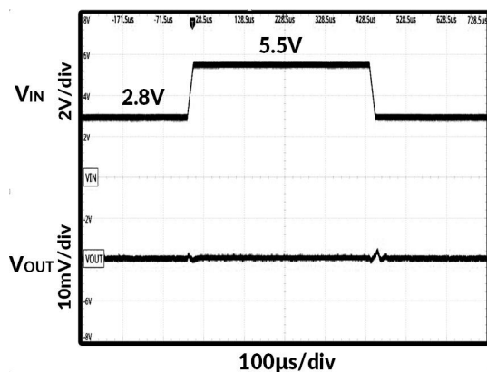
图 24. 线性瞬态响应 ( I_{OUT}=1mA )
