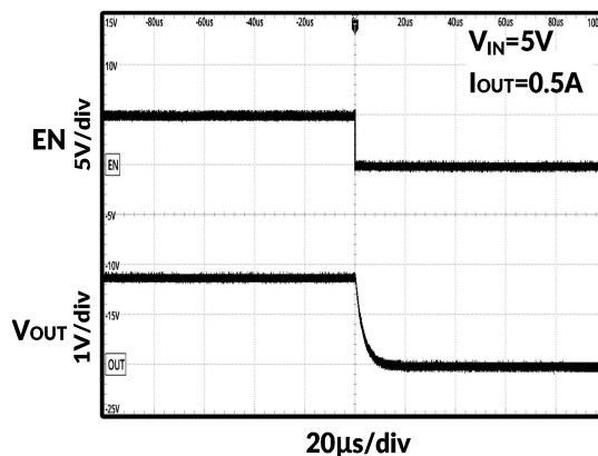
图 21. 关断时序
