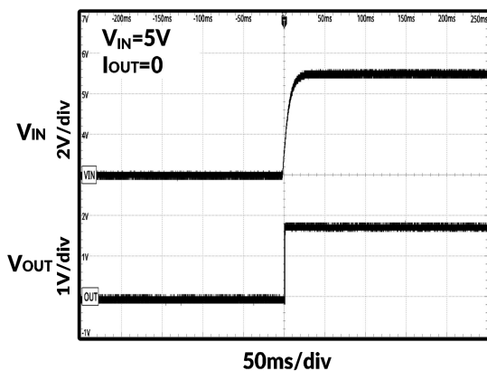
图 14. 上电时序
