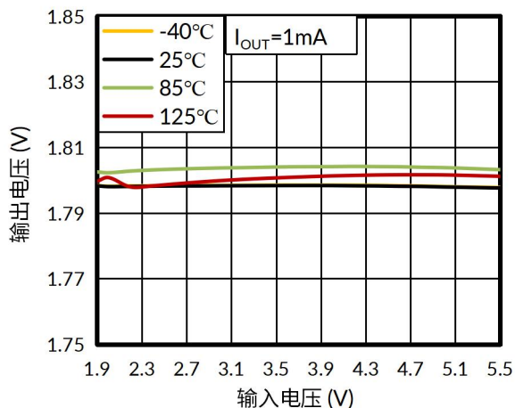
图 7. 线性调整率
