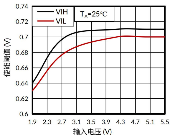
图 11. 使能阈值与输入电压的关系
