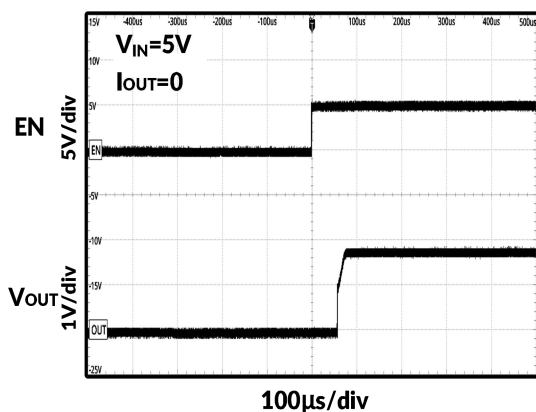
图 18. 开启时序
