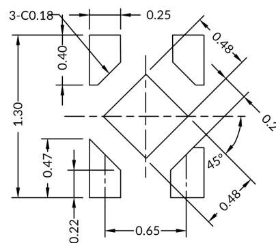
推荐焊盘尺寸 (单位: 毫米)
