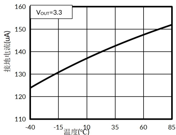
图 7. 接地电流与温度
