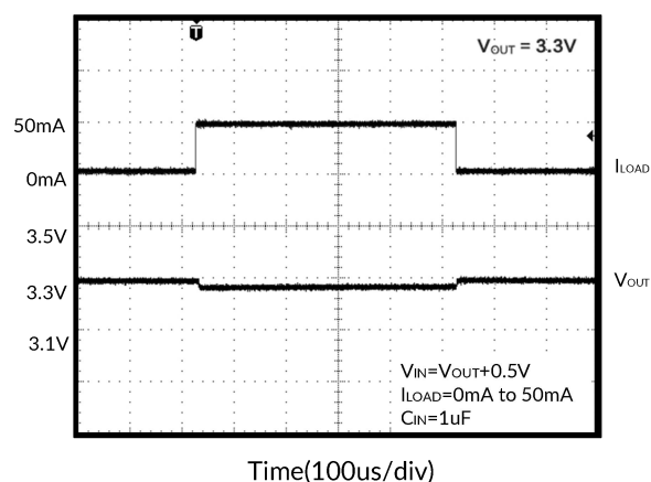
图 4. 负载瞬态响应
