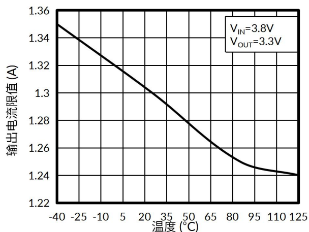
图 17. 输出电流限值与温度的关系
