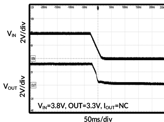
图 19. 下电时序
