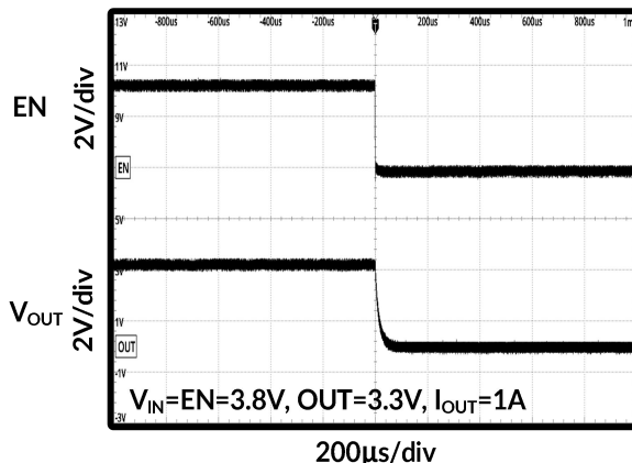
图 25. EN 关断时序
