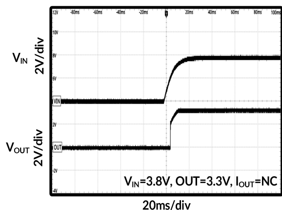
图 18. 上电时序
