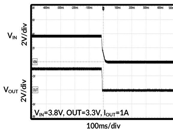
图 21. 下电时序
