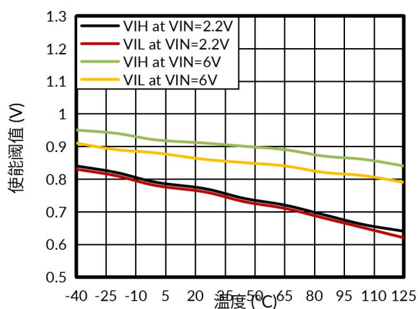
图 12. 使能阈值与结温的关系
