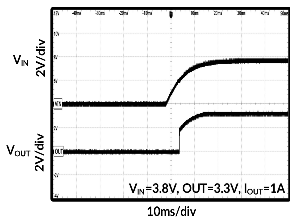
图 20. 上电时序
