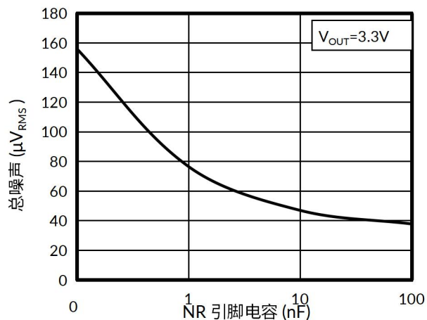
图 16. RMS 噪声与 C_{NR} 的关系
