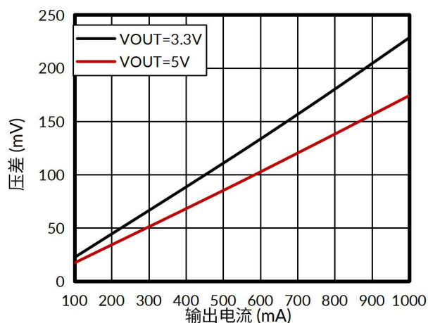
图 13. 压差与输出电流的关系
