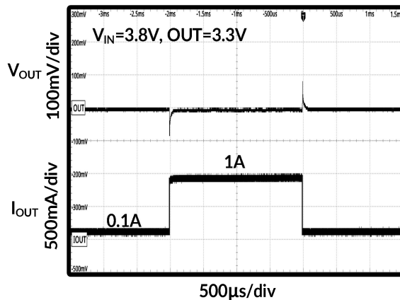
图 29. 负载瞬态响应
