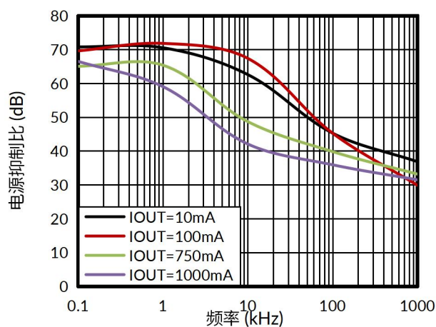
图 15. 电源抑制比与频率的关系
