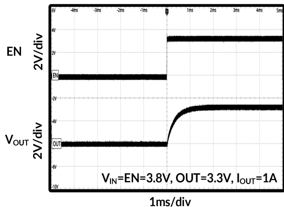
图 24. EN 开启时序
