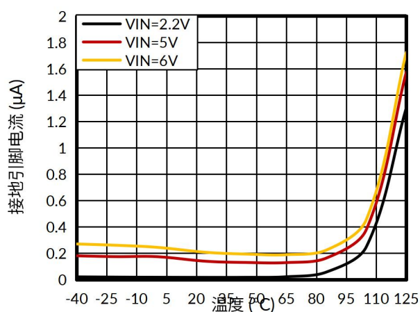
图 5. 关断电流与温度的关系
