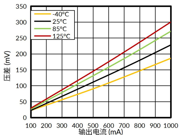
图 14. 压差与输出电流的关系
