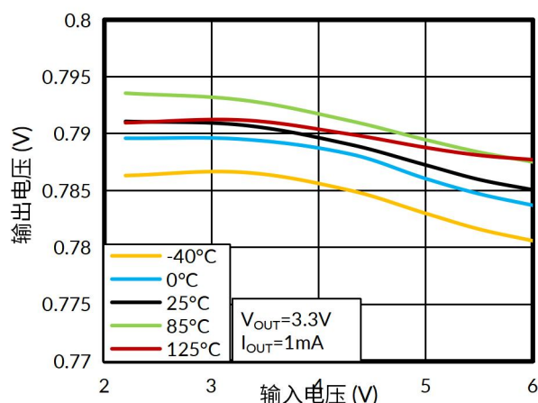
图 7. 线性调整率
