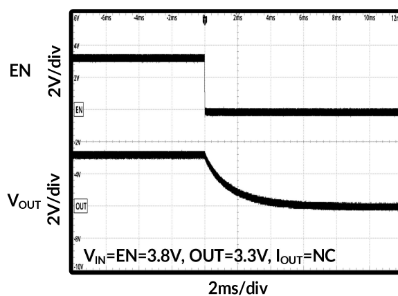
图 23. EN 关断时序
