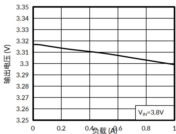
图 6. 负载调整率
