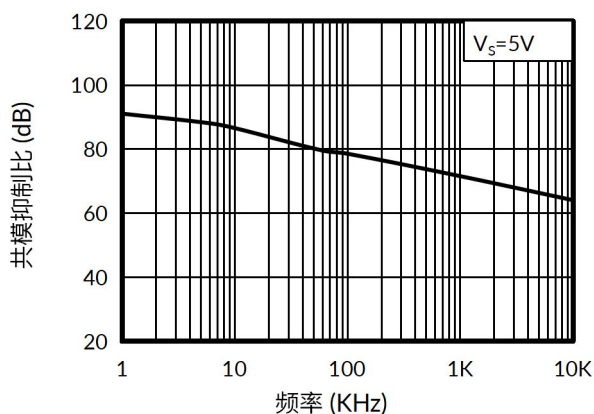
图 2. 共模抑制比与频率的关系
