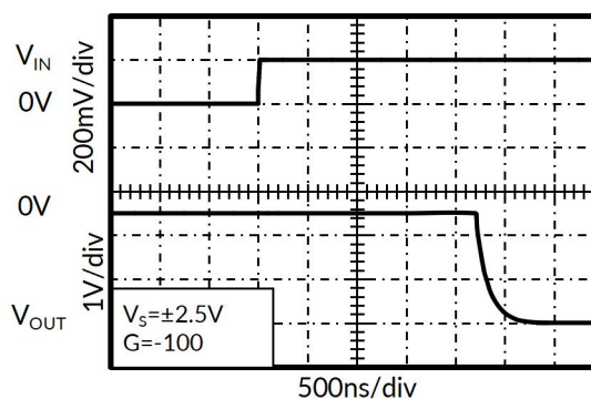
图 12. 正向过载恢复
