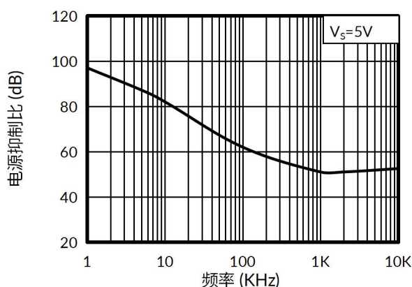
图 4. 电源抑制比与频率的关系
