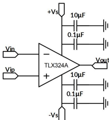
图 14. 带旁路电容器的放大器
