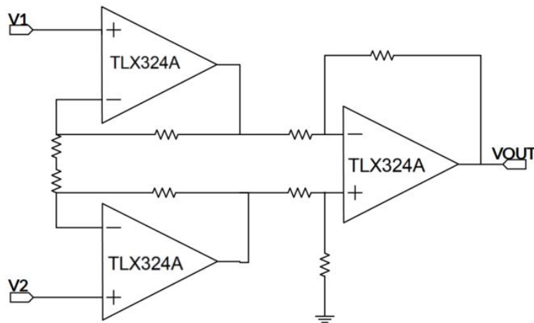
图 15. 仪表放大器
