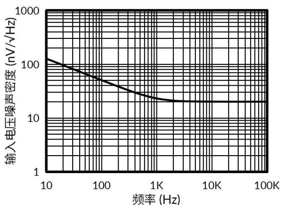
图 3. 输入电压噪声密度与频率的关系
