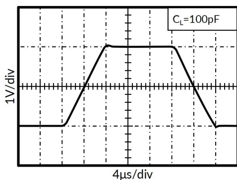
图 11. 大信号阶跃响应
