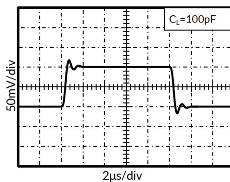
图 10. 小信号阶跃响应
