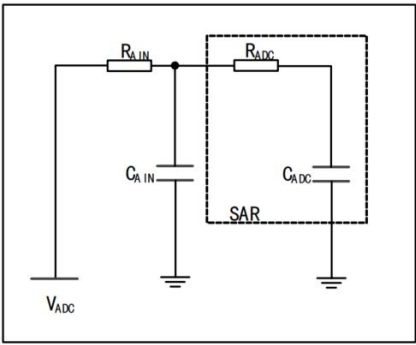
图 13 ADC 的典型应用
