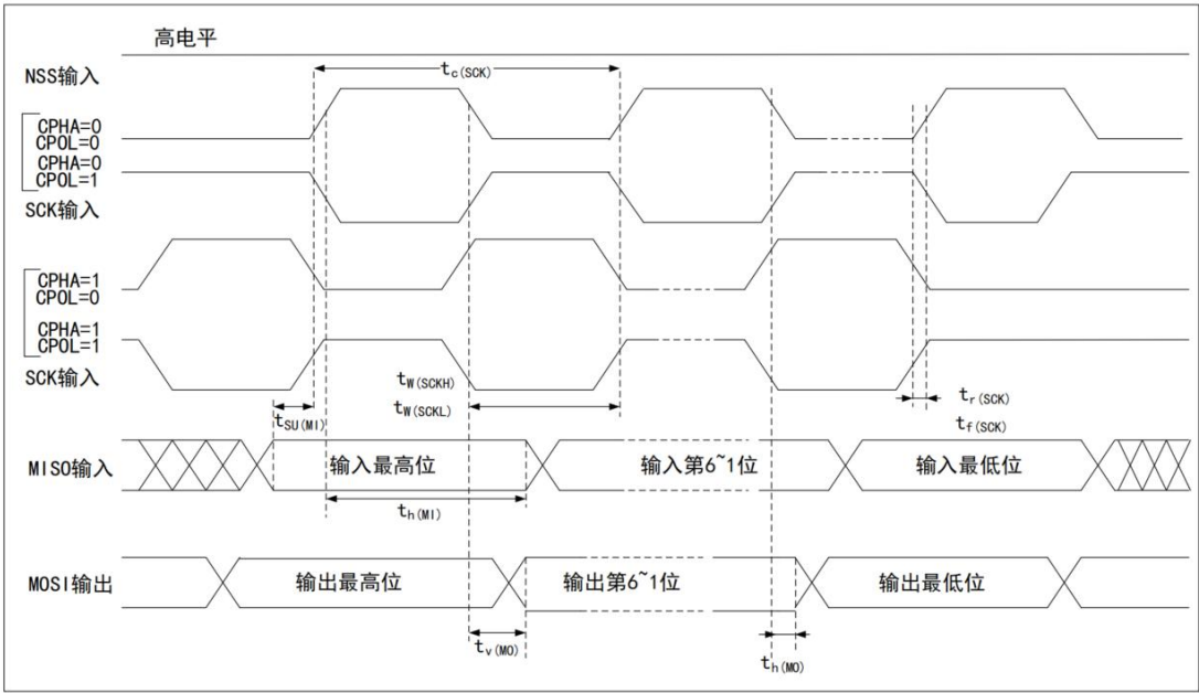
图 12 SPI 时序图—主模式(1)
