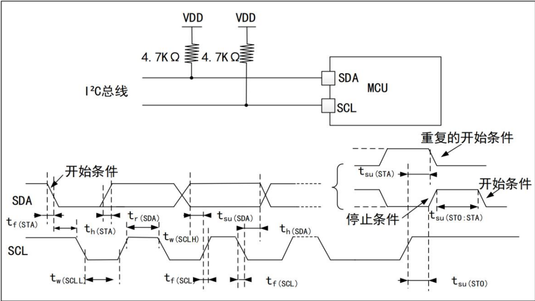
图 9 总线交流波形和测试电路
