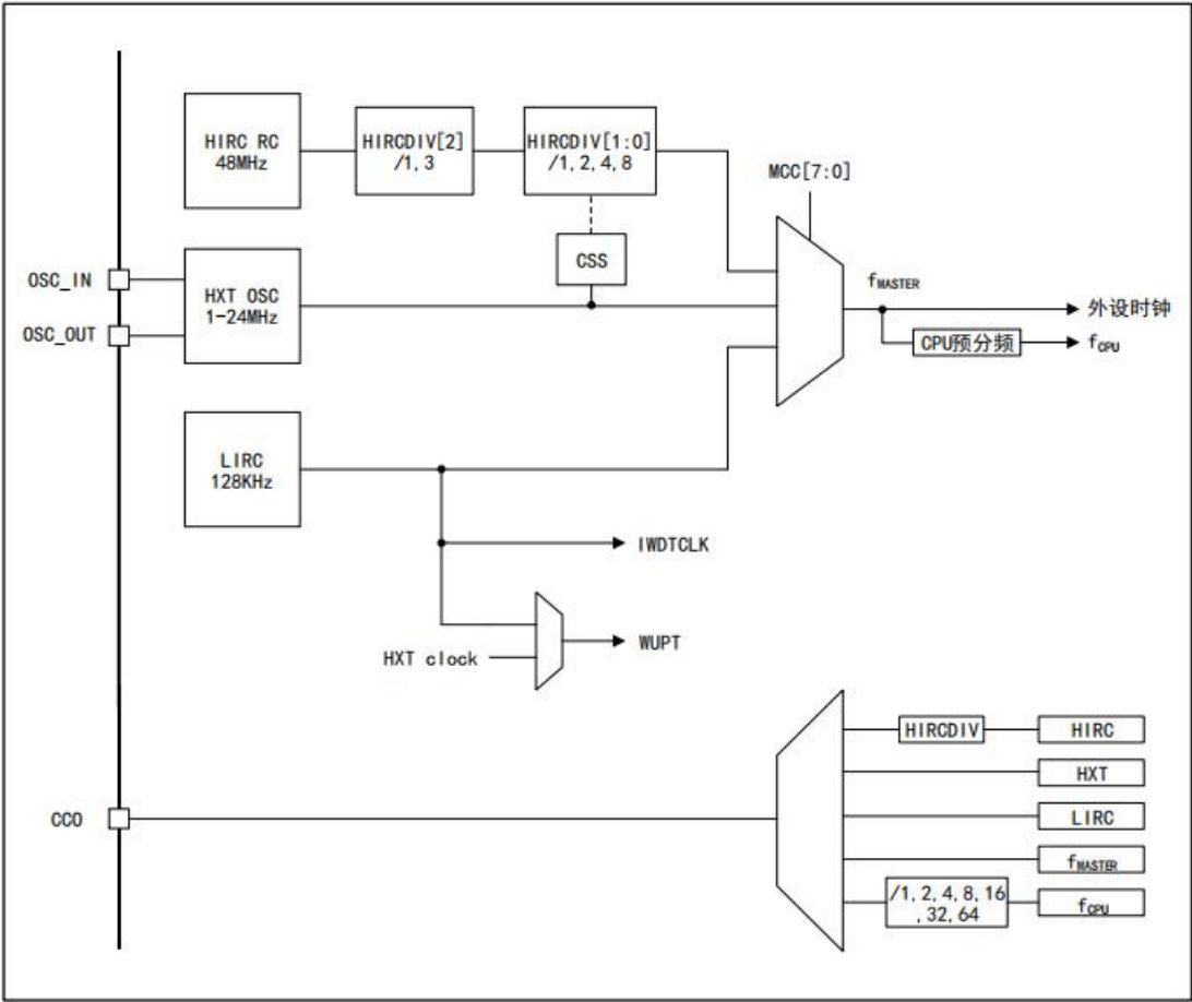
图 5 TLX32F003x4x6 系列时钟树
