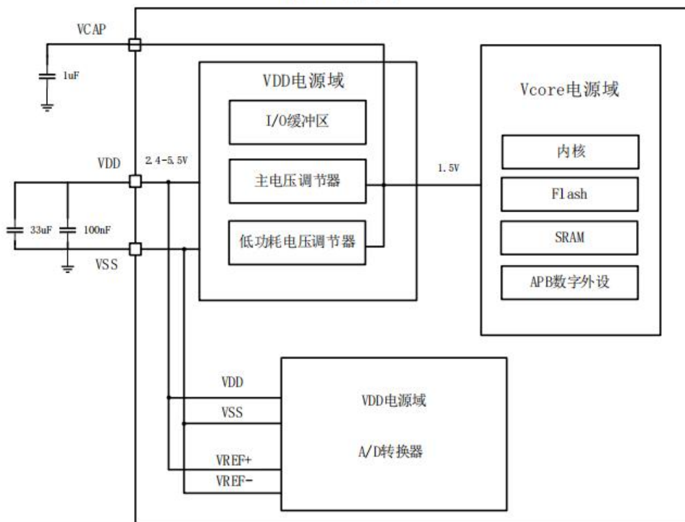
图 6 电源方案
