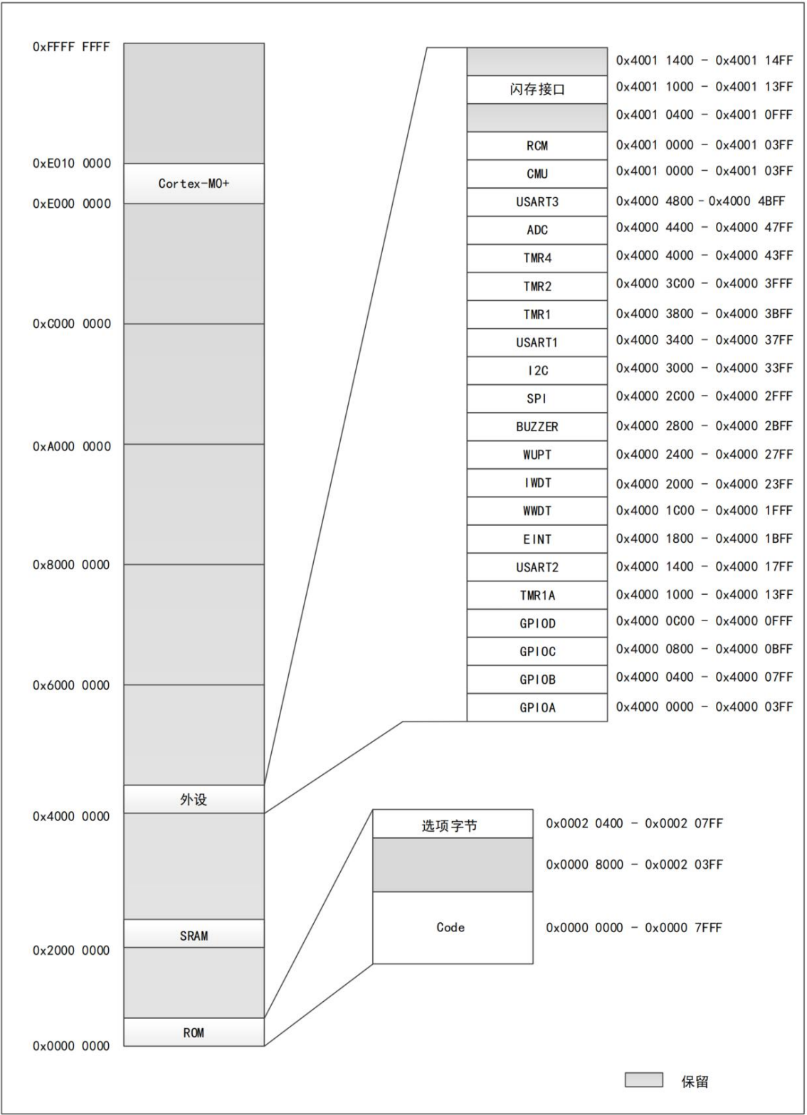
图 4 TLX32F003x4x6 系列地址映射图
