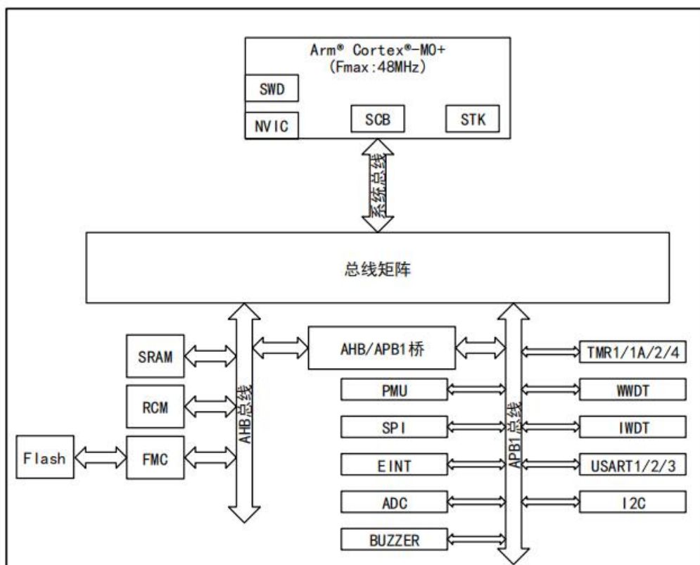
图 3 TLX32F003x4x6 系列系统框图
