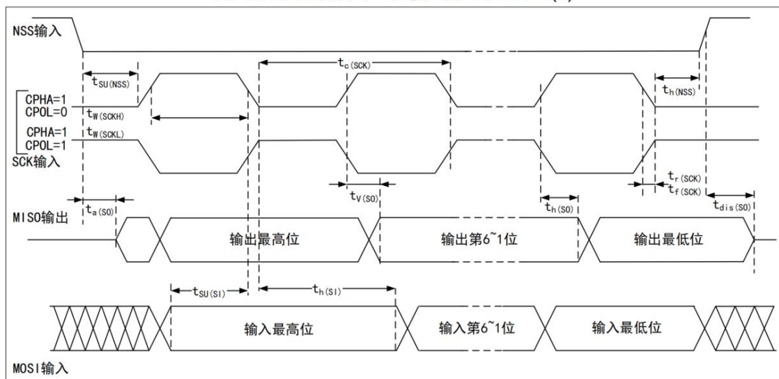
图 11 SPI 时序图—从模式和 CPHA=1(1)
