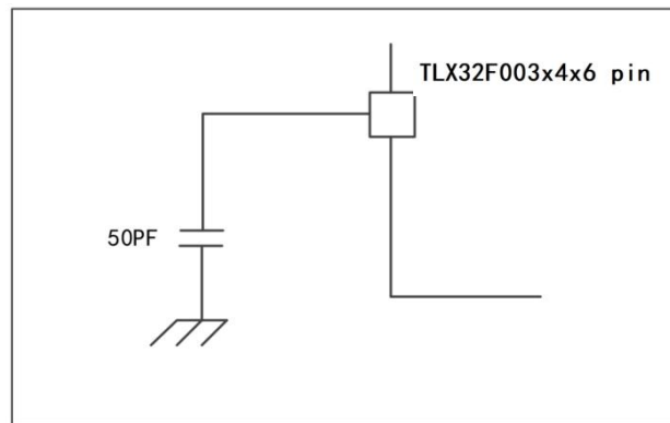
图 7 测量引脚参数时的负载条件
