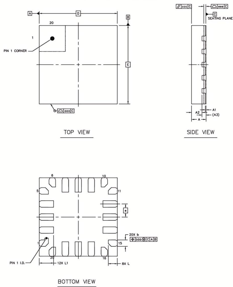
图 18 QFN20 封装图
