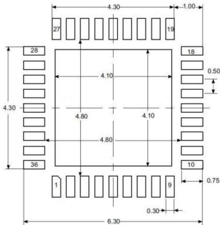
图28 QFN36 - 36 引脚, 6 x 6 mm 焊接 Layout 建议
