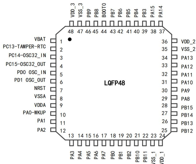
图 3 TLX32F103XB 标准型 LQFP48 引脚分布
