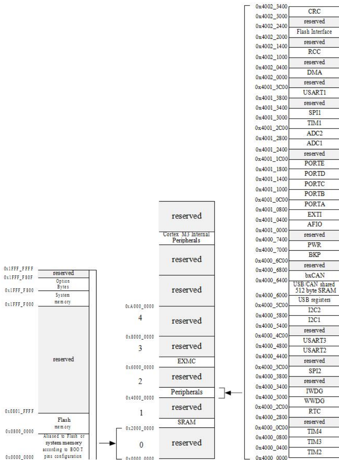
图 6 存储器 MAP 图
