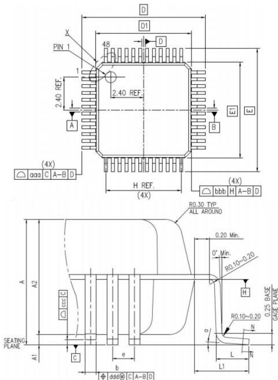
图25 LQFP48 封装图
