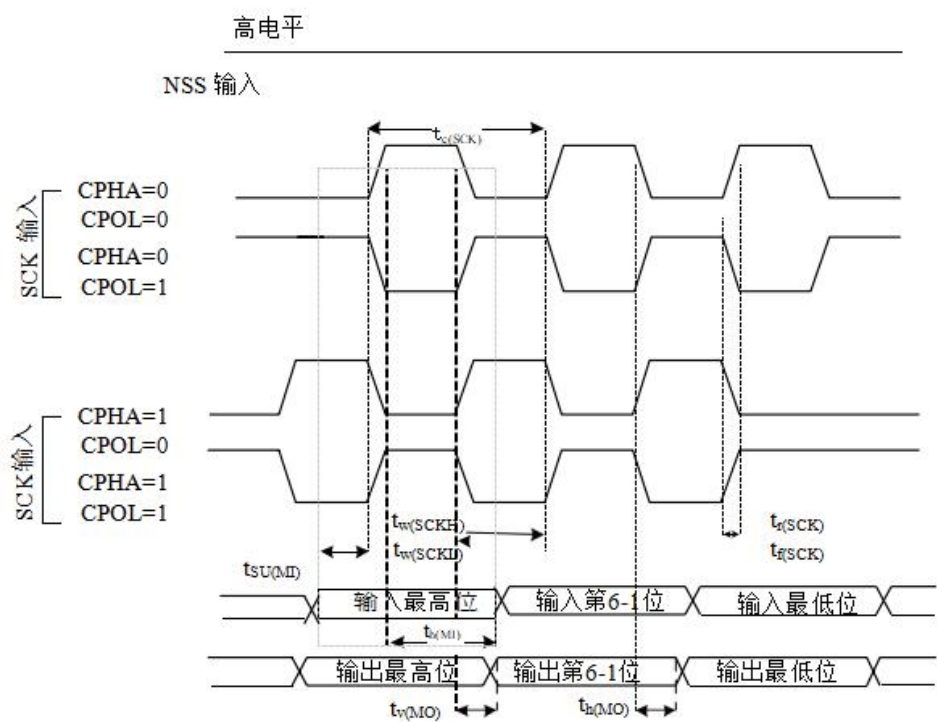
图 21 SPI 时序图-主模式 (1)
