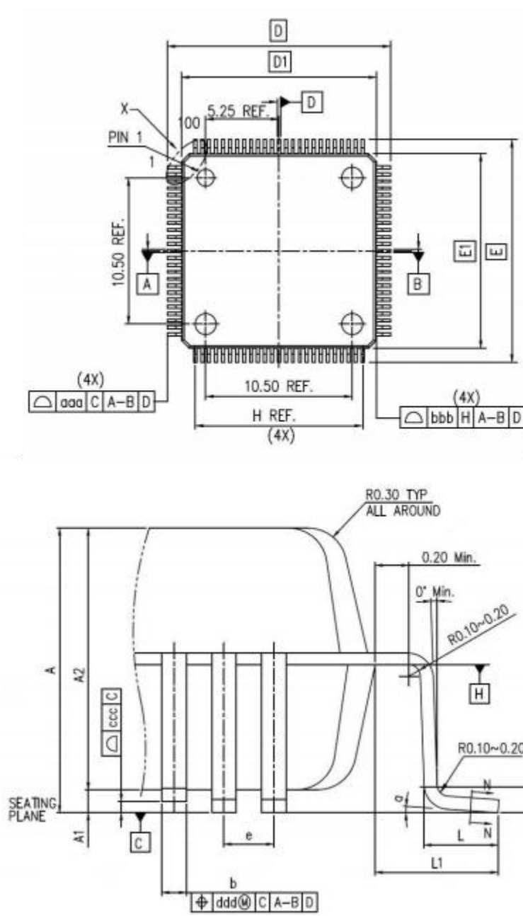
图21 LQFP100 封装图
