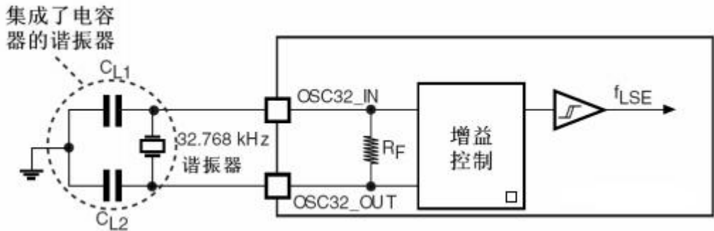
图 15 使用 32.768kHz 晶体的典型应用
