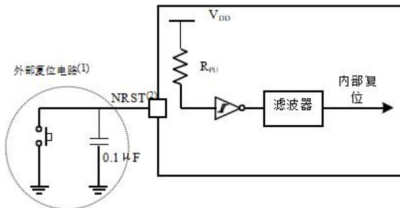
图 17 建议的 NRST 引脚保护
