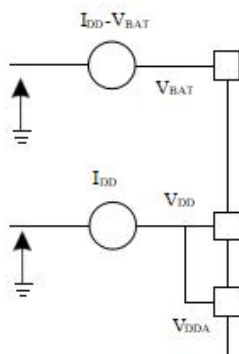
图 10 电流消耗测量方案
