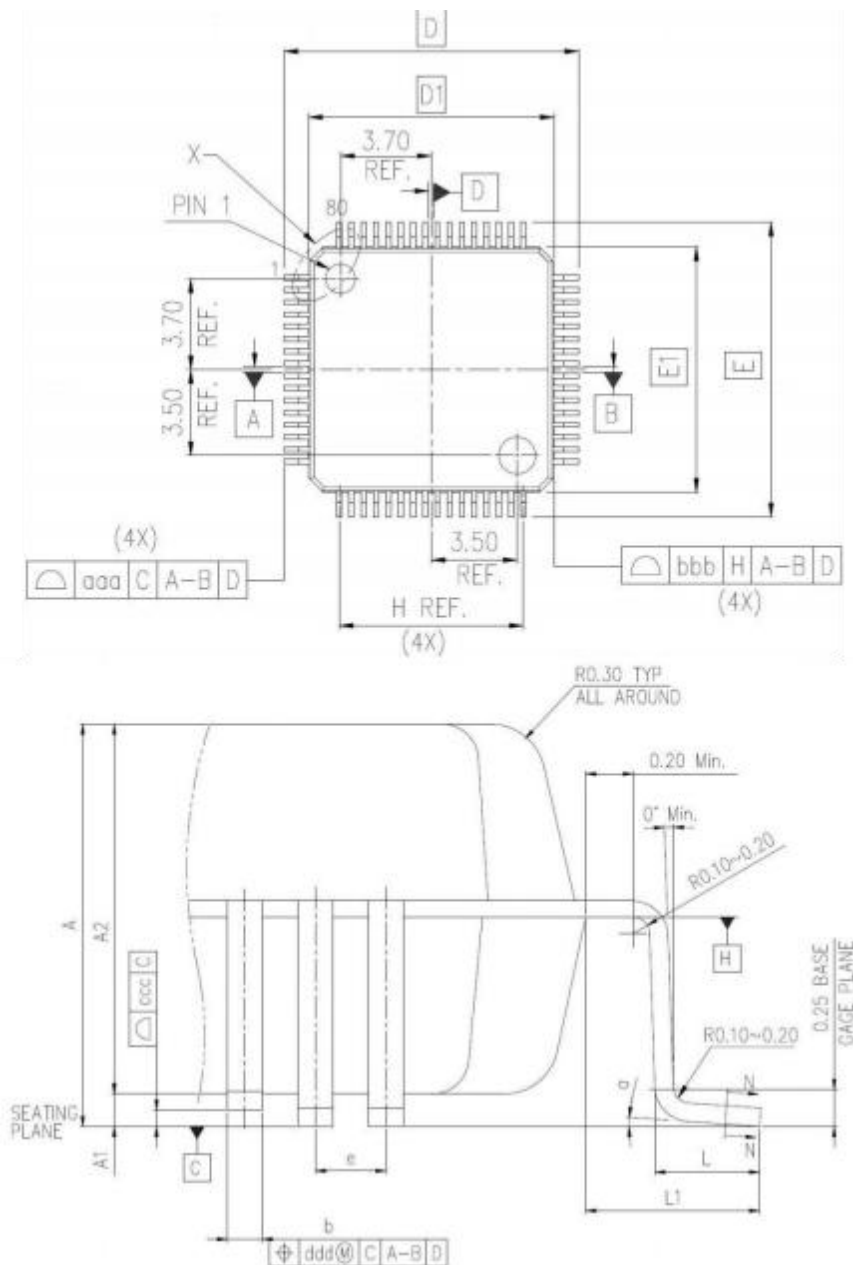
图23 LQFP64 封装图
