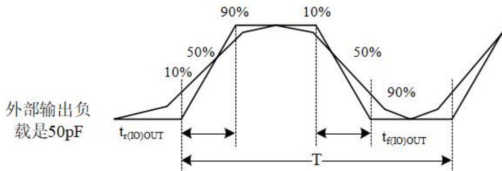
图 16 输入输出交流特性定义
