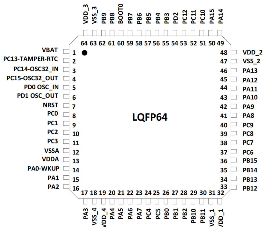
图 4 TLX32F103XB 标准型 LQFP64 引脚分布
