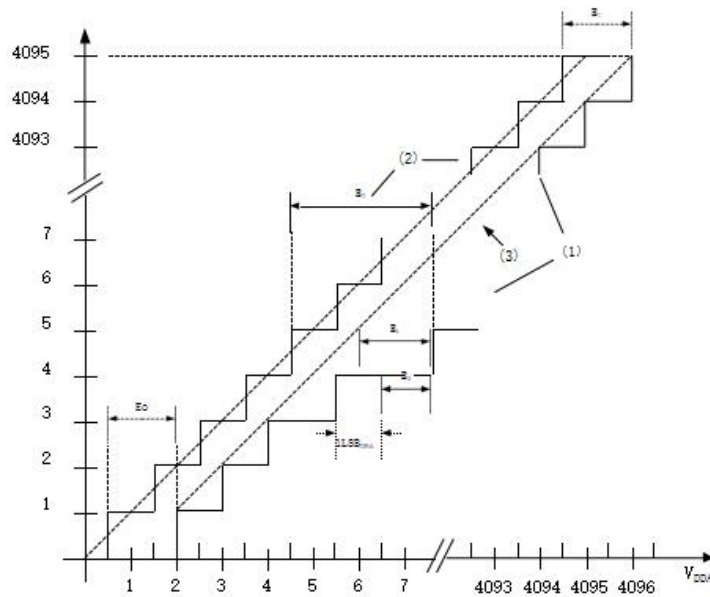
图 23 ADC 精度特性
