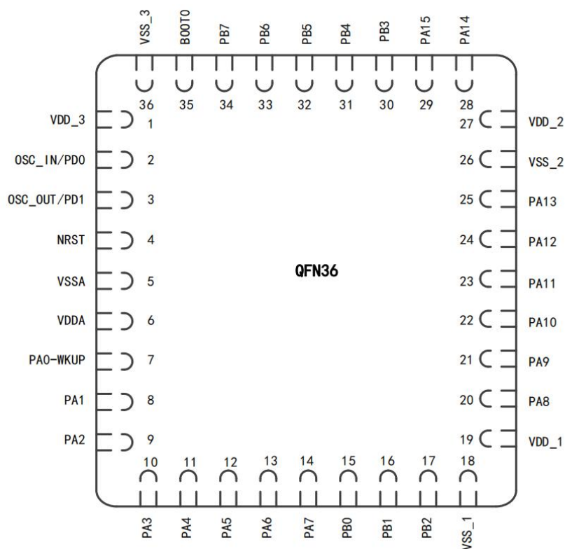
图 6 TLX32F103XB 标准型 QFN36 引脚分布
