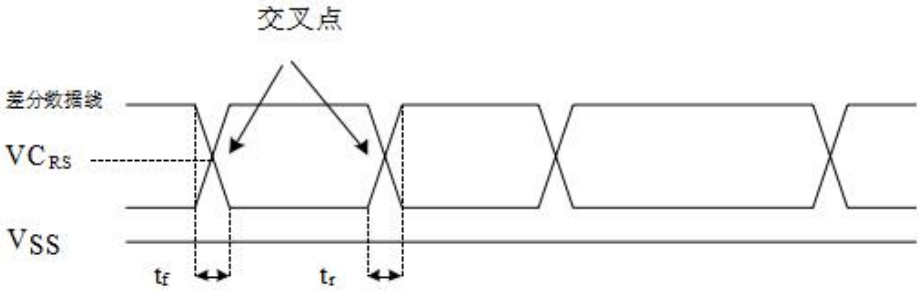
图22 USB 时序：数据信号上升和下降时间定义表
