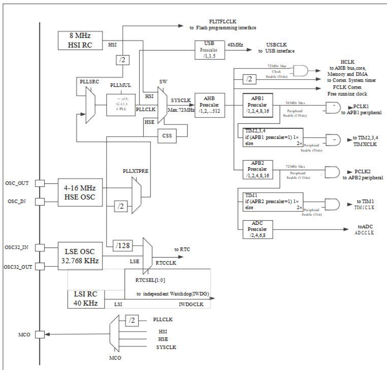
图2 时钟树
