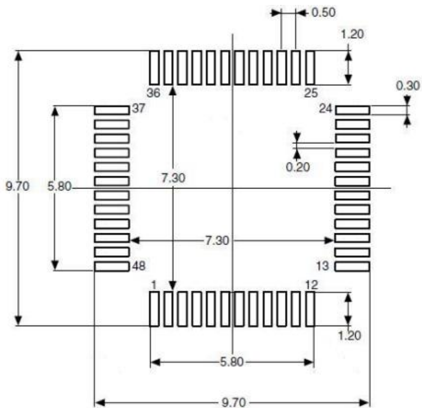
图26 LQFP48 - 48 引脚，7 x 7 mm 焊接 Layout 建议
