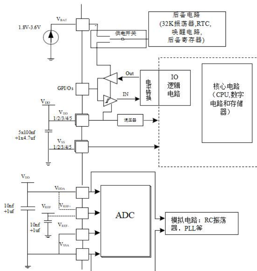
图 9 供电方案
