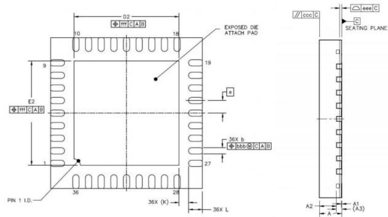
图27 QFN36 封装图
