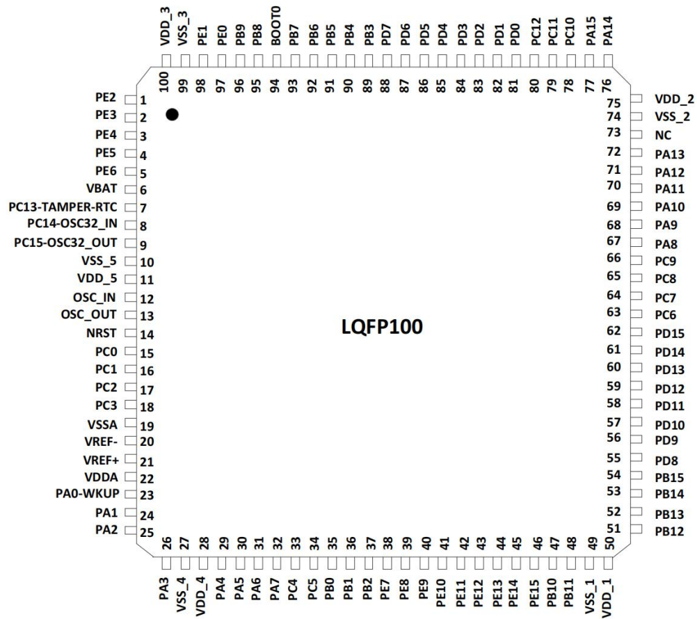
图 5 TLX32F103XB 标准型 LQFP100 引脚分布
