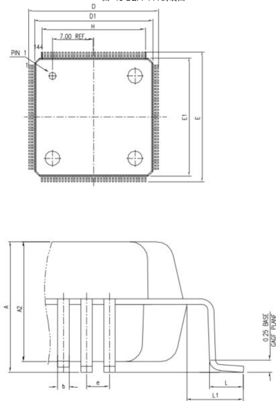
图 18 LQFP144 封装图
