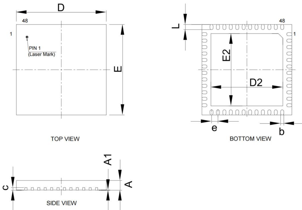
图 26 QFN48 封装图
