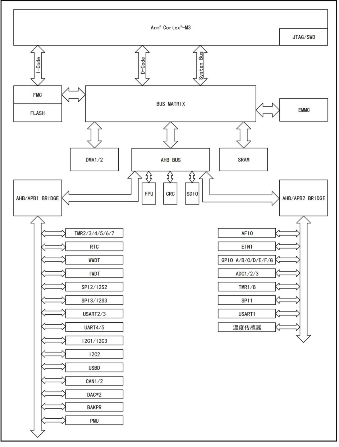
图 6 TLX32F103xE 系统框图
