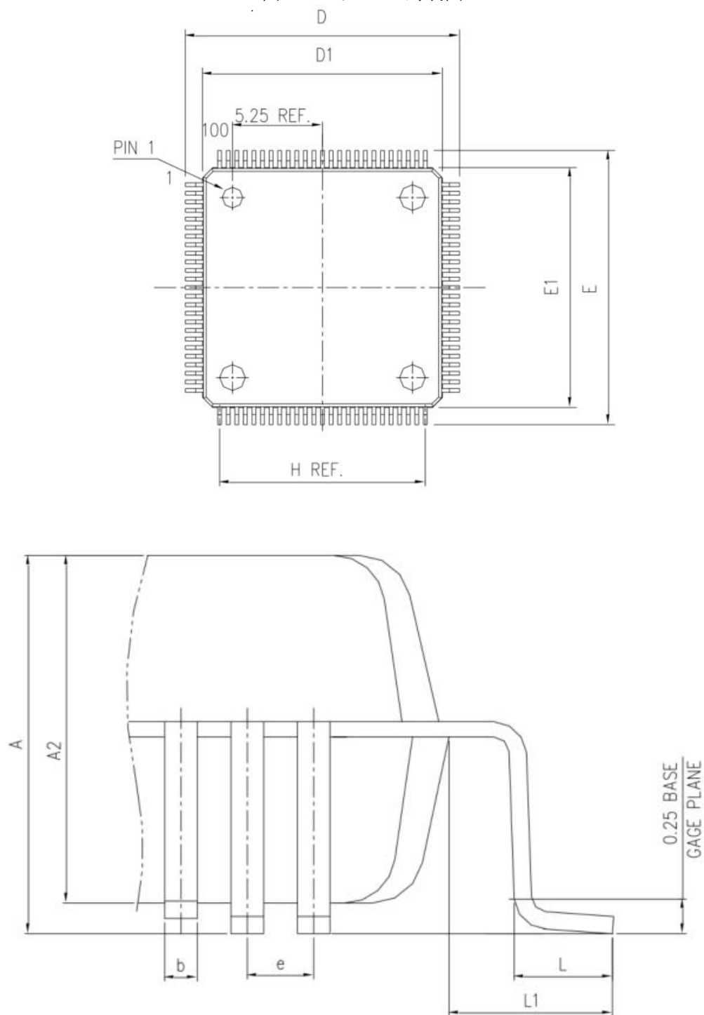
图 20 LQFP100 封装图
