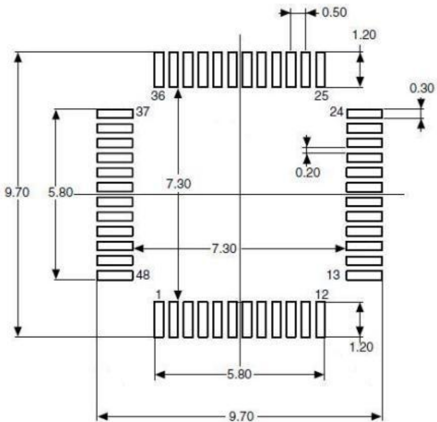
图 25 LQFP48, 7×7mm 焊接 Layout 建议
