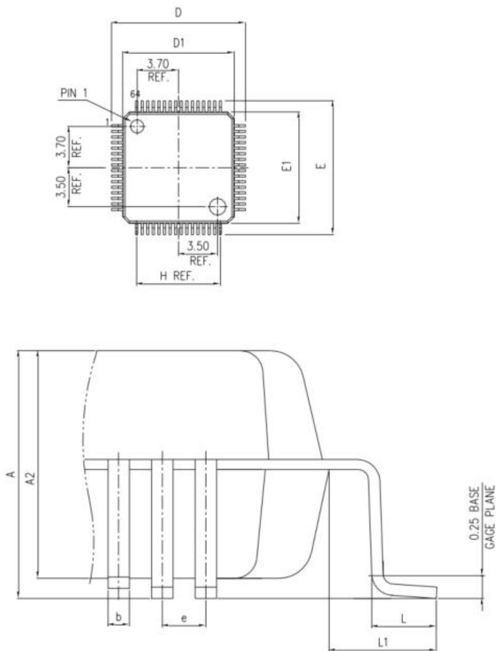
图 22 LQFP64 封装图
