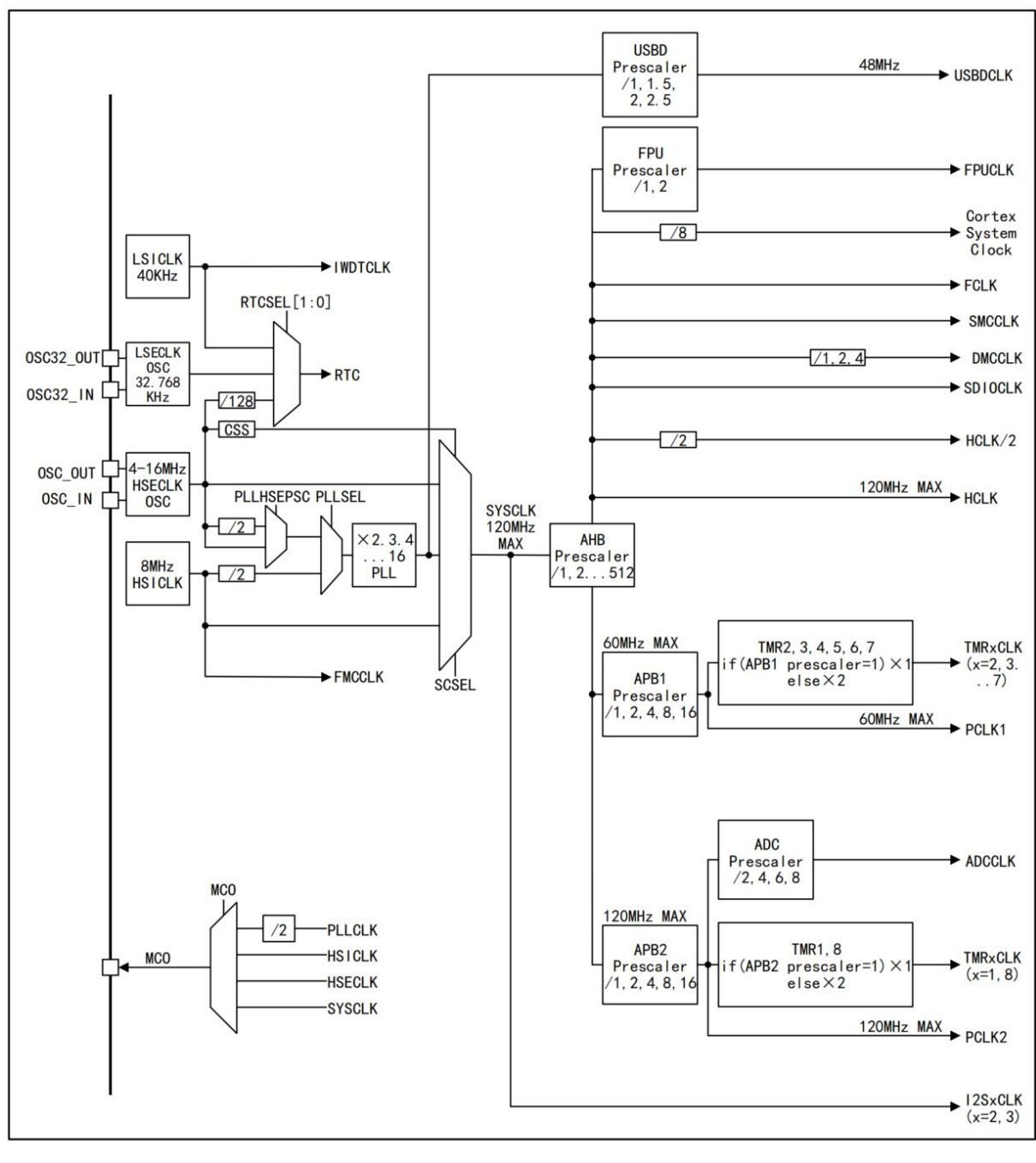
图 8 TLX32F103xE 时钟树
