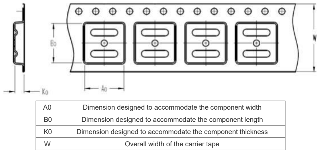
图 27 带状包装规格图
