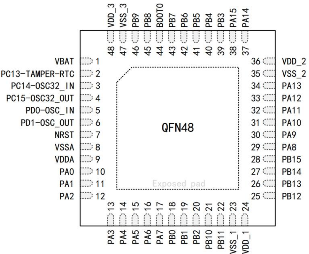
图 5 TLX32F103xE 系列 QFN48 引脚分布图
