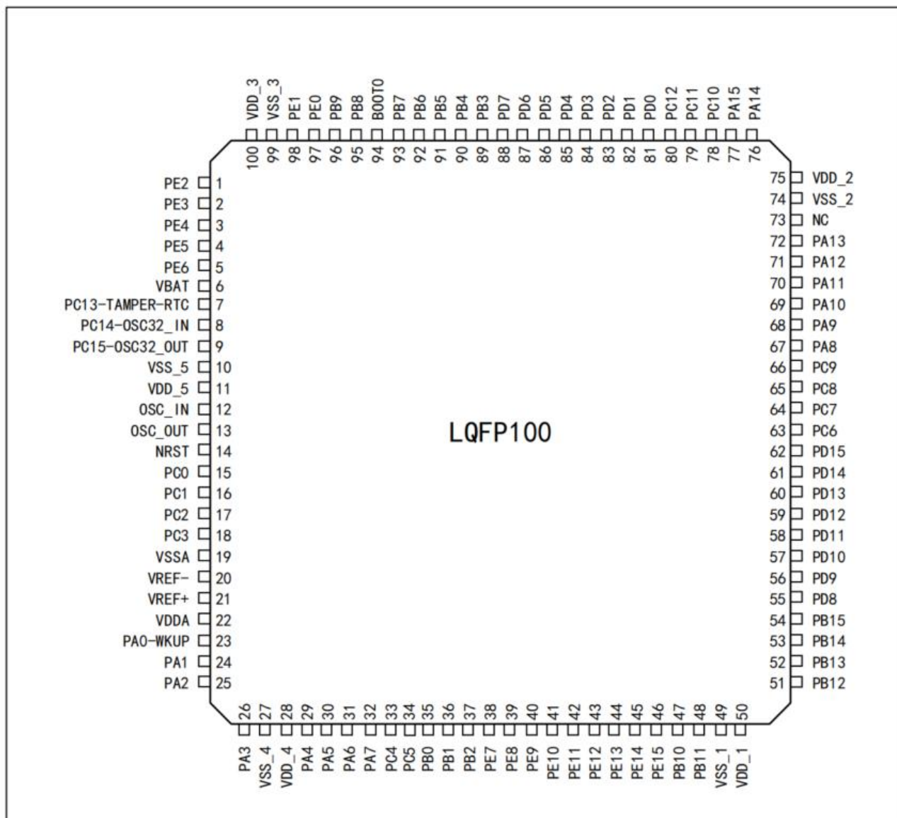
图 2 TLX32F103xE 系列 LQFP100 引脚分布图
