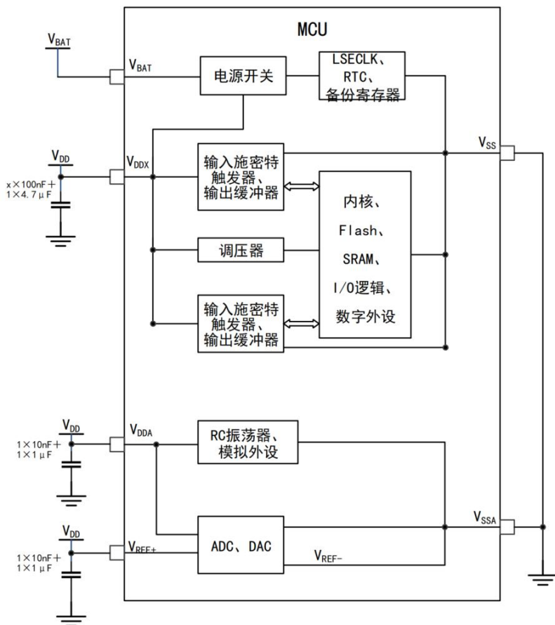
图 9 电源方案
