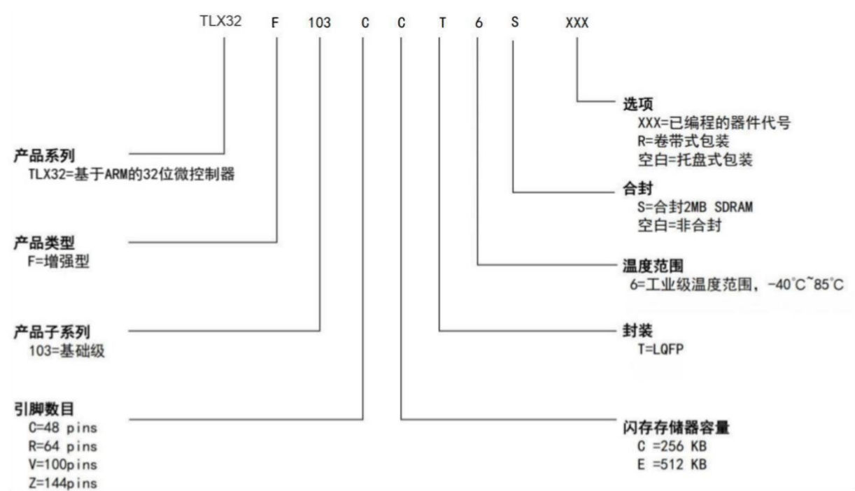
图 29 产品命名规则
