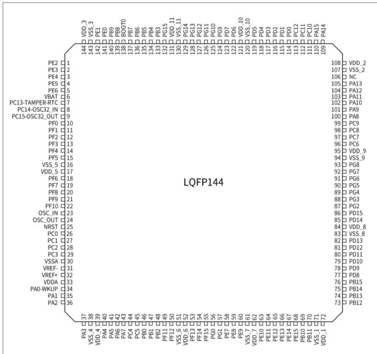
图 1 TLX32F103xE 系列 LQFP144 引脚分布图
