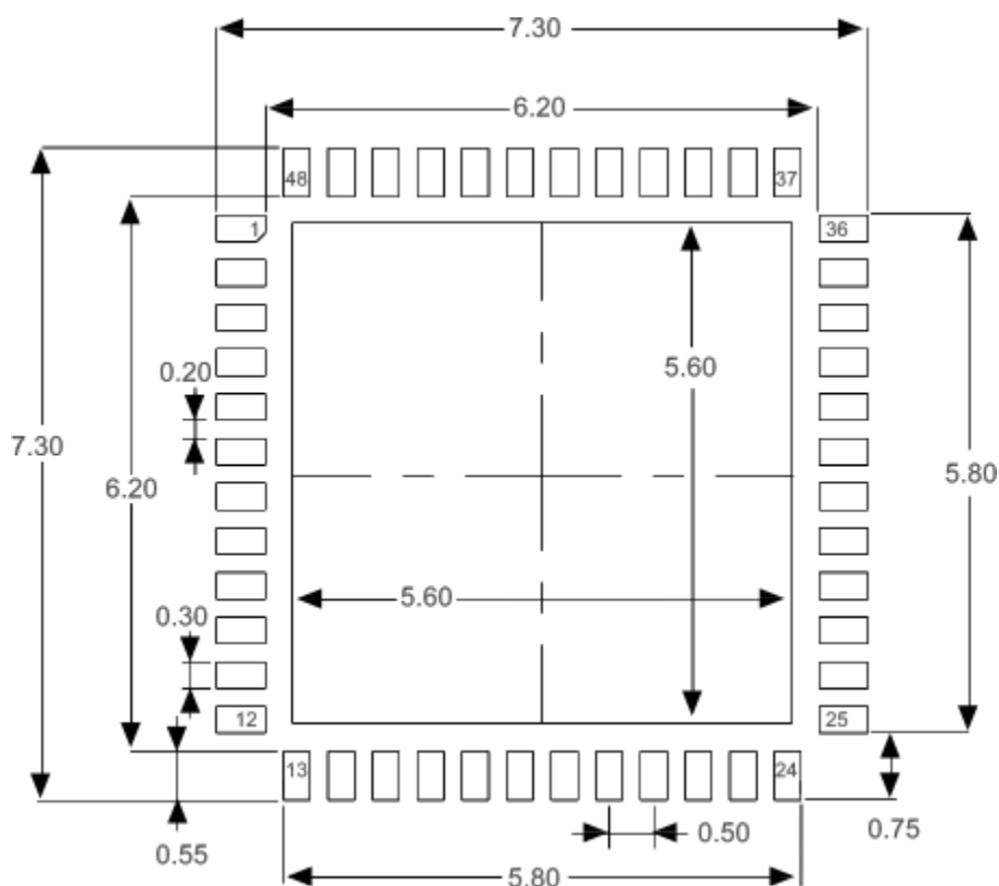
图 27 QFN48 焊接 Layout 建议
