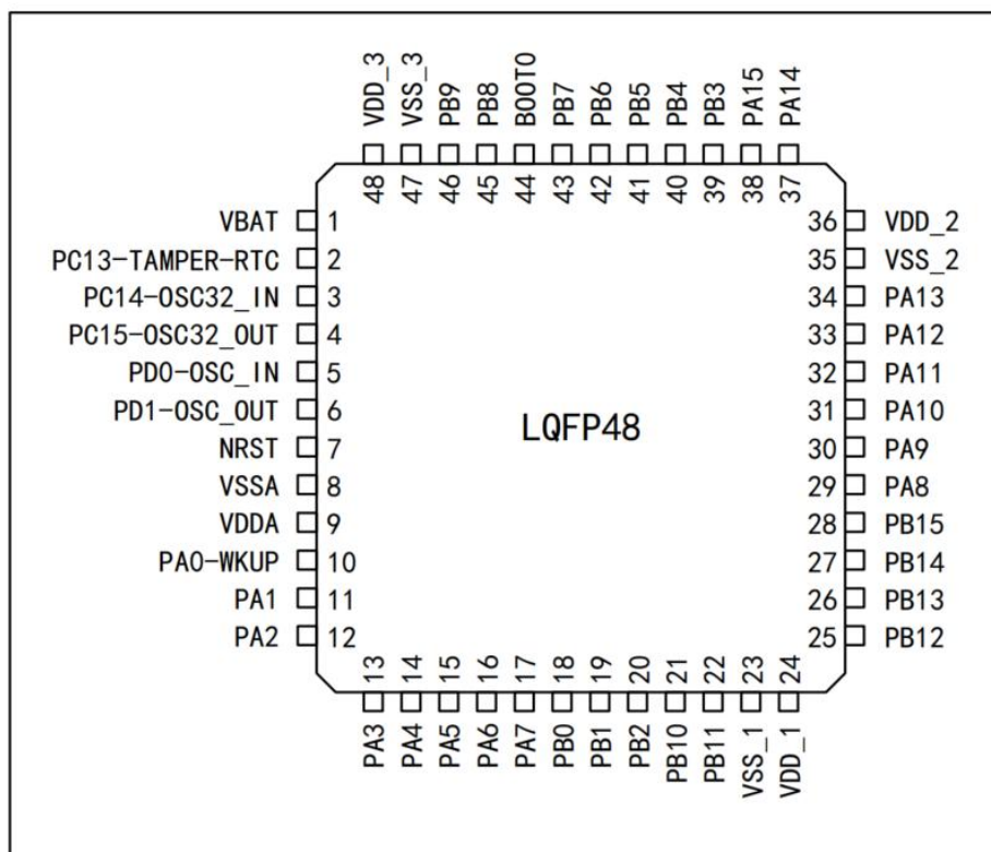
图 4 TLX32F103xE 系列 LQFP48 引脚分布图
