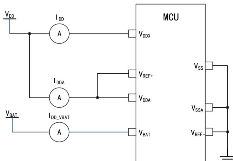
图 12 功耗测量方案
