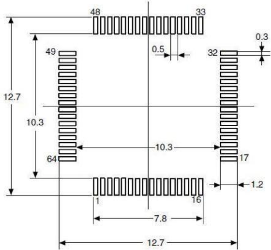
图 23 LQFP64 - 64 引脚，10 x 10mm 焊接 Layout 建议
