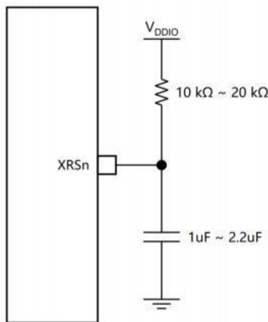
图 4.3 复位电路
