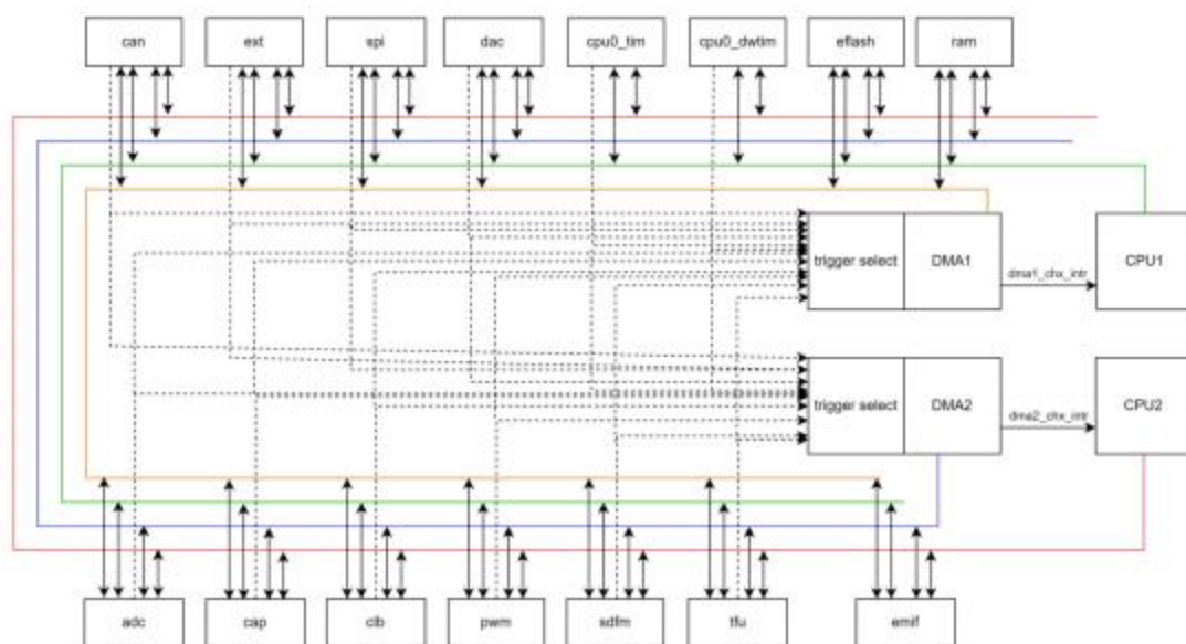
图 5.9 DMA框图
