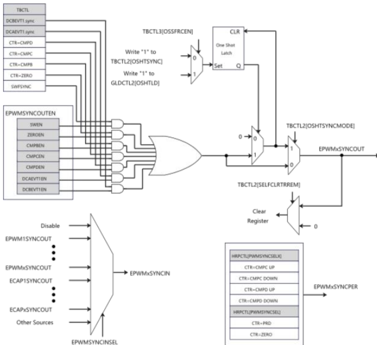
图 4.41 同步链架构
