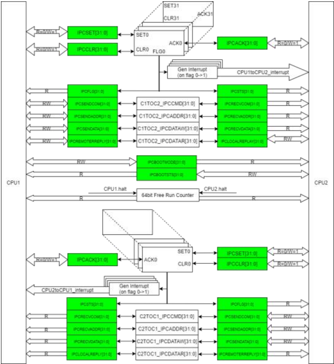
图 5.10 IPC架构
