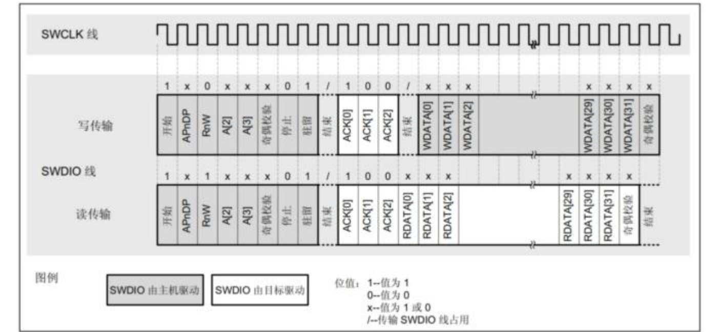
图 4.10 SWD成功的数据传输过程
