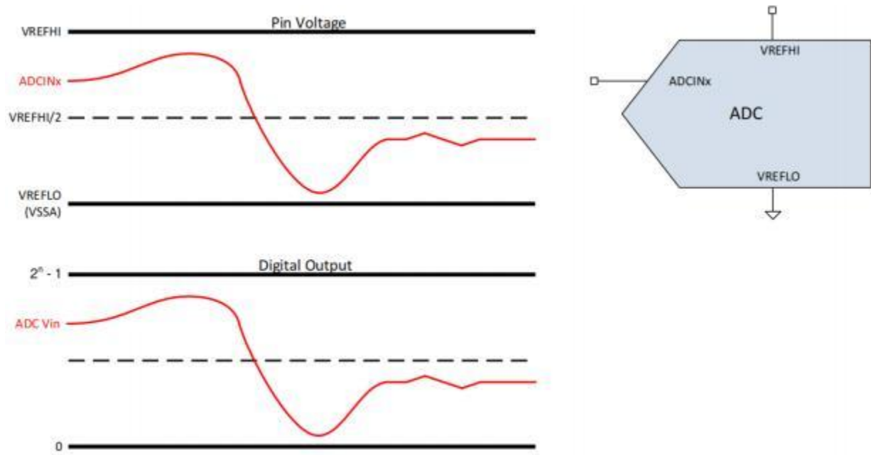
图 4.22 单端信号模式
