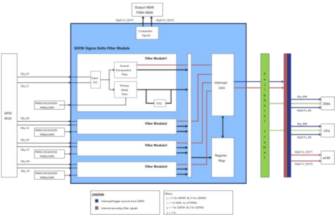
图 4.45 SDFM框图
