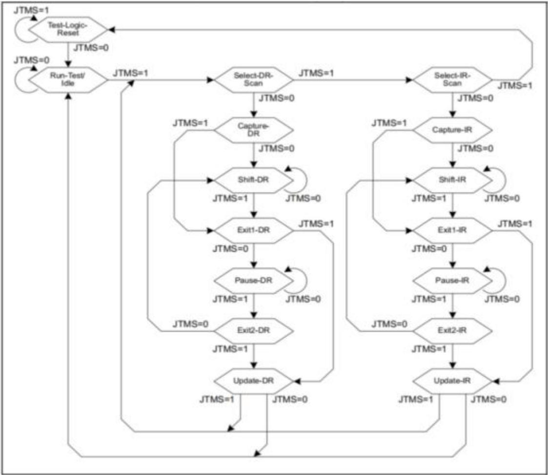
图 4.9 JTAG TAP状态机
