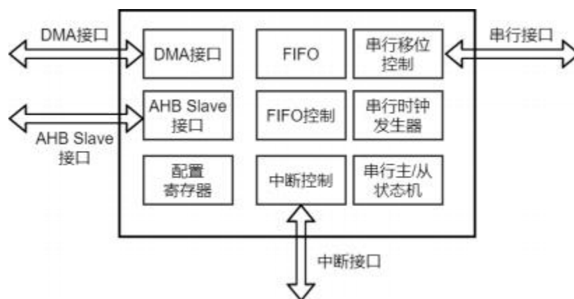
图 4.52 SPI框图
