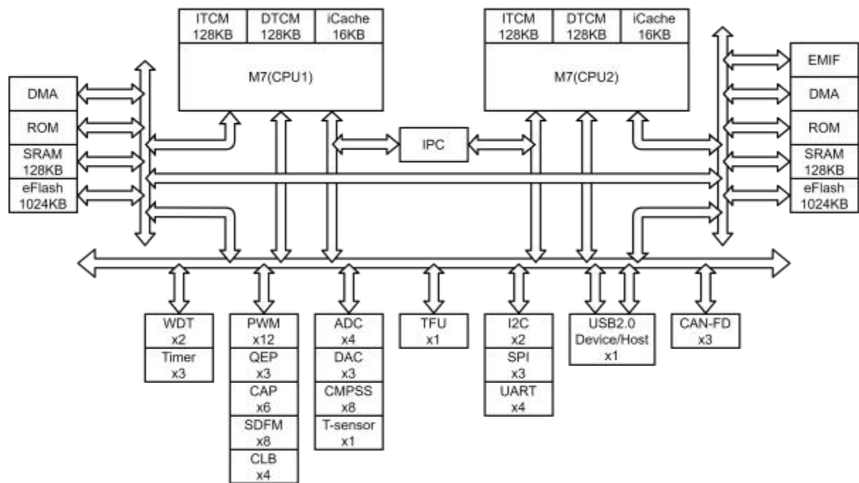
图 1.1 功能方框图
