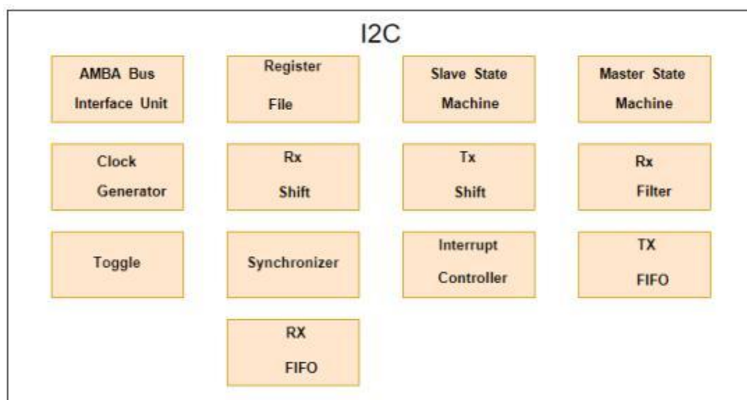
图 4.50 I2C(SMBus/PMBus)模块概念框图
