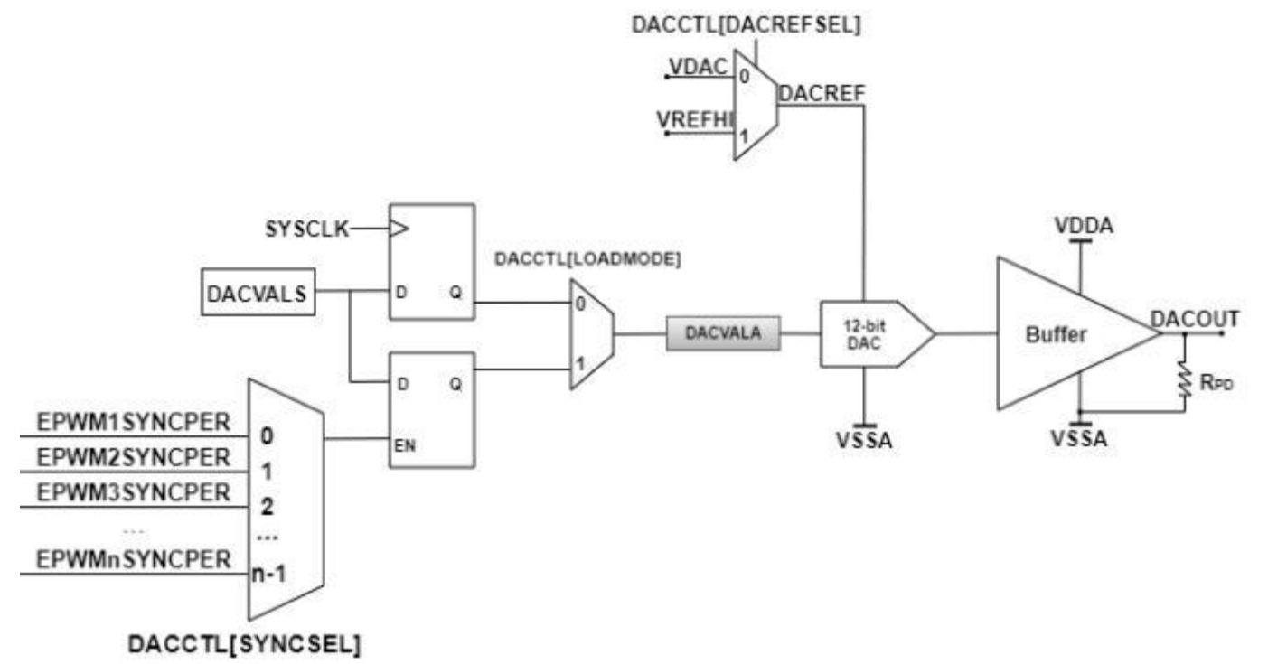
图 4.33 DAC模型框图
