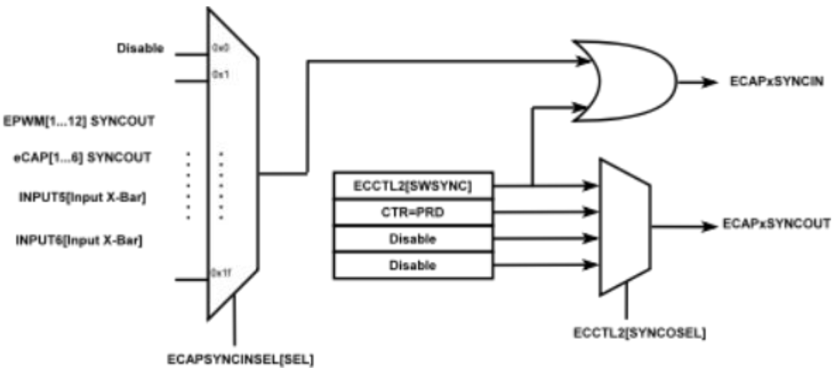
图 4.38 eCAP的同步信号
