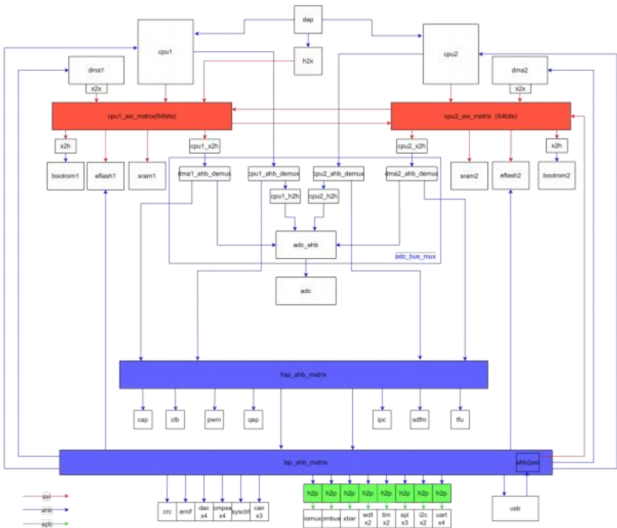
图 5.3 全芯片的总线结构
