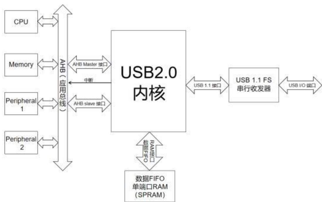
图 4.53 USB框图
