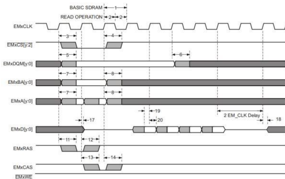
图 4.18 SDRAM读时序
