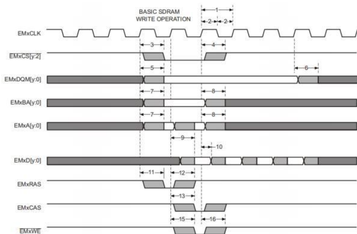
图 4.19 SDRAM写时序
