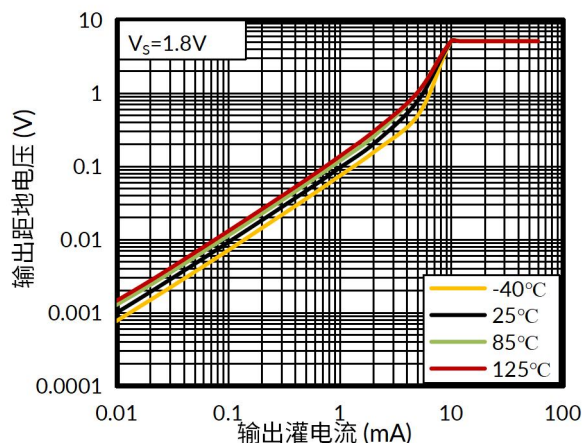
图 7. 输出电压与输出灌电流的关系
