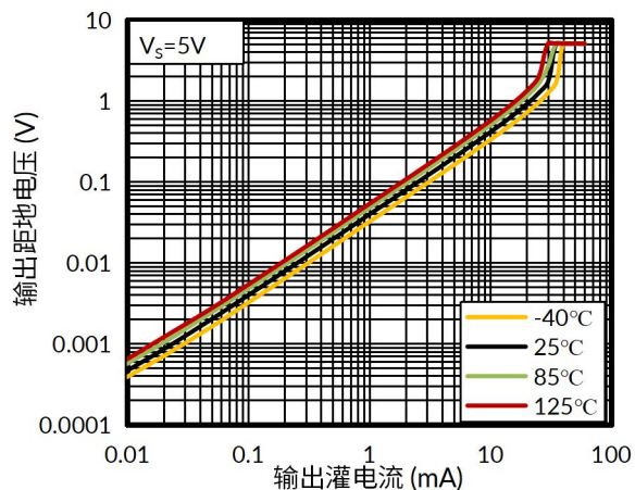
图 9. 输出电压与输出灌电流的关系
