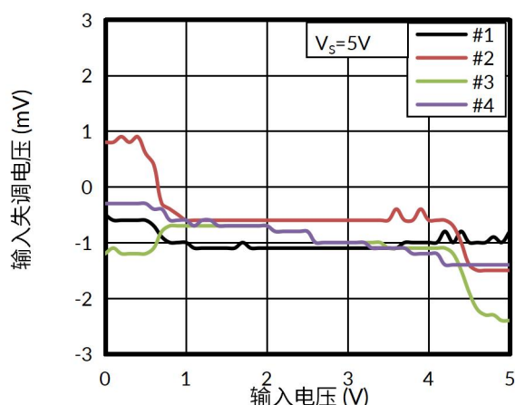
图 22. 输入失调电压与输入电压的关系, 25^{\circ}\text{C}
