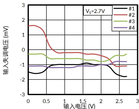
图 19. 输入失调电压与输入电压的关系, 85^{\circ}\text{C}
