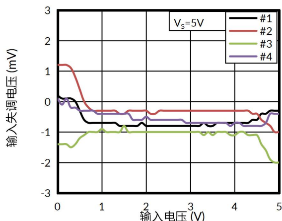
图 24. 输入失调电压与输入电压的关系, 125^{\circ}\text{C}
