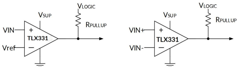
图 38. 典型应用电路
