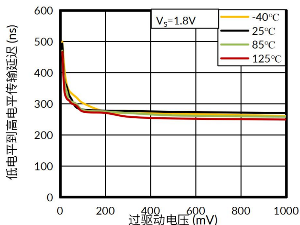
图 31. 低电平到高电平传输延迟与输入过驱动电压的关系
