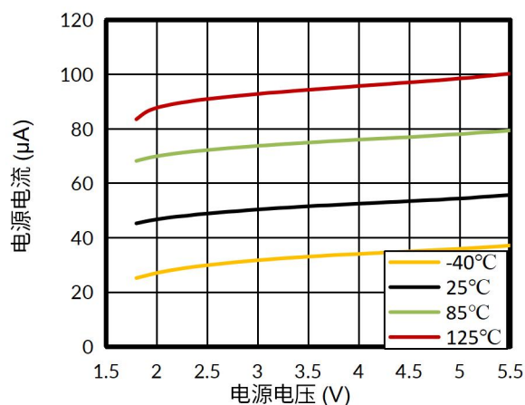
图 1. 电源电流与电源电压的关系
