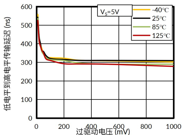
图 35. 低电平到高电平传输延迟与输入过驱动电压的关系
