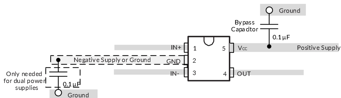
图 39. TLX331 PCB 布局示例
