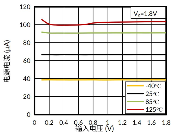
图 3. 电源电流与输入电压的关系
