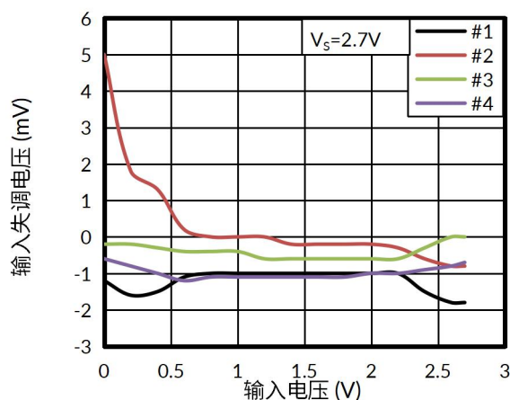
图 20. 输入失调电压与输入电压的关系, 125^{\circ}\text{C}
