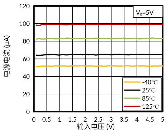
图 5. 电源电流与输入电压的关系
