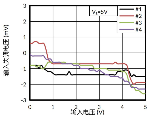
图 21. 输入失调电压与输入电压的关系, -40^{\circ}\text{C}
