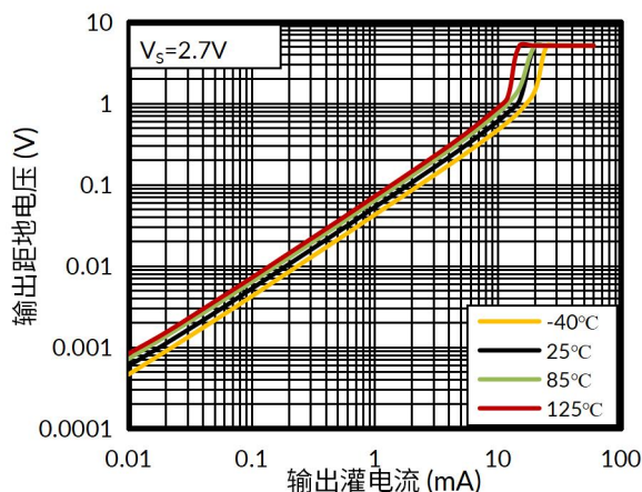
图 8. 输出电压与输出灌电流的关系
