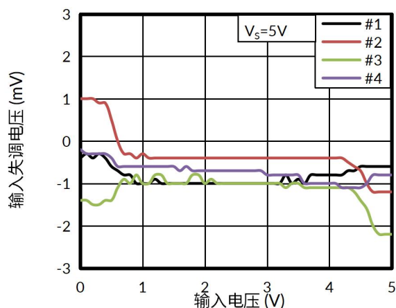
图 23. 输入失调电压与输入电压的关系, 85^{\circ}\text{C}
