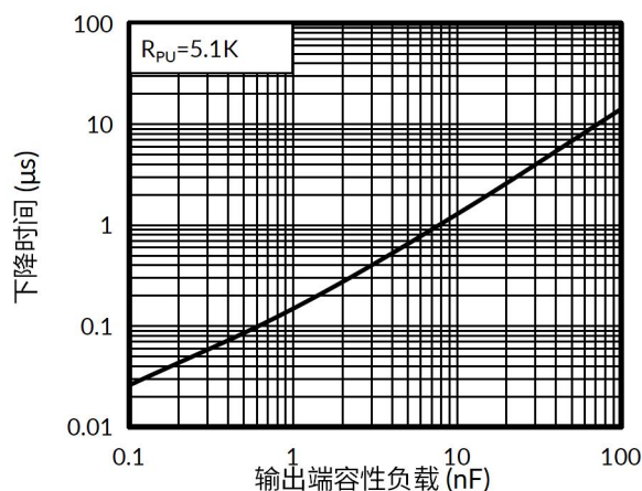
图 29. 下降时间与容性负载的关系
