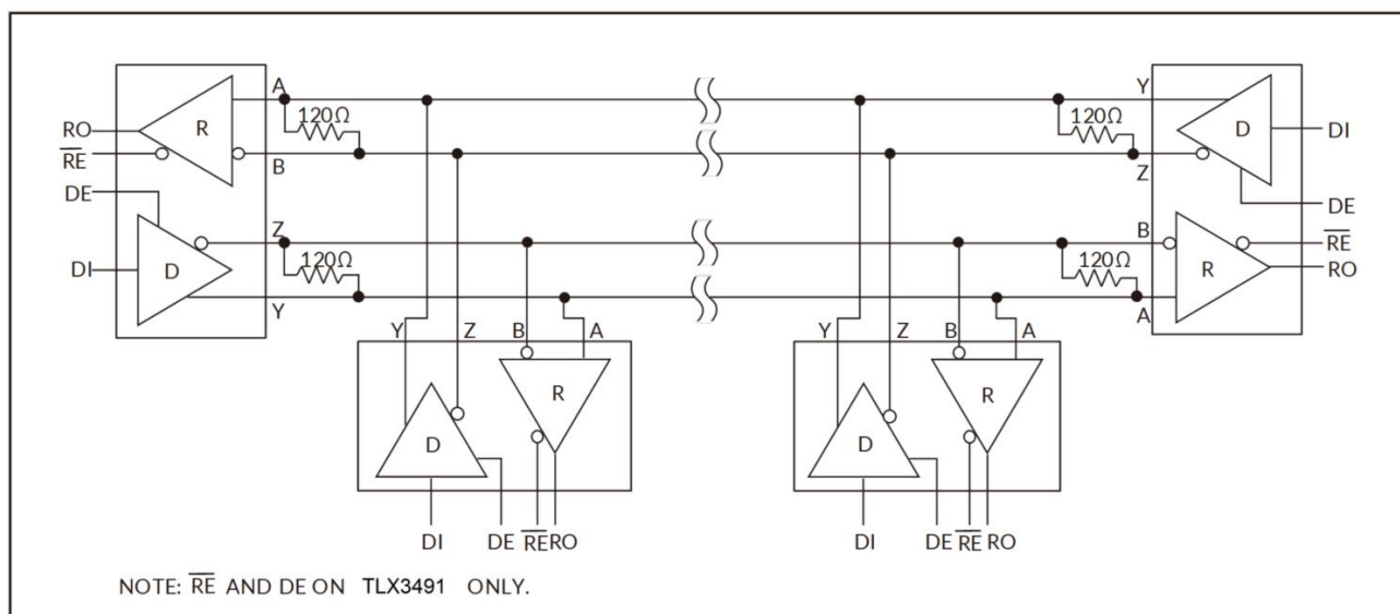
图 23. TLX3490/TLX3491 全双工 RS-485 网络
