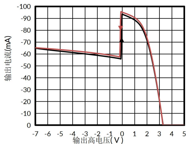
图 7. 输出电流与驱动器输出高电压
