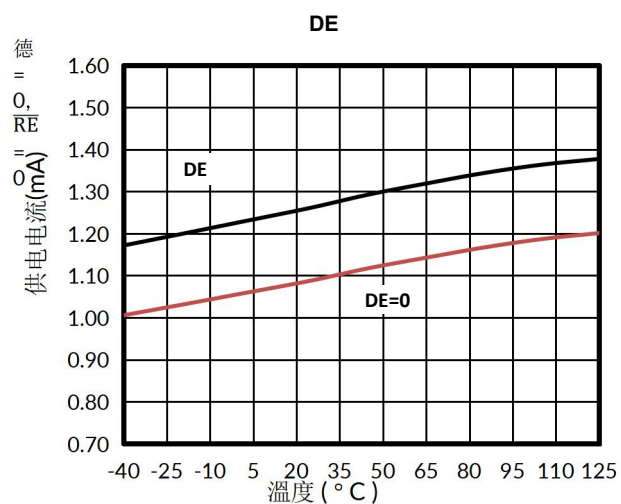
图 9. 电源电流 与温度
