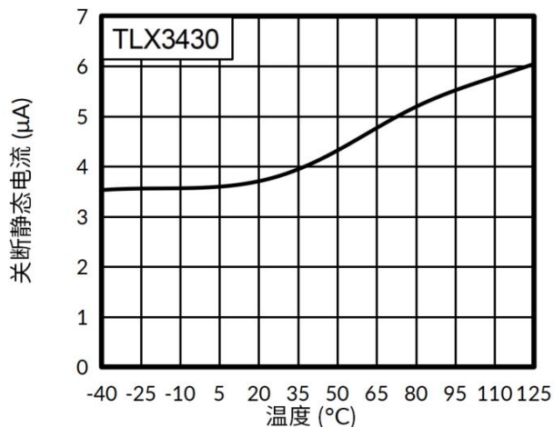
图 6. 关断模式静态电流
