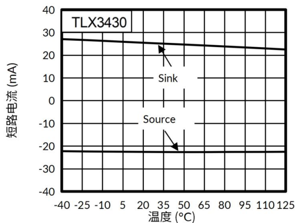
图 7. 短路电流与温度间的关系
