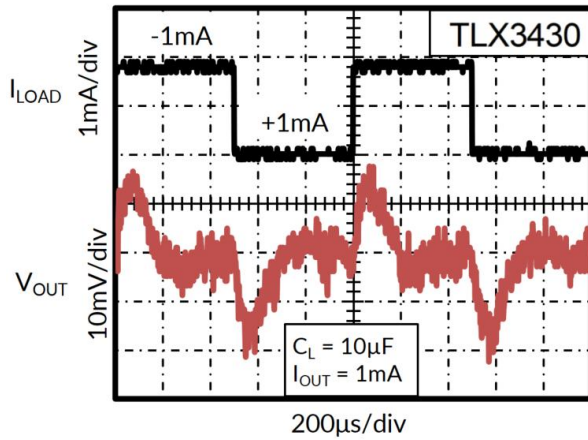
图 13. 负载调整率
