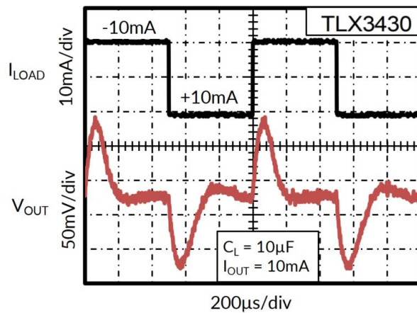
图 15. 负载调整率
