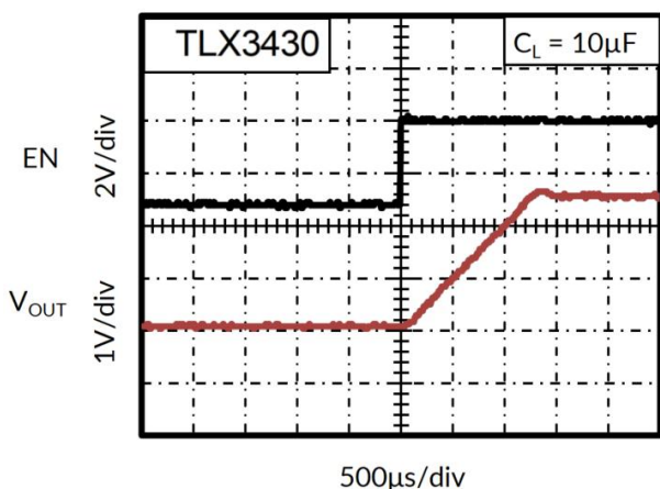
图 11. 使能导通时间
