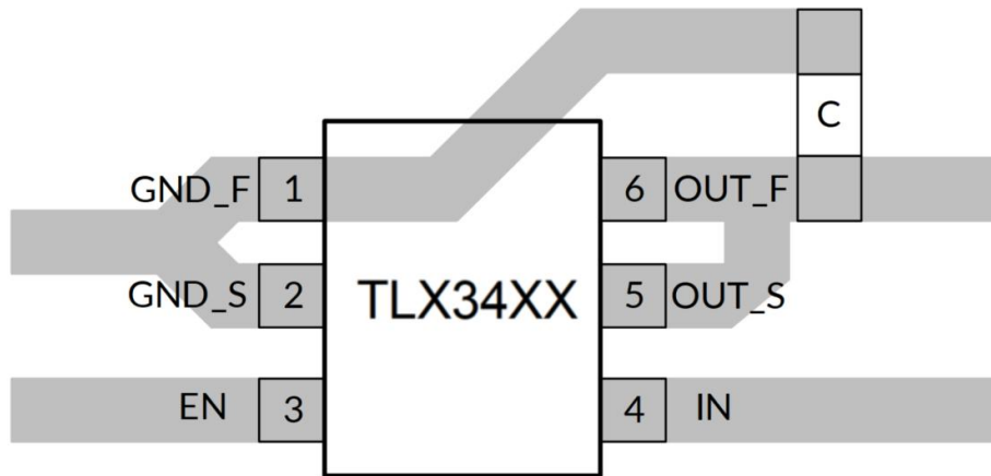
图 24. 布局示例
