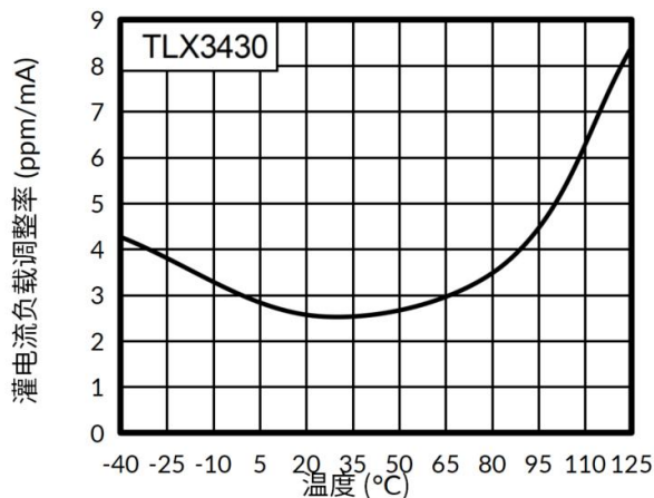
图 10. 灌电流负载调整率
