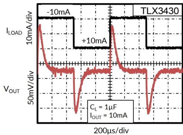
图 14. 负载调整率
