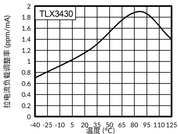
图 9. 拉电流负载调整率
