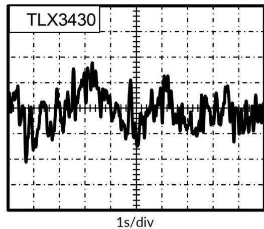
图 18. 0.1-Hz ~ 10-Hz V_{OUT} 噪声
