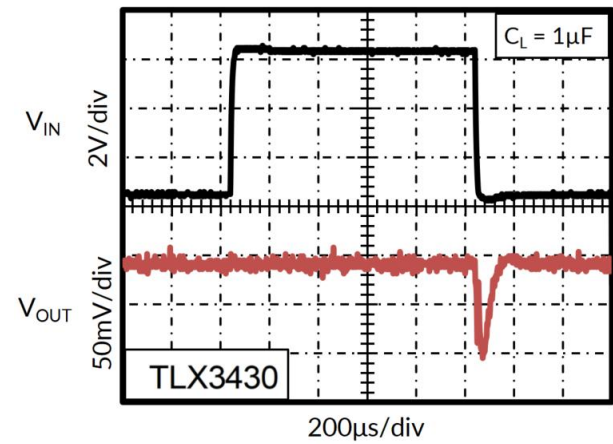
图 16. 线性调整率
