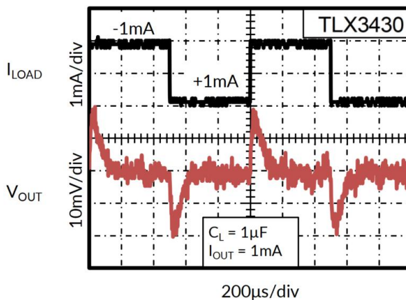
图 12. 负载调整率
