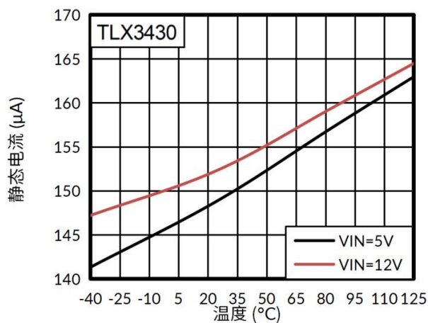
图 4. 静态电流随温度及输入电压间的关系
