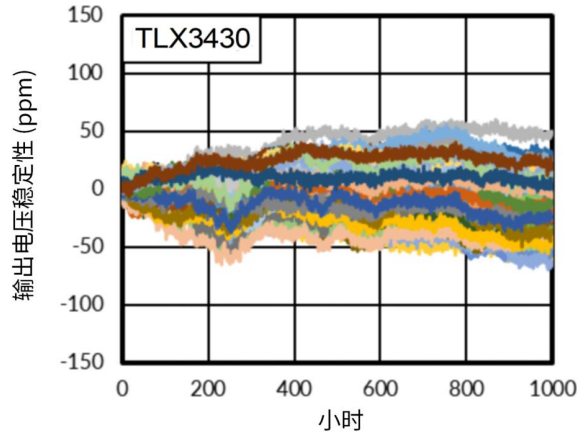
图 19. 长期稳定性 (0-1000 小时)
