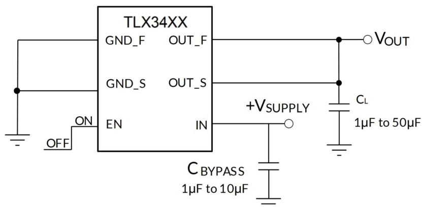
图 22. 基本连接
