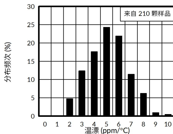
图 2. 温漂 (-55°C ~ 105°C)
