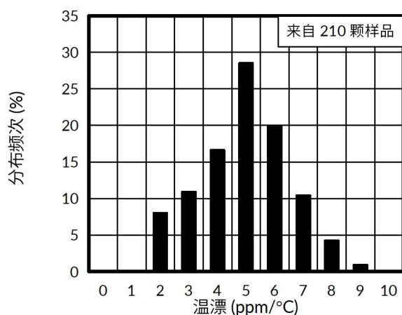
图 3. 温漂 (-55°C ~ 125°C)
