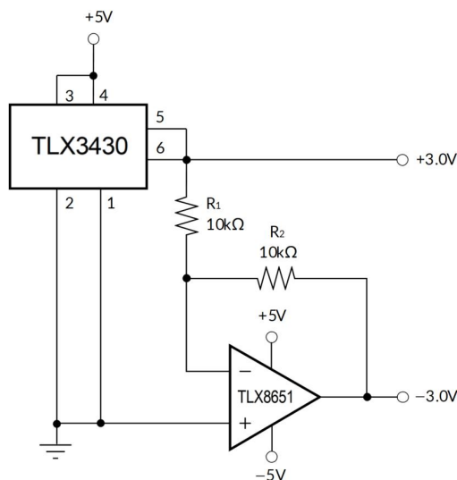
图 23. TLX3430 与 TLX8651 可产生正负基准电压
