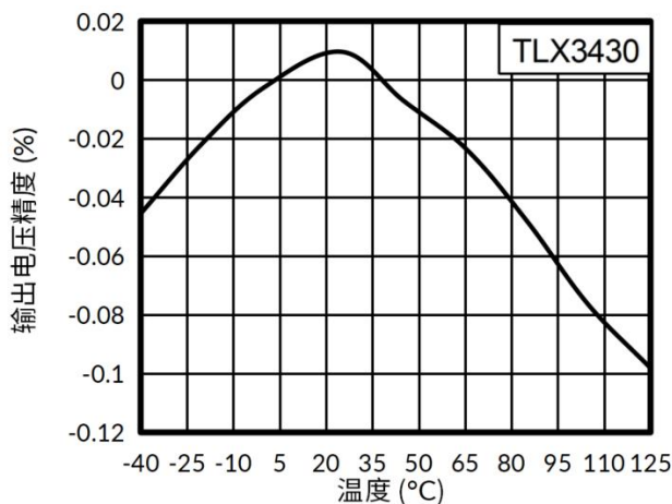
图 5. 输出电压精度与温度间的关系
