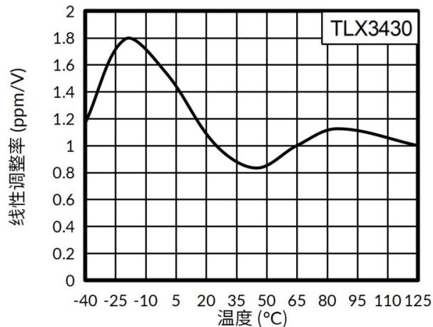
图 8. 线性调整率
