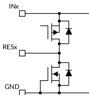
图 39. RESx 引脚
