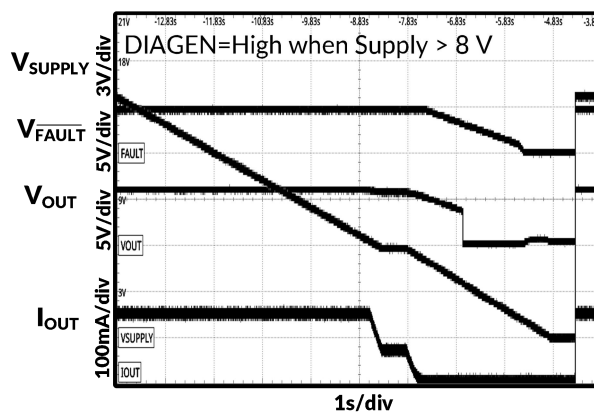
图 22. 电源电压缓慢下降和快速上升
