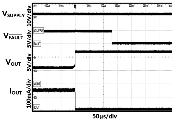
图 16. LED 开路保护
