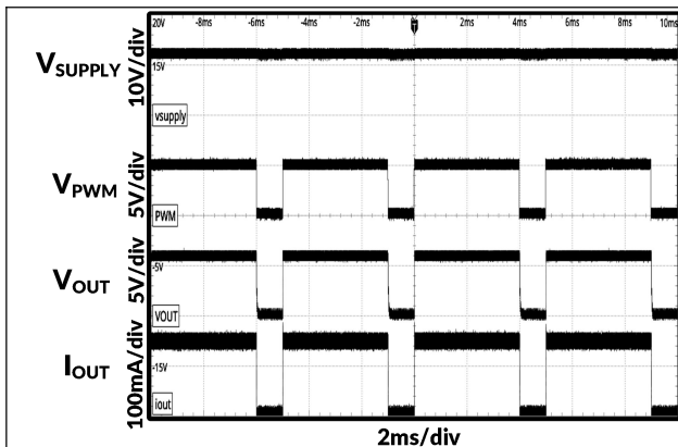
图 45. 80%占空比下的 200Hz PWM 调光
