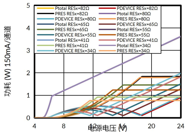
图 11. 功耗与电源电压的关系
