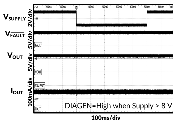
图 20. 瞬态欠电压
