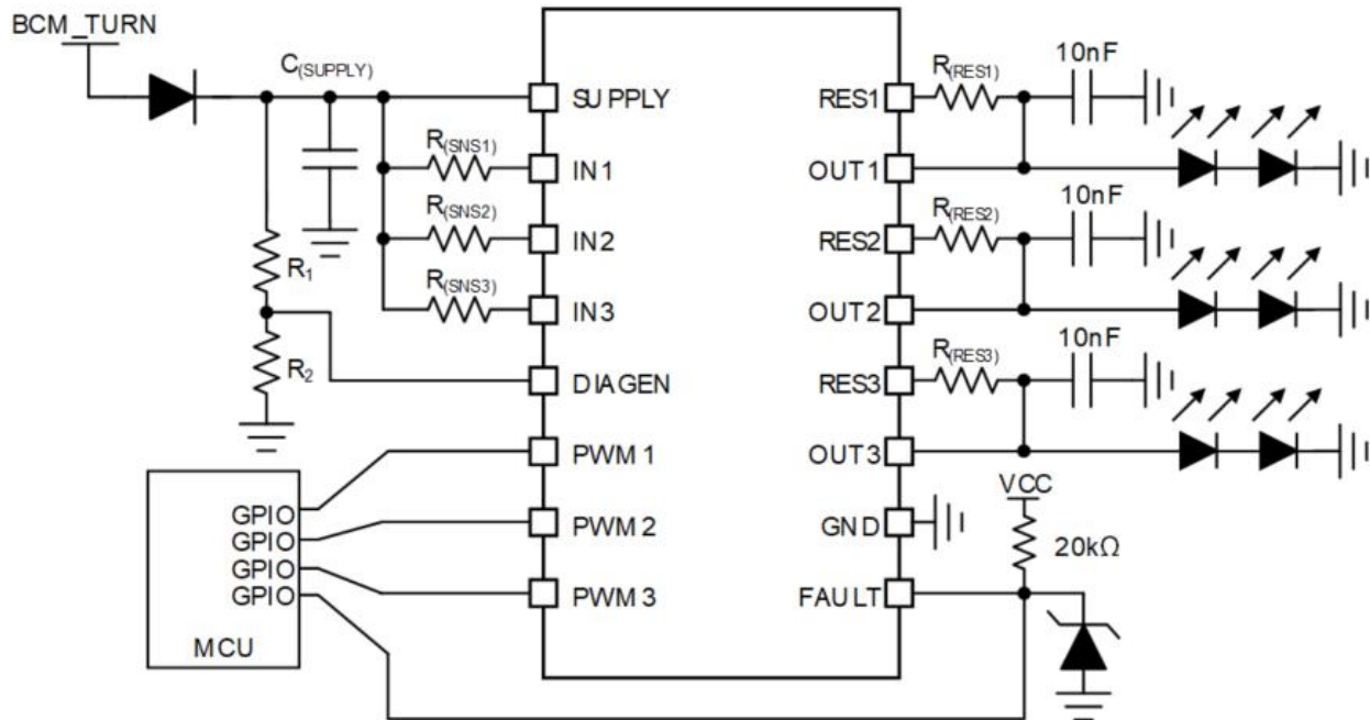
图 44. 典型应用示意图
