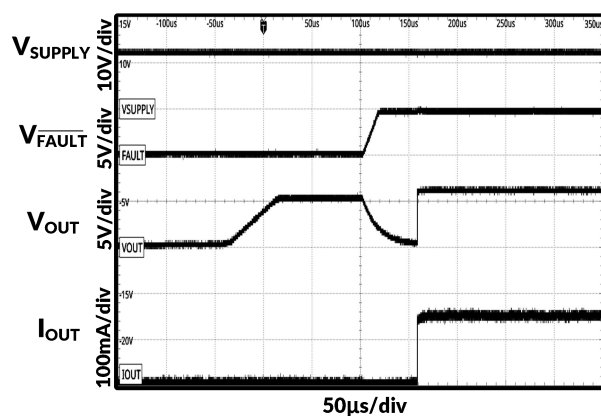
图 19. LED 短路保护恢复
