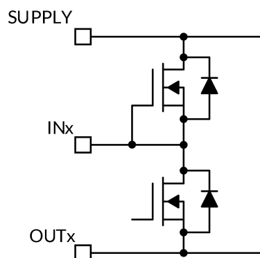
图 40. INx 引脚
