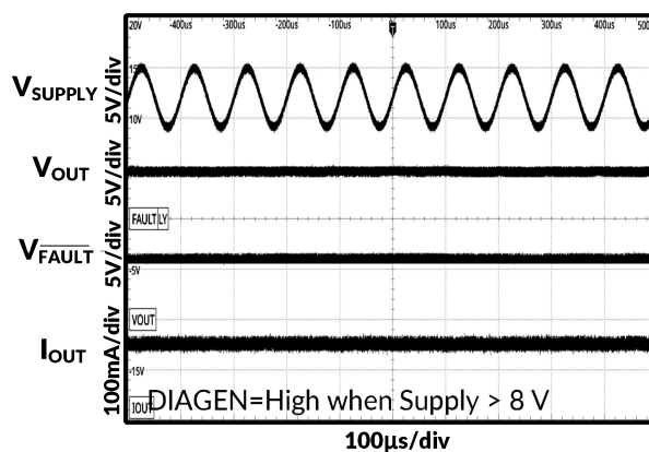
图 26. 10kHz 叠加交流电压
