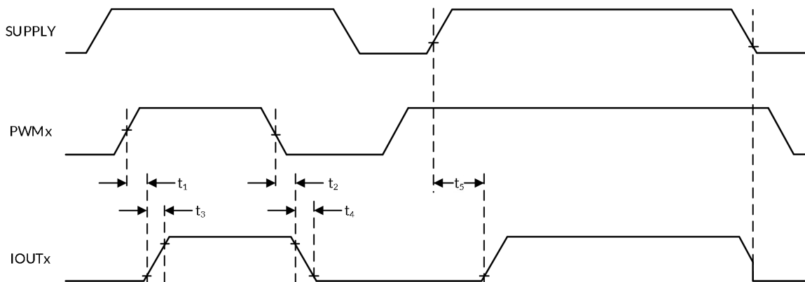
图 28. 上电顺序和 PWM 调光时序
