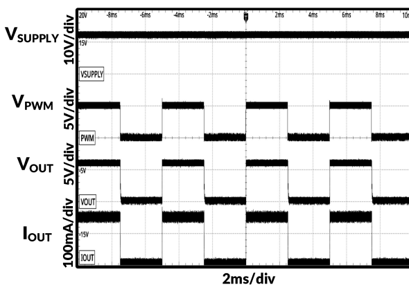
图 14. 200 Hz 时 PWM 调光
