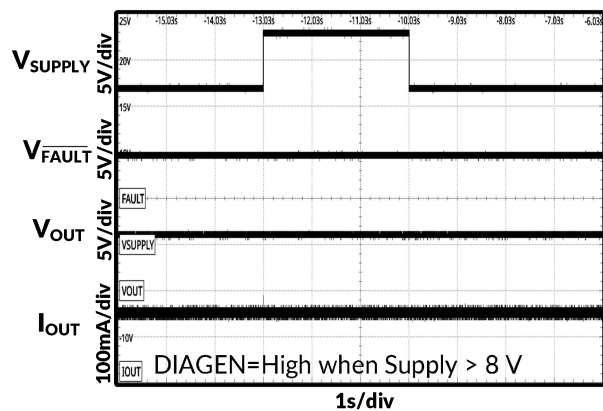
图 27. 跨接启动
