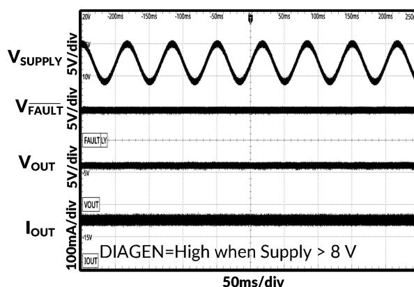
图 24. 15Hz 叠加交流电压
