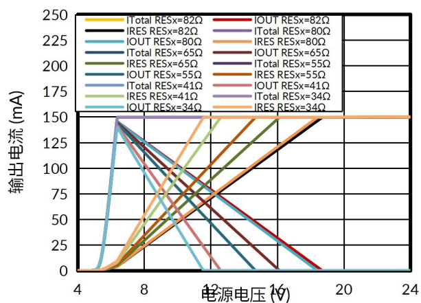
图 10. 输出电流分布与电源电压的关系
