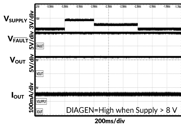
图 21. 瞬态过电压
