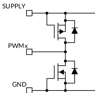
图 35. PWMx 引脚
