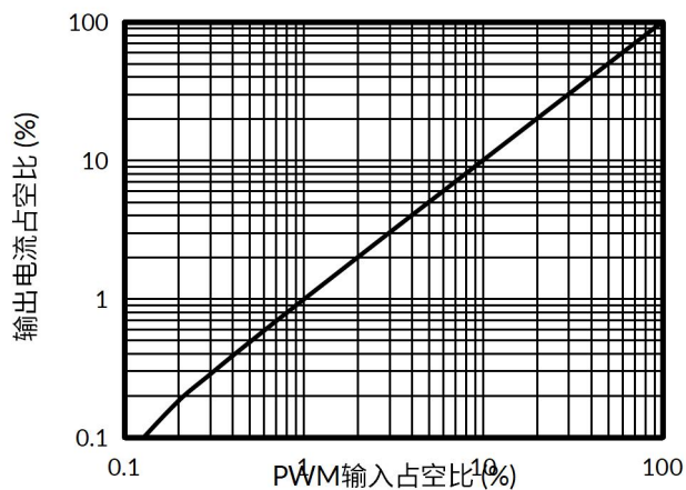
图 5. PWM 输出占空比与输入占空比的关系
