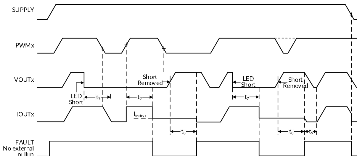
图 30. LED 接地短路检测和恢复时序图
