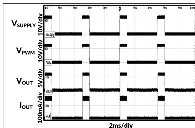
图 42. 200Hz 电源调光 20%亮度
