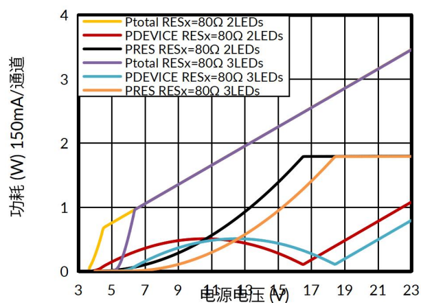
图 7. 功耗与电源电压的关系
