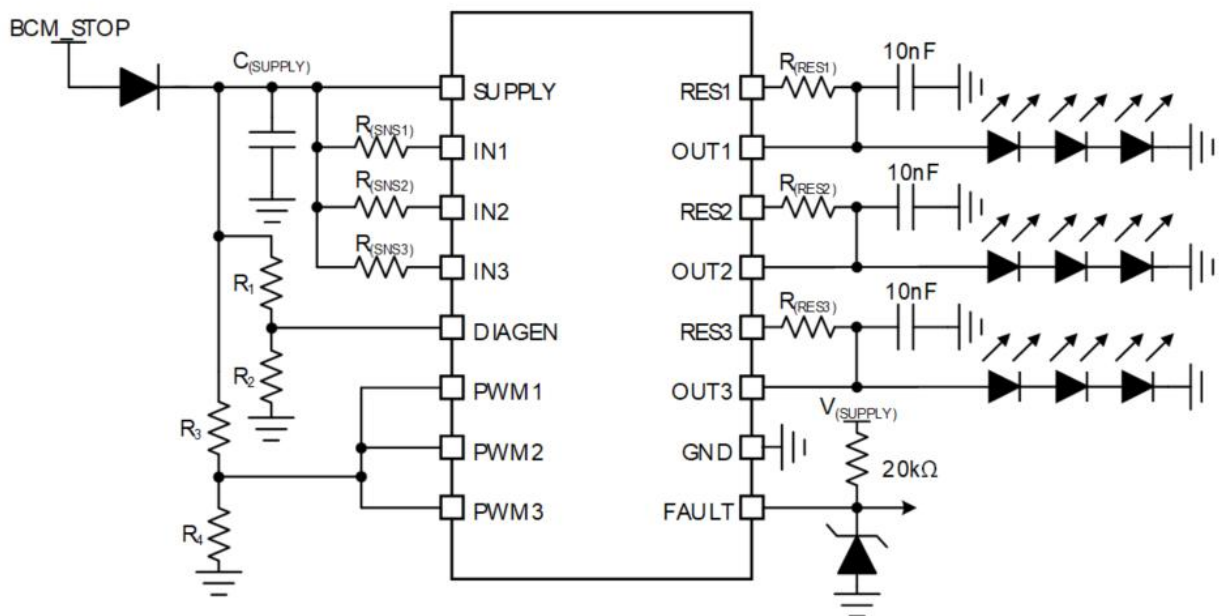
图 48. 典型应用示意图
