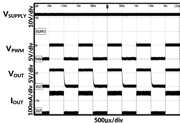
图 15. 1 kHz 时 PWM 调光
