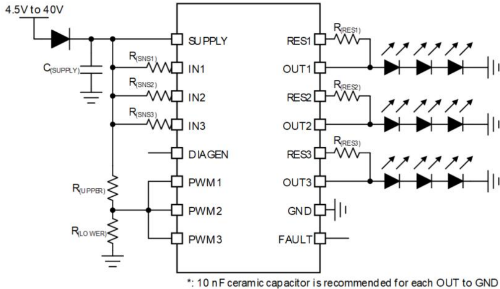
图 29. 电源控制 LED 亮度应用示意图
