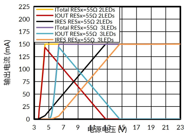
图 8. 输出电流分布与电源电压的关系
