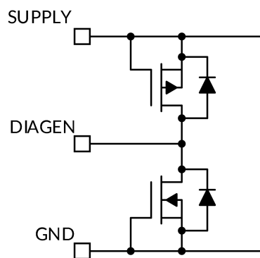
图 36. DIAGEN 引脚
