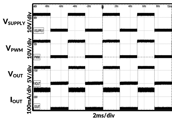
图 13. 200 Hz 时电源调光
