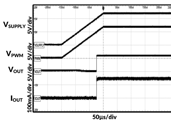
图 12. 上电顺序
