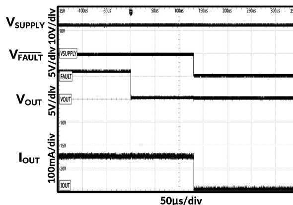
图 18. LED 短路保护
