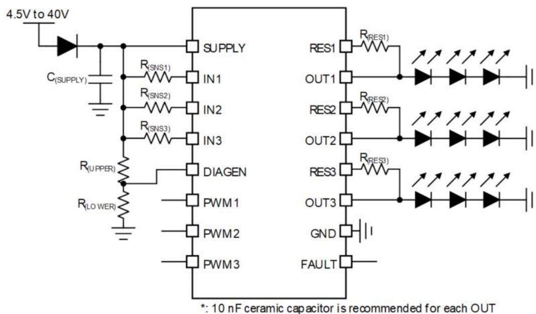
图 32. DIAGEN 应用示意图
