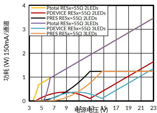
图 9. 功耗与电源电压的关系
