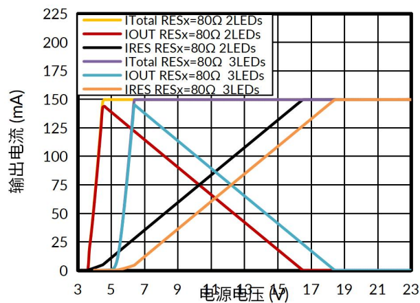
图 6. 输出电流分布与电源电压的关系
