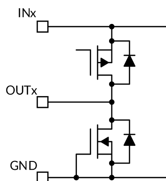
图 38. OUTx 引脚
