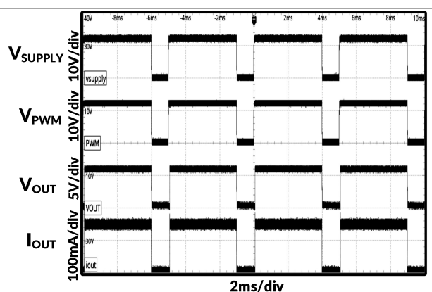
图 43. 200Hz 电源调光 80%亮度
