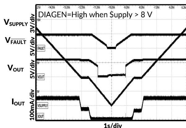
图 23. 电源电压缓慢下降和缓慢上升
