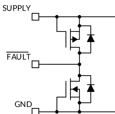
图 37. FAULT 引脚
