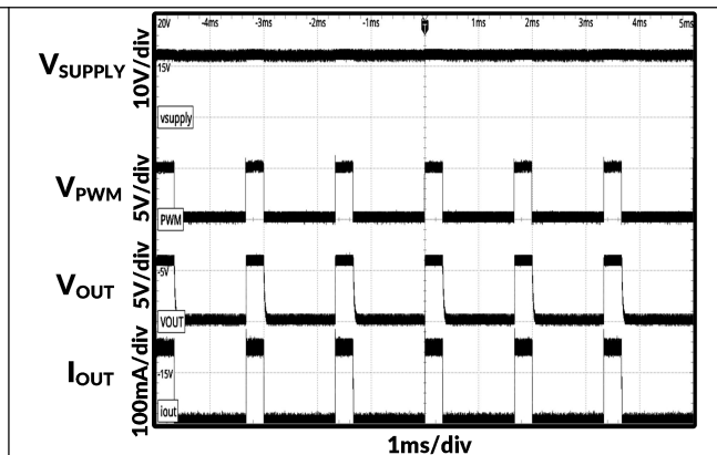
图 46. 20%占空比下的 600Hz PWM 调光
