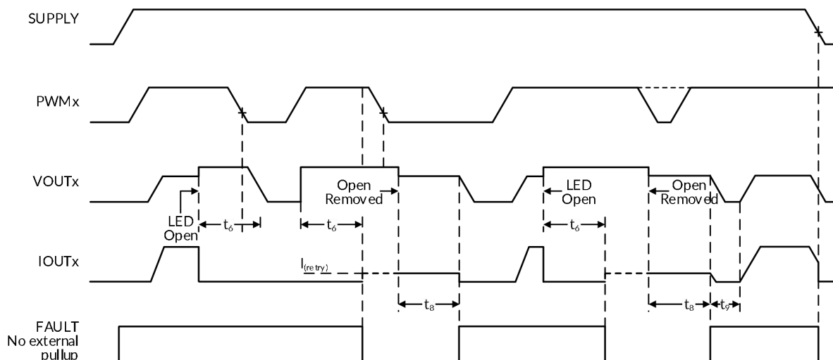
图 31. LED 开路检测和恢复时序图
