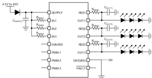
典型应用图
