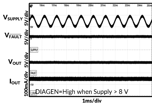
图 25. 1kHz 叠加交流电压
