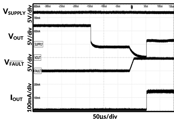
图 17. LED 开路保护恢复
