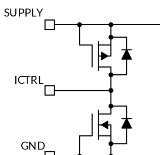
图 42. ICTRL 引脚
