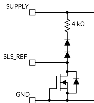
图 47. SLS_REF 引脚
