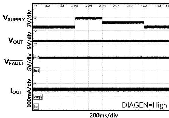
图 18. 瞬态过电压
