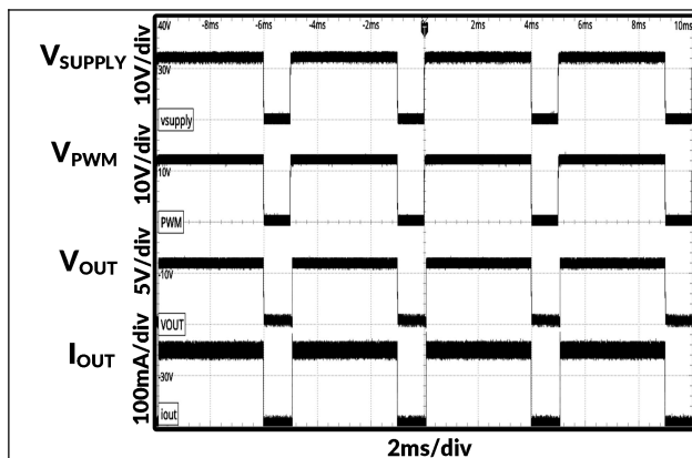
图 49. 电源调光 80% 的亮度
