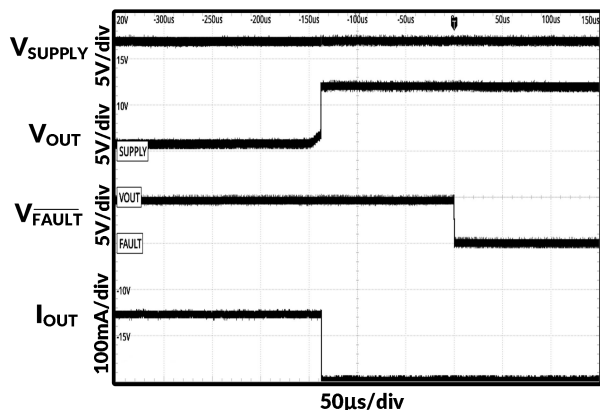
图 11. LED 开路保护
