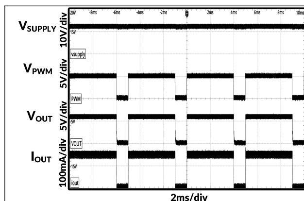
图 52. 200 Hz 时，PWM 调光占空比 80%
