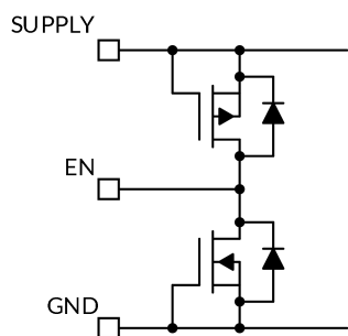
图 38. EN 引脚
