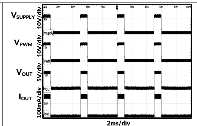
图 50. 电源调光 20% 的亮度
