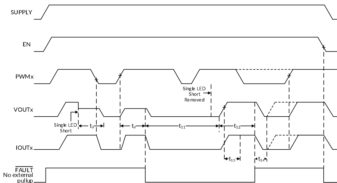
图 34. 单个 LED 短路检测和恢复时序图
