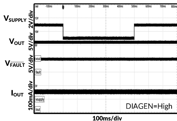
图 17. 瞬态欠电压
