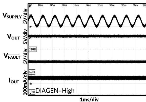
图 22. 1kHz 叠加交流电压
