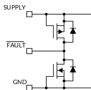
图 41. FAULT 引脚
