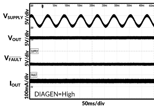
图 21. 15Hz 叠加交流电压
