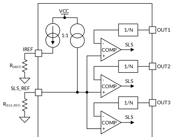
图 33. 单个 LED 短路检测框图
