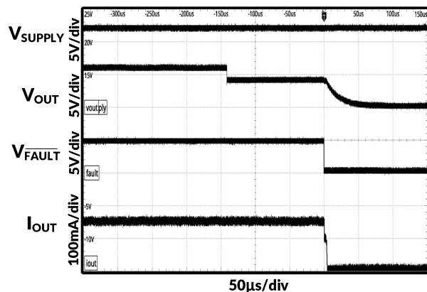
图 15. 单个 LED 短路保护
