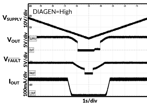
图 20. 电源电压缓慢下降和缓慢上升
