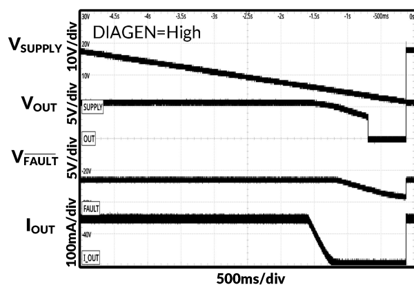
图 19. 电源电压缓慢下降和快速上升
