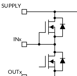
图 45. IN1, IN2 和 IN3 引脚
