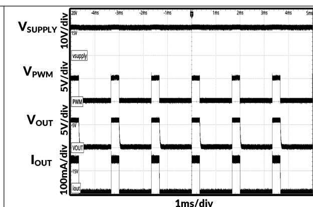
图 53. 600 Hz 时，PWM 调光占空比 20%
