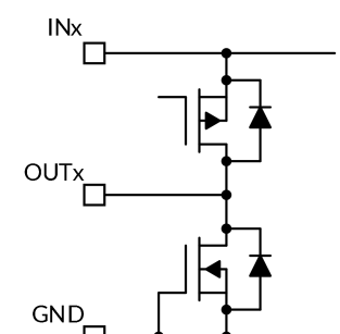
图 43. OUT1, OUT2 和 OUT3 引脚
