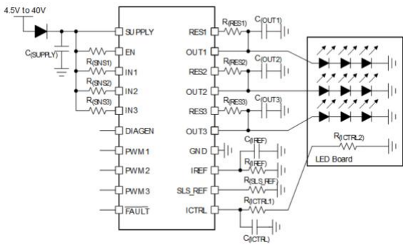
典型应用图
