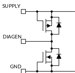
图 40. DIAGEN 引脚
