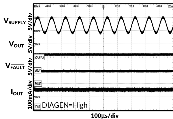
图 23. 10kHz 叠加交流电压
