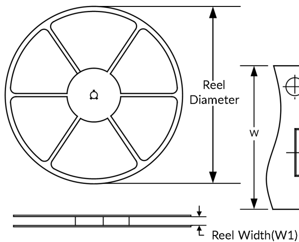
REEL DIMENSIONS
