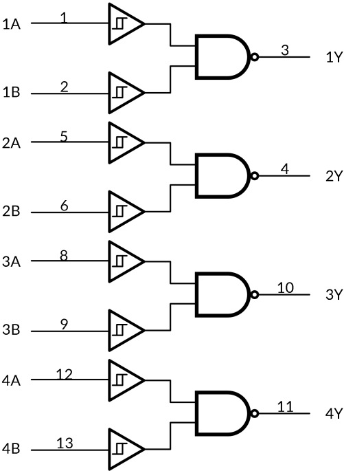
功能框图
