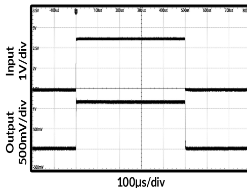
图 7. 脉冲响应
