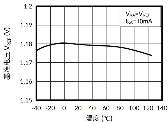
图 8. 基准电压与环境温度的关系
