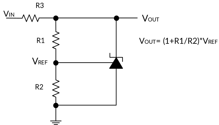
图 1. 并联稳压器
