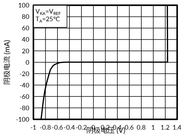
图 4. 阴极电流与阴极电压的关系
