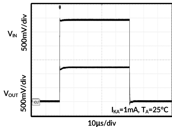
图 10. 脉冲响应
