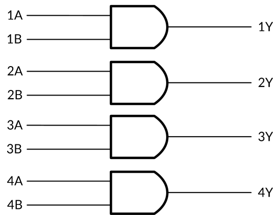
逻辑符号
