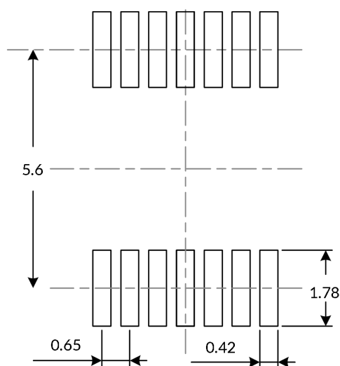
推荐焊盘尺寸 (单位: 毫米)
