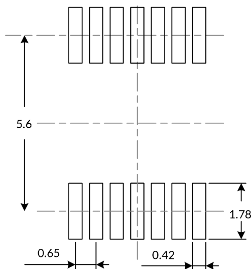
推荐焊盘尺寸 (单位: 毫米)
