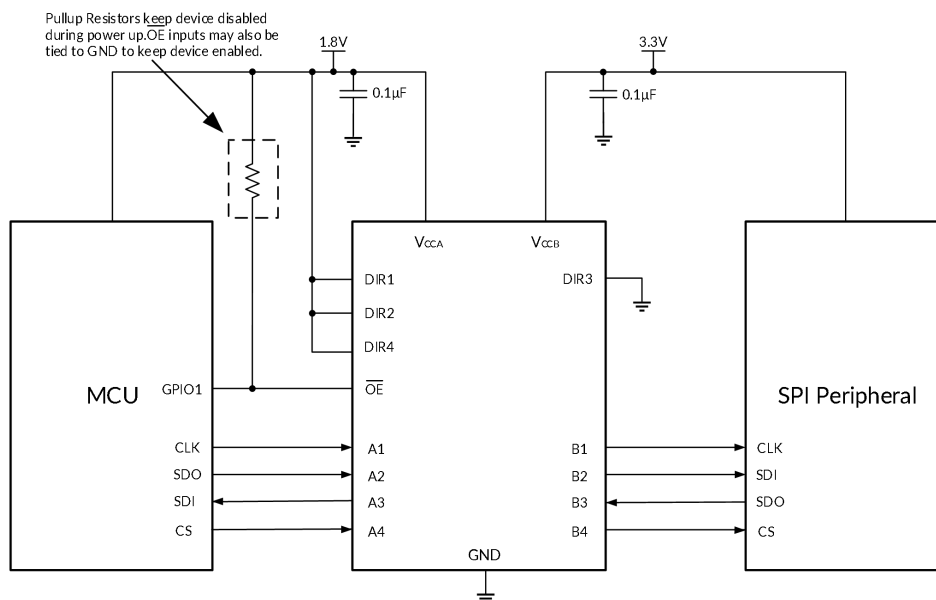
图 2. 典型应用电路
