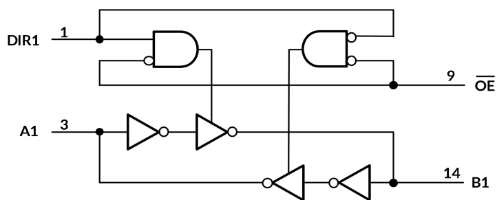
逻辑图（正逻辑）
