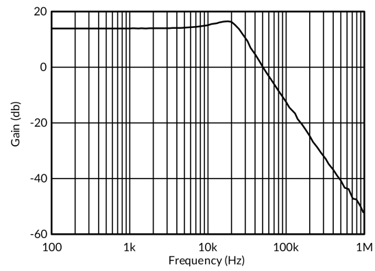
图 19. 低通滤波器
