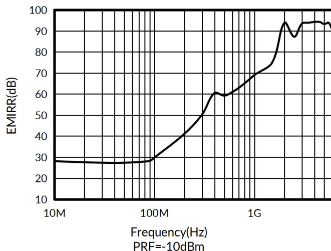
图 16. TLX52X EMIRR和频率的关系
