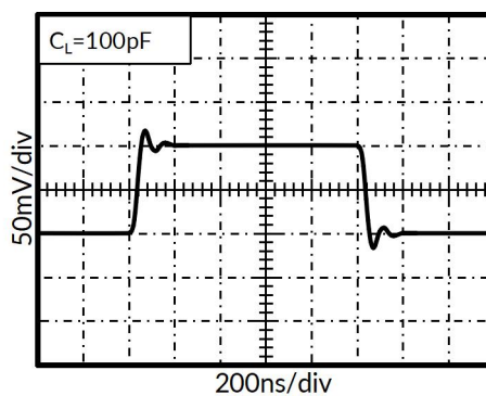
图 10. 小信号阶跃响应
