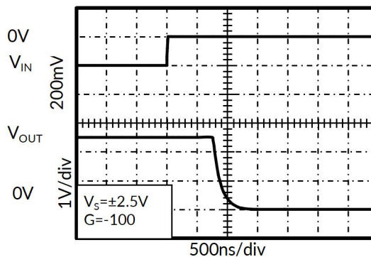
图 12. 正向过压恢复
