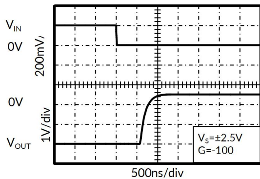
图 13. 反向过压恢复
