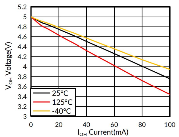
图 2. 电压与电流
