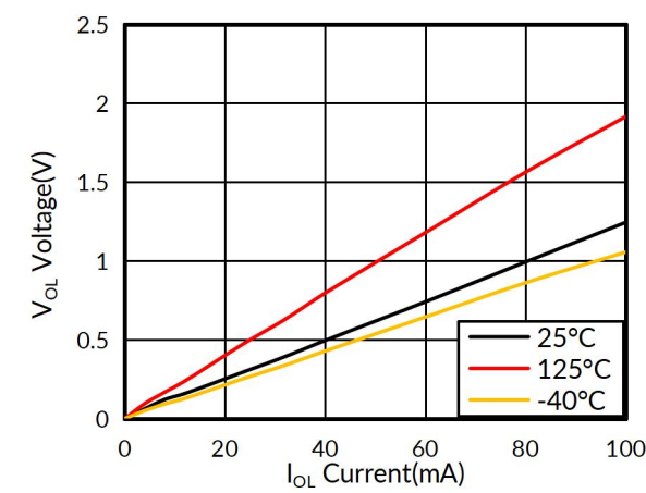
图 1. 电压与电流
