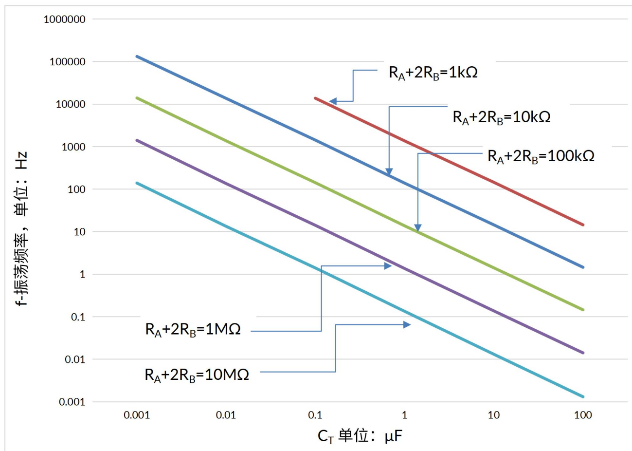
图 9 自由频率与电容电阻间的关系
