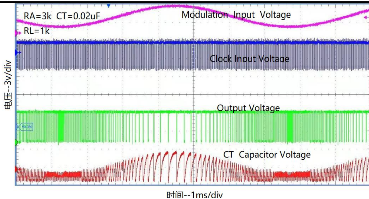
图 12 脉宽调制波形
