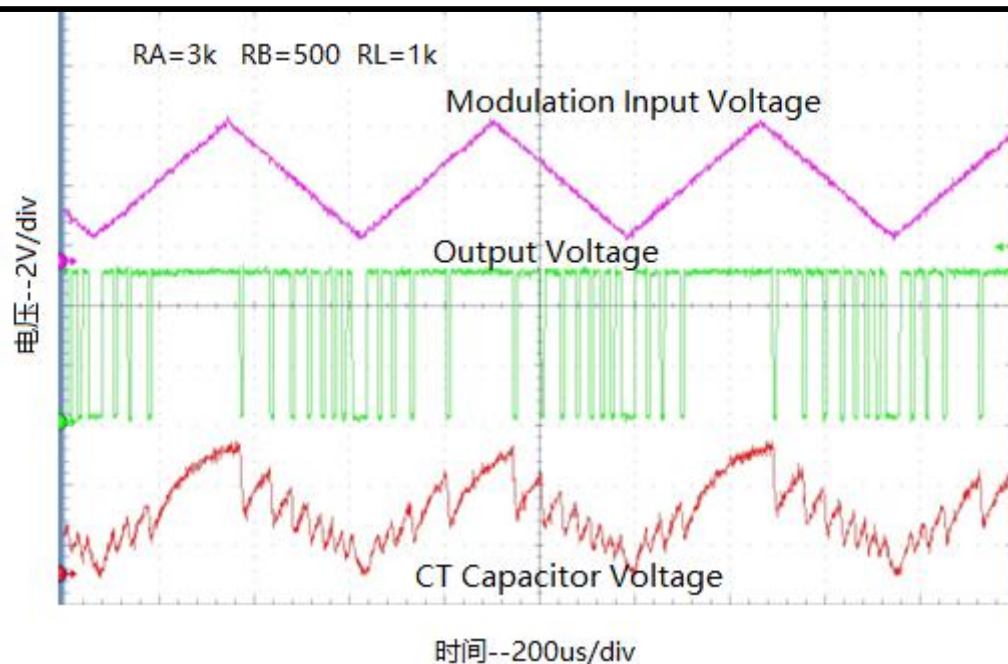
图 14 脉冲位置调制波形
