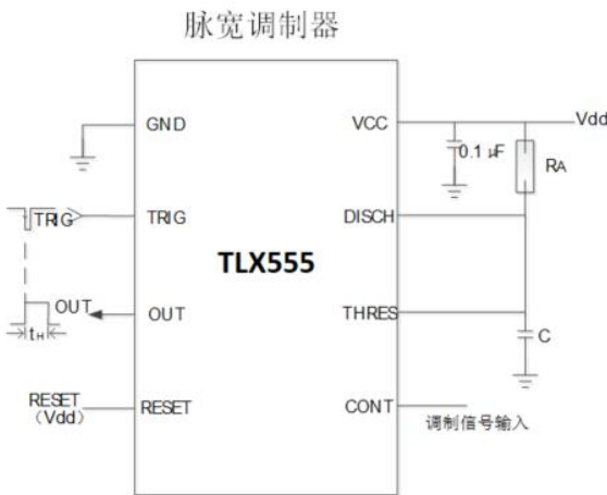
图1 TLX555 典型应用场合
