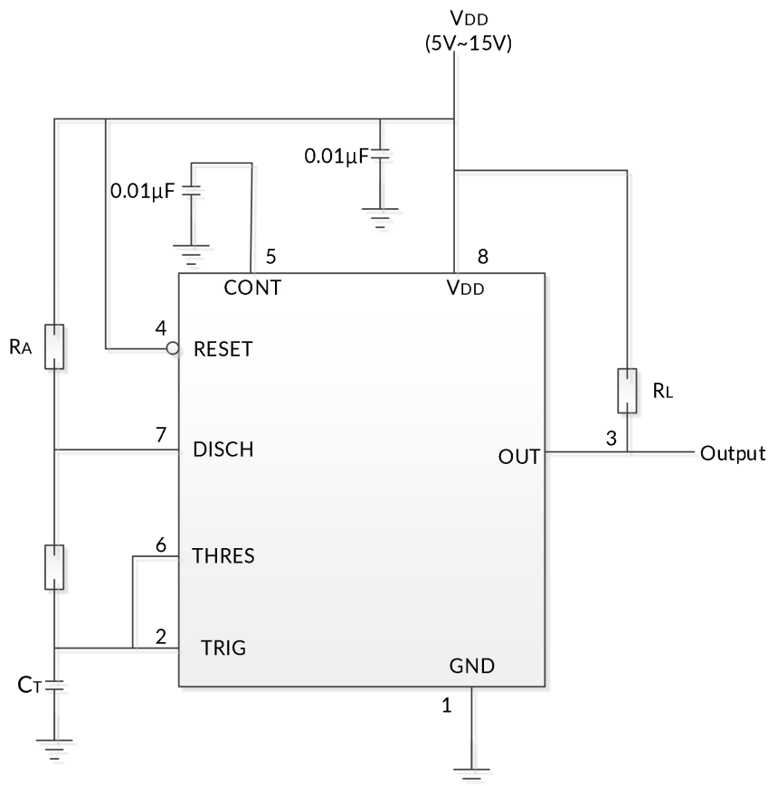
图 7 A 稳态工作电路
