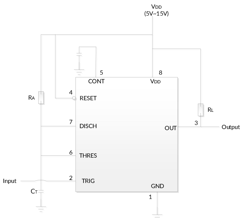
图 4 单稳态工作模式
