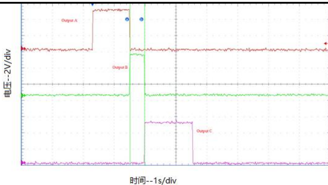
图 16 顺序计时器波形
