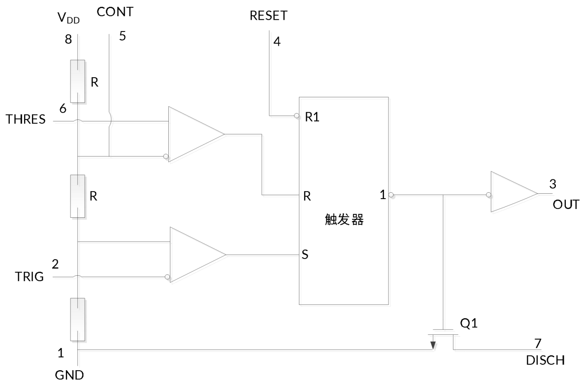
图 3 TLX555 芯片示意图
