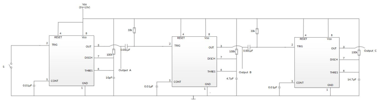
图 15 顺序计时器电路
