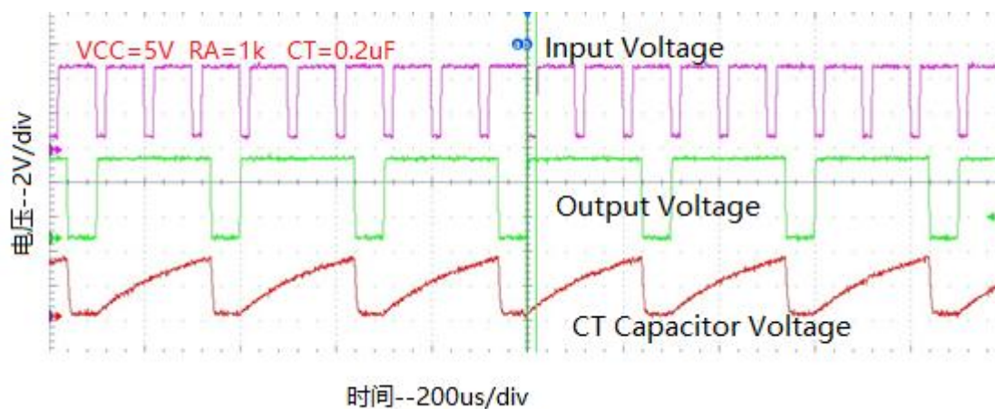
图 10 三分频电路波形
