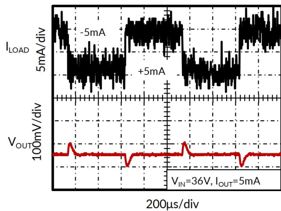
图 13. 负载瞬变
