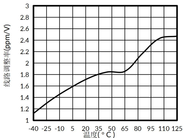
图 5. 线路调节率与温度的关系
