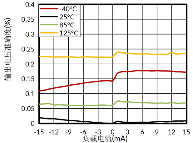
图 2. 输出电压与负载电流
