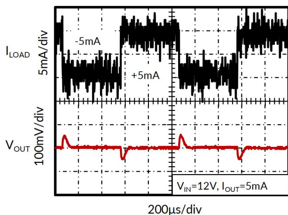
图 11. 负载瞬变
