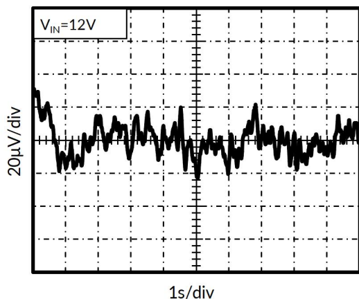
图 7. 0.1Hz 至 10Hz 噪声
