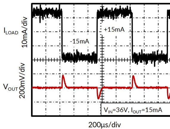
图 14. 负载瞬变
