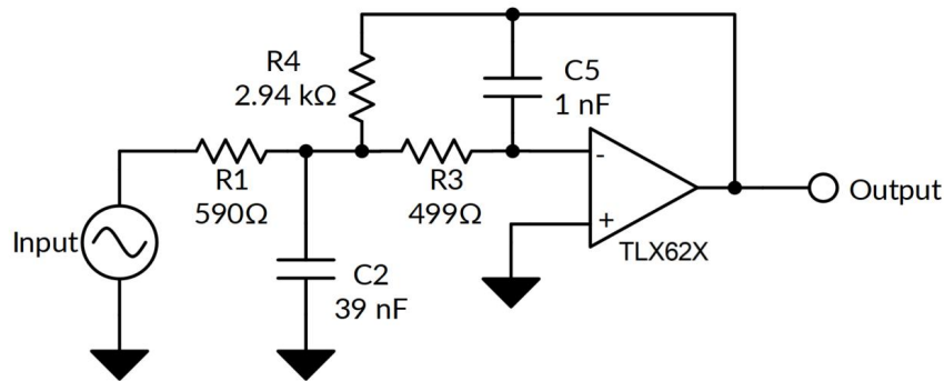
图 18. 25-kHz 低通滤波器
