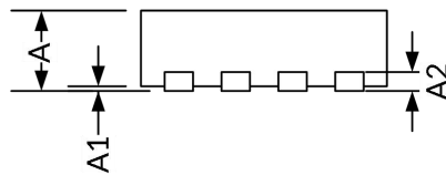
侧视图
