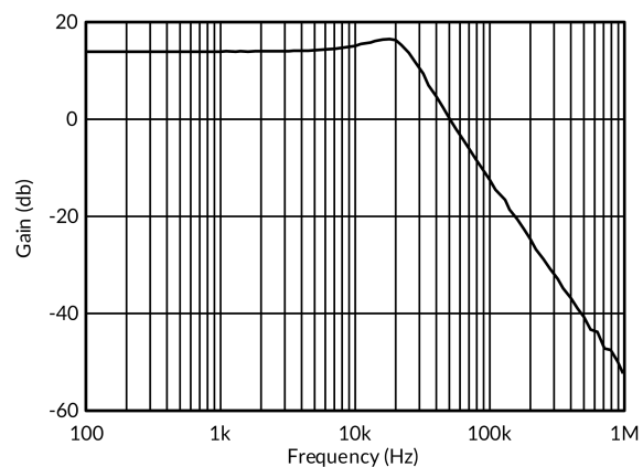
图 19. 低通滤波器
