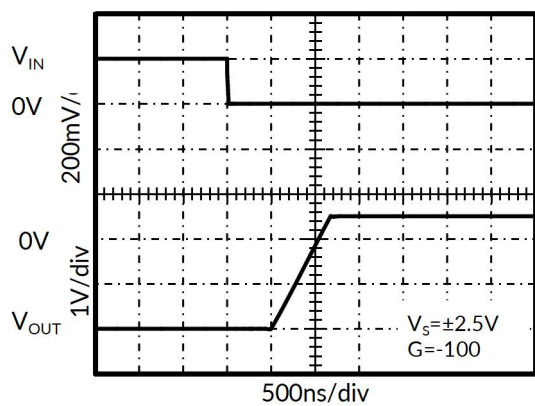
图 13. 反向过载恢复
