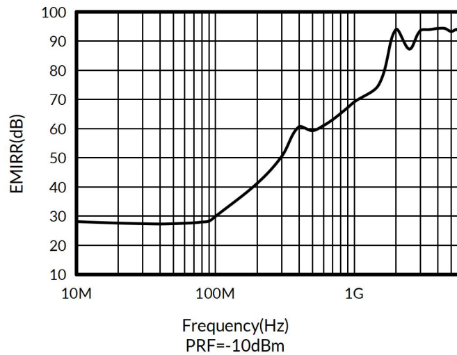
图 16. TLX62X EMIRR和频率的关系
