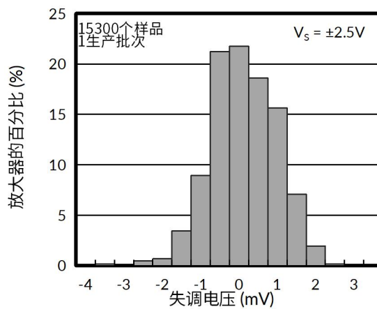
图 14. 失调电压分布
