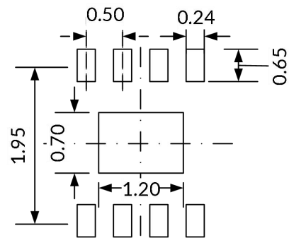
底视图
