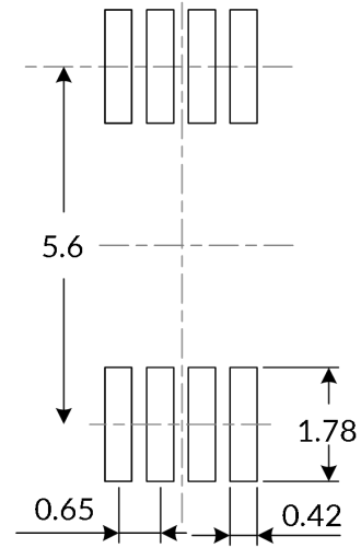
推荐焊盘尺寸 (单位: 毫米)
