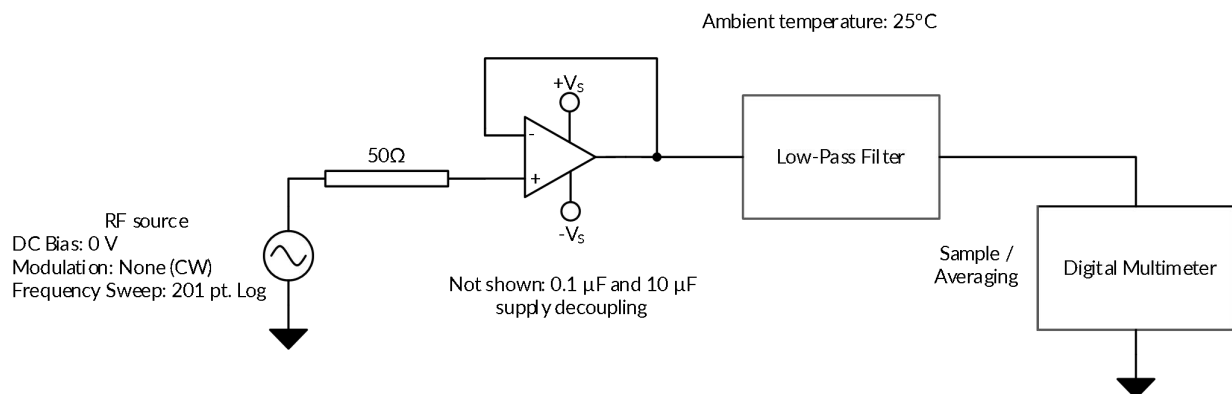
图 17. EMIRR IN+ 测试配置示意图
