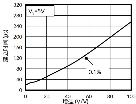
图 5. 建立时间与增益的关系
