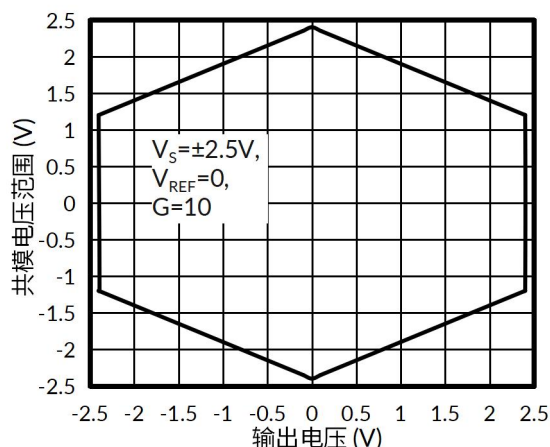
图 12. 典型共模范围与输出电压的关系
