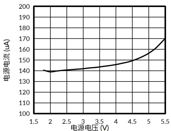
图 11. 电源电流与电源电压的关系
