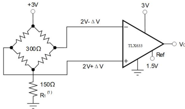
图 16. 单电源桥式放大器
