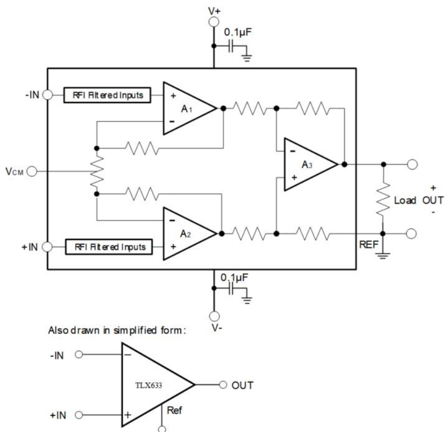
图 13. 基本连接
