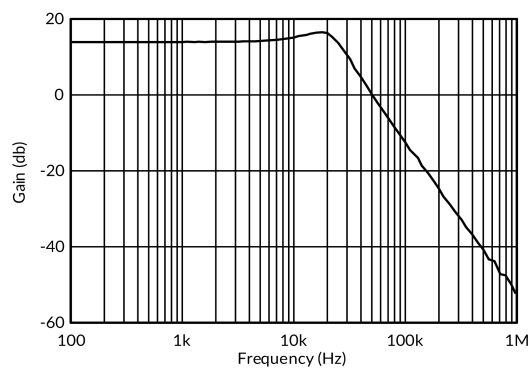
图 18. 低通滤波器
