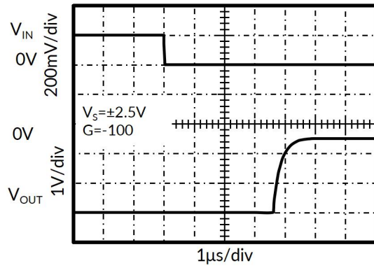
图 13. 反向过载恢复
