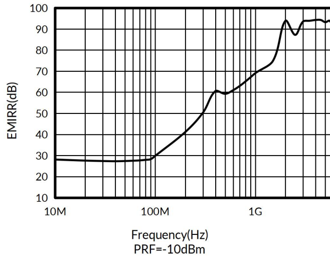
图 15.TLX633XP EMIRR和频率的关系
