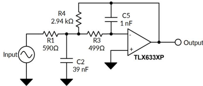
图 17. 25-kHz 低通滤波器
