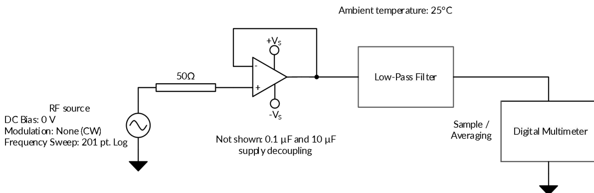
图 16. EMIRR IN+ 测试配置示意图
