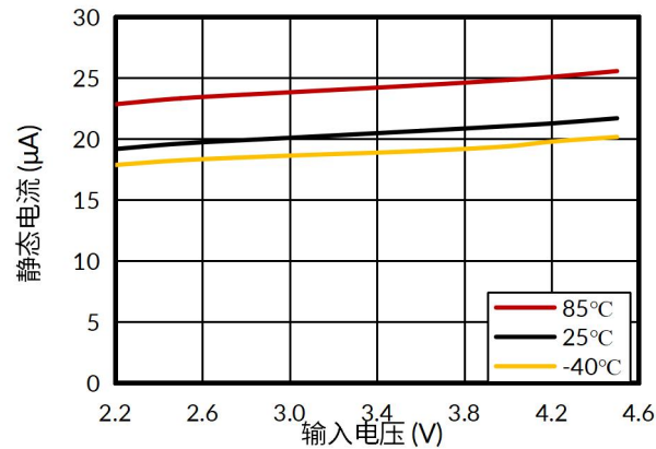
图 4. 静态电流与输入电压曲线
