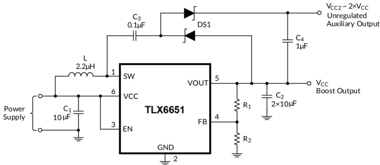
图 14. 辅助正输出电源
