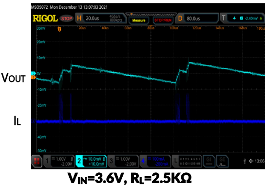
图 11. 省电模式下的输出电压
