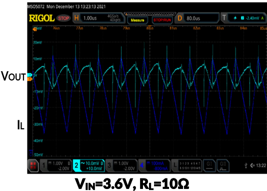
图 12. 连续模式下的输出电压
