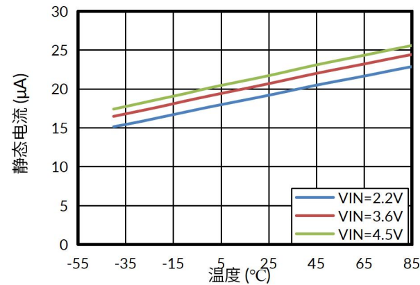
图 3. 静态电流与温度曲线
