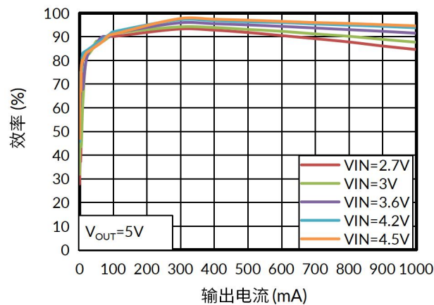
图 5. 输出电流与效率曲线
