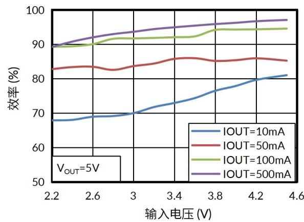
图 6. 输入电压与效率曲线
