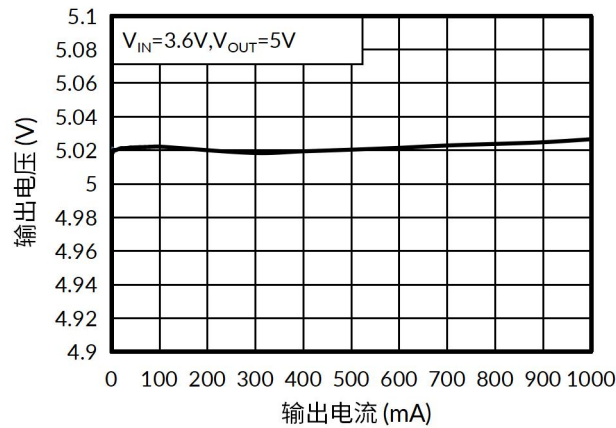
图 1. 输出电压与输出电流曲线
