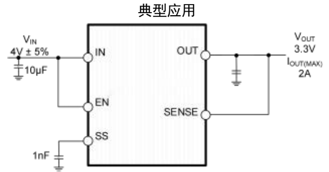
图 1 典型应用
