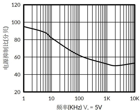
图 4. 电源抑制比与频率
