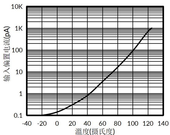
图 9. 输入偏置电流与温度
