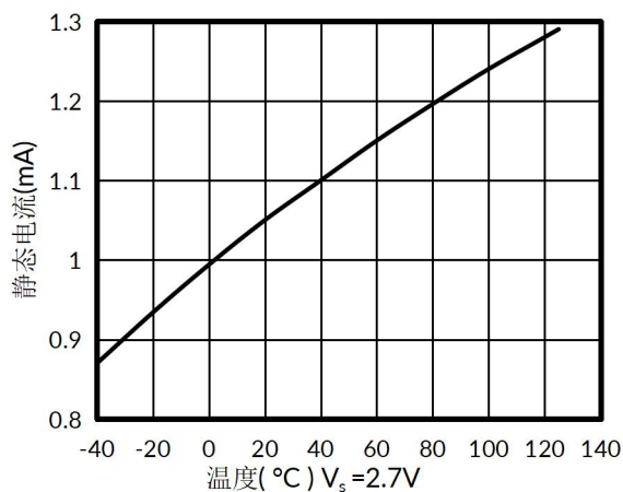
图 6. 静态电流与温度
