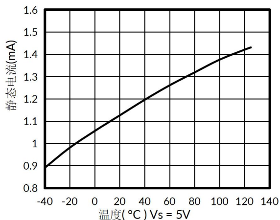
图 5. 静态电流与温度
