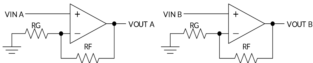
图 20. 示意图
