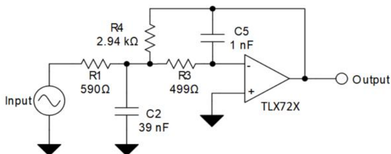
图 18. 25 kHz 低通滤波器
