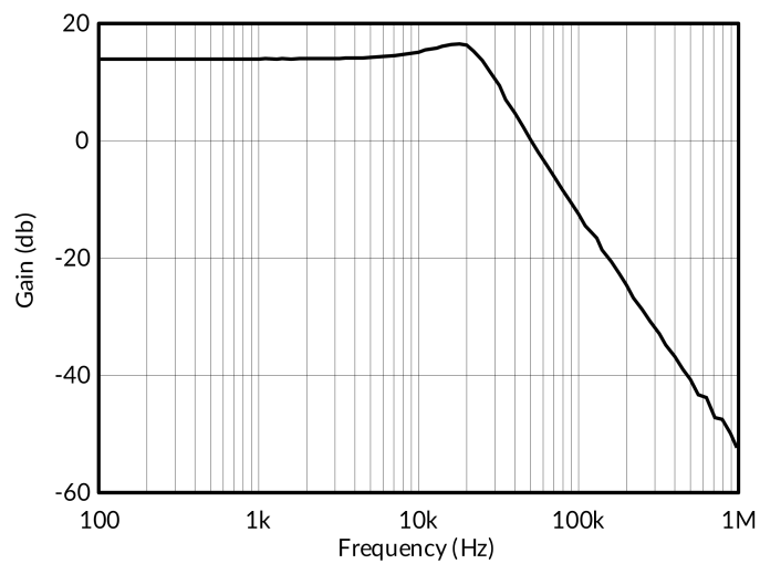
图 19. 低通滤波器传递函数
