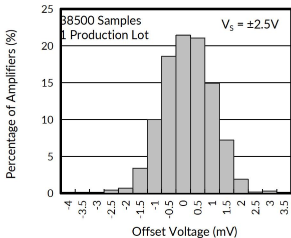
图 14. 失调电压产生分布
