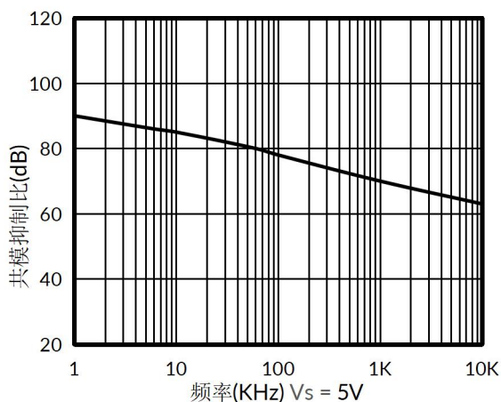
图 2. 共模抑制比与频率
