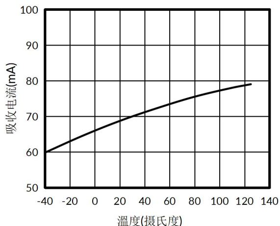
图 7. 吸收电流与温度
