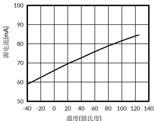
图 8. 源电流与温度
