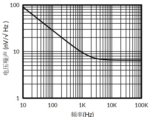
图 3. 输入电压噪声 频谱密度与频率
