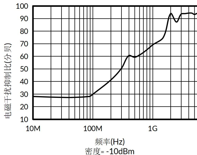
图 16. TLX72X EMIRR 与频率
