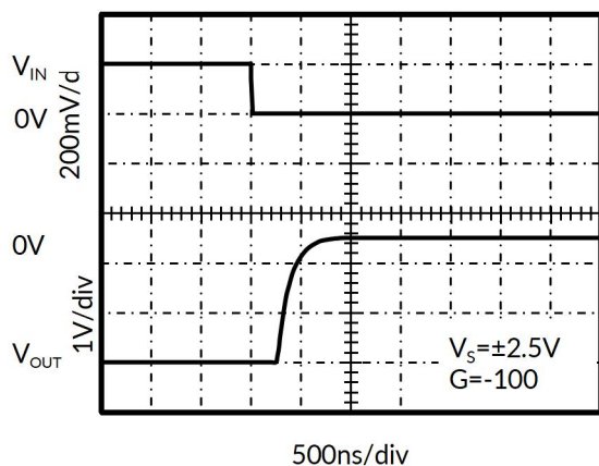
图 13. 负过载恢复
