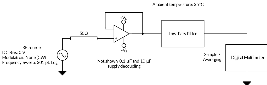
图 24. EMIRR IN+ 测试配置原理图
