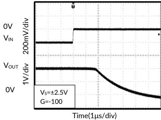
图 13. 正过压恢复
