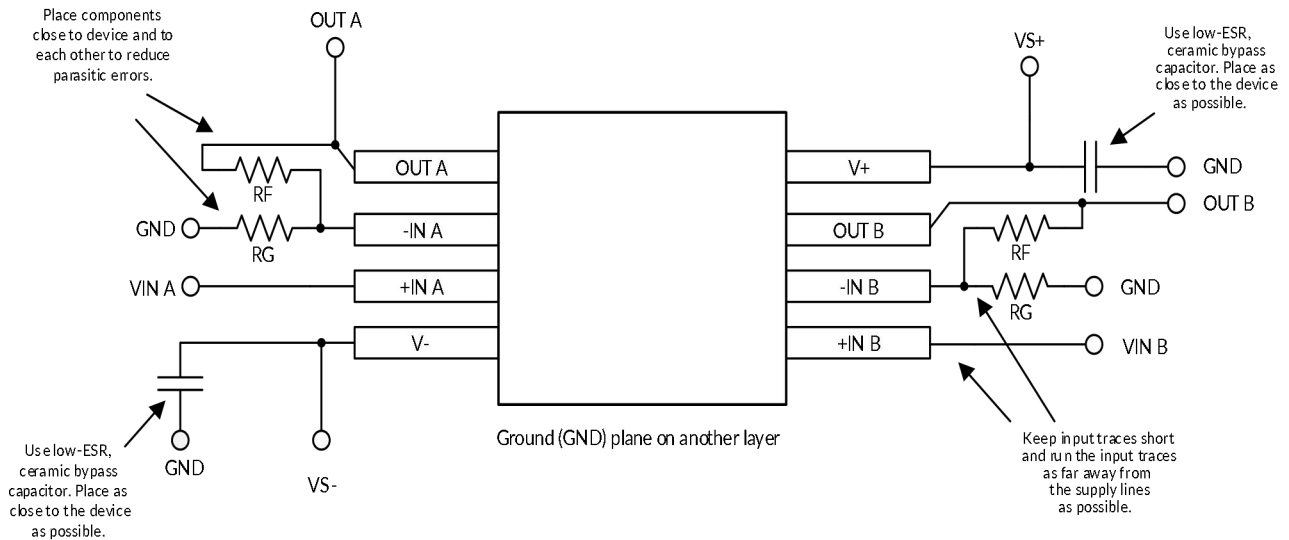
图 28. 布局示例
