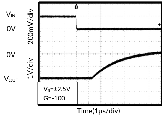
图 14. 负过压恢复
