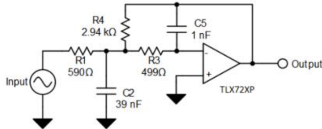
图 25. 25 kHz 低通滤波器
