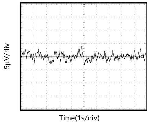
图 12. 0.1Hz 至 10Hz 输入电压噪声
