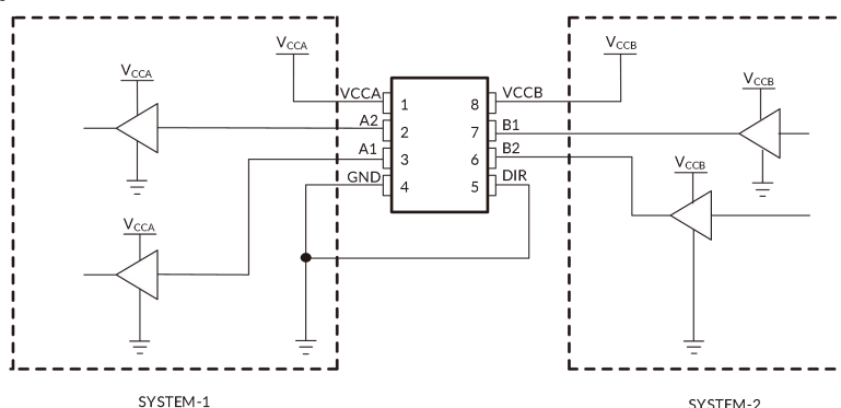
图 4. 单向逻辑电平转换应用
