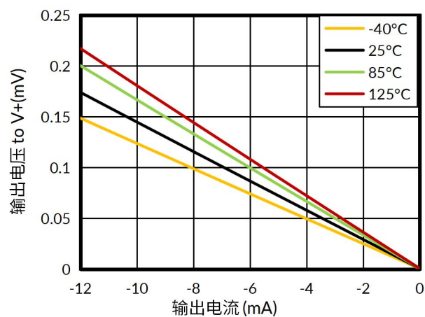
图 2. 输出高电压与输出电流的关系，3V
