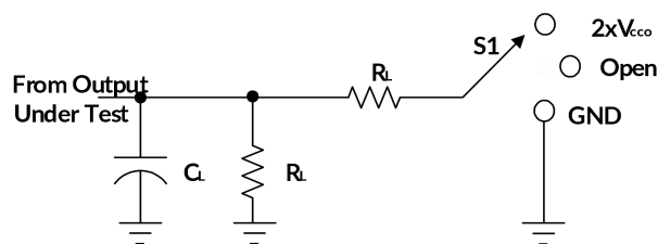
负载电路
