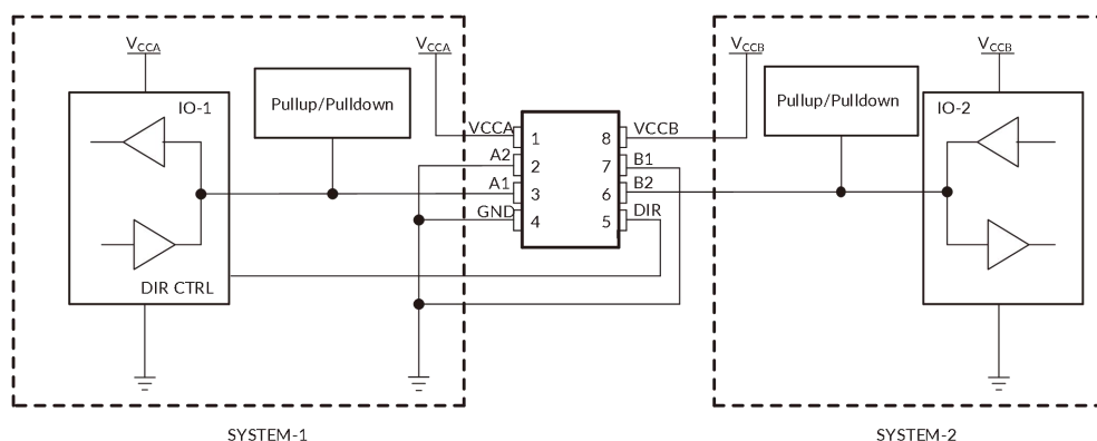
图 5. 双向逻辑电平转换应用
