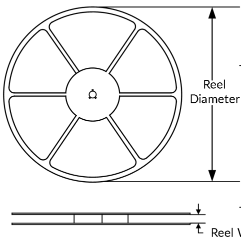
卷盘尺寸
