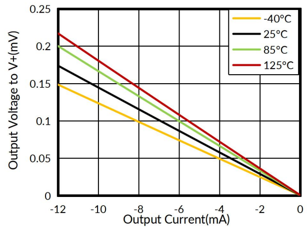
图 2. 输出电压高与输出电流，3V
