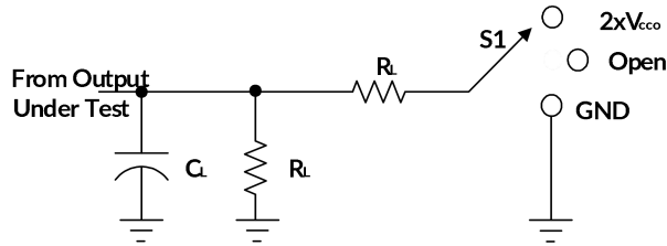
负载电路
