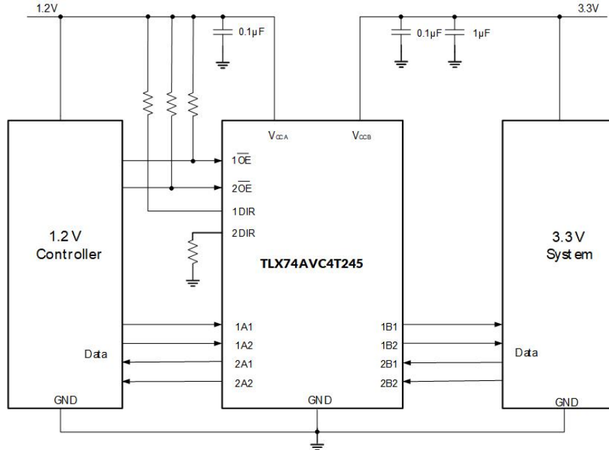
图 4.典型应用图
