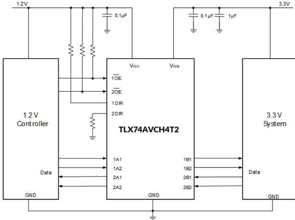
图 4.典型应用图
