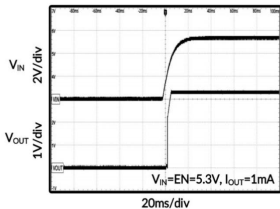
图 21. 上电时序
