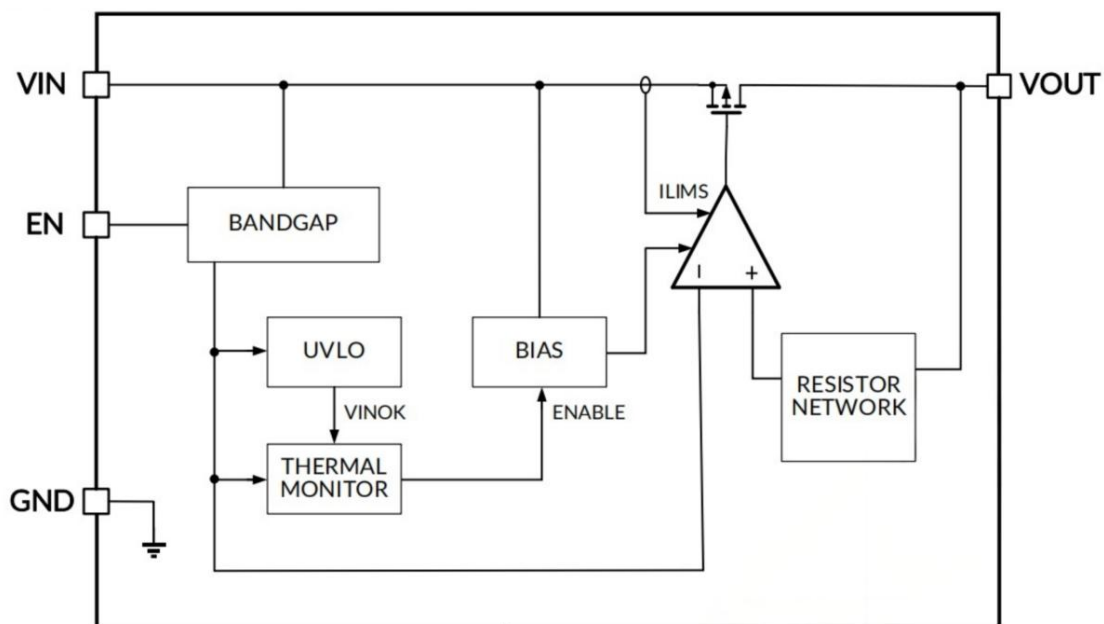
图 1. 固定电压版本
