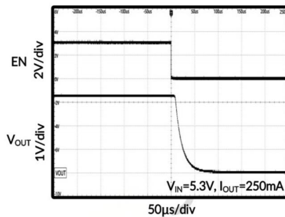
图 28. 关断时序
