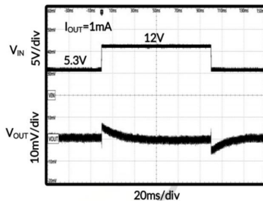
图 34. 线性瞬态响应
