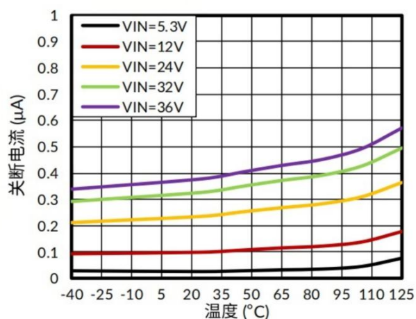
图6. 关断电流与温度的关系
