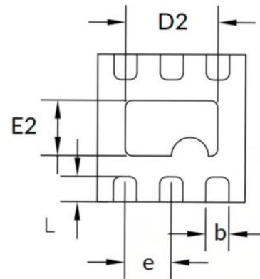
底视图
