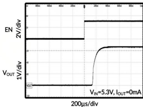
图 25. 开启时序
