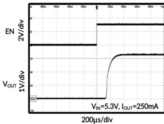
图 27. 开启时序
