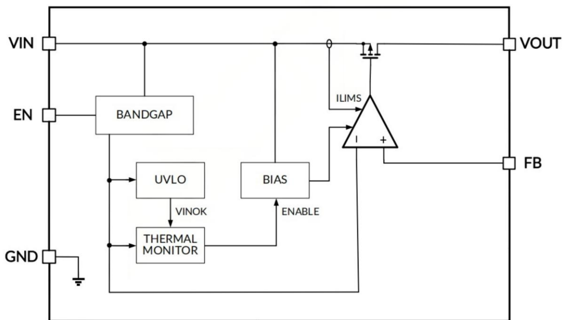
图2.可调电压版本
