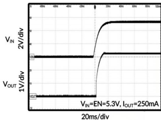
图 23. 上电时序
