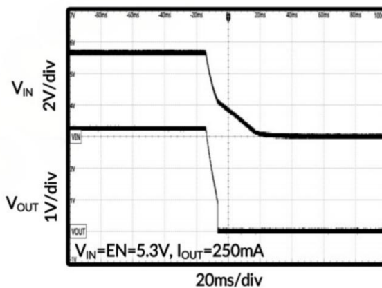
图 24. 下电时序
