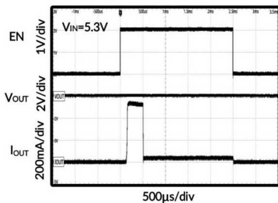
图 31. 先短路后使能时序图
