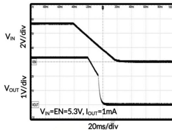
图 22. 下电时序
