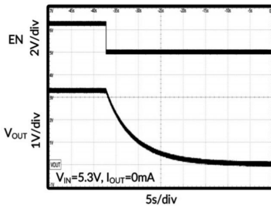
图 26. 关断时序
