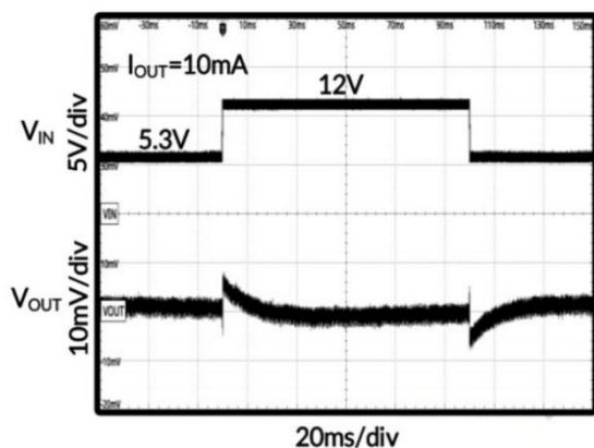
图 35. 线性瞬态响应
