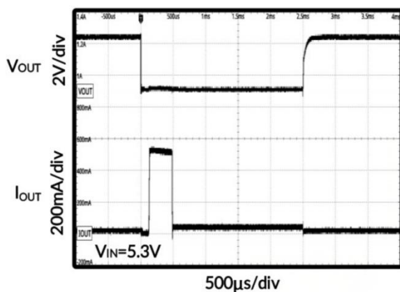
图 29. 先开机后短路时序图
