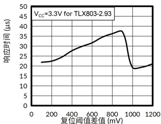
图 3. 响应时间与复位阈值差值的关系
